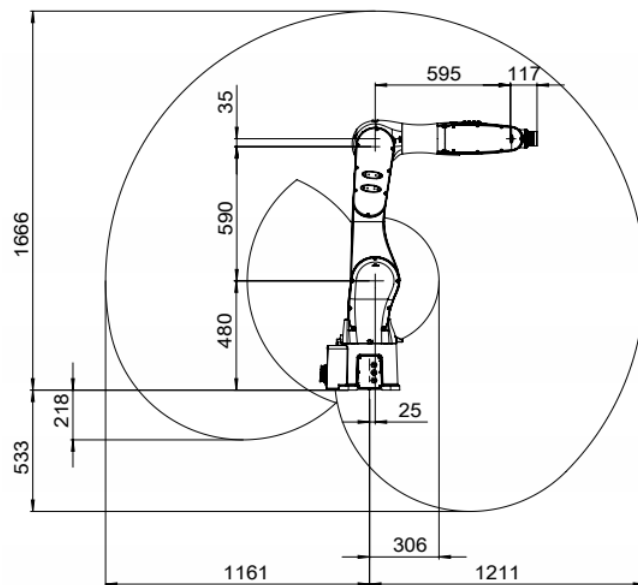
(a)侧视图
