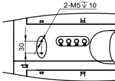
(b) 顶部安装孔
