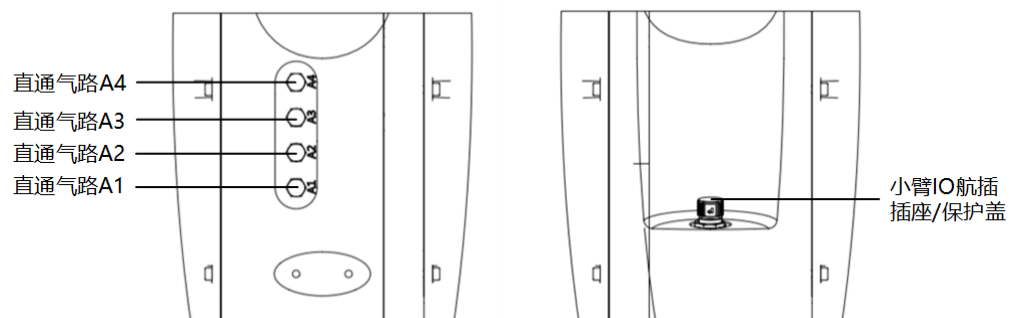
图 5-2 AIR10-1210C 操作机小臂上接口
