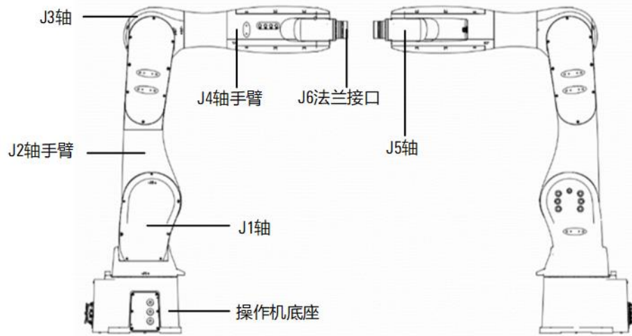
图 1-3 机器人本体及其各个部分
