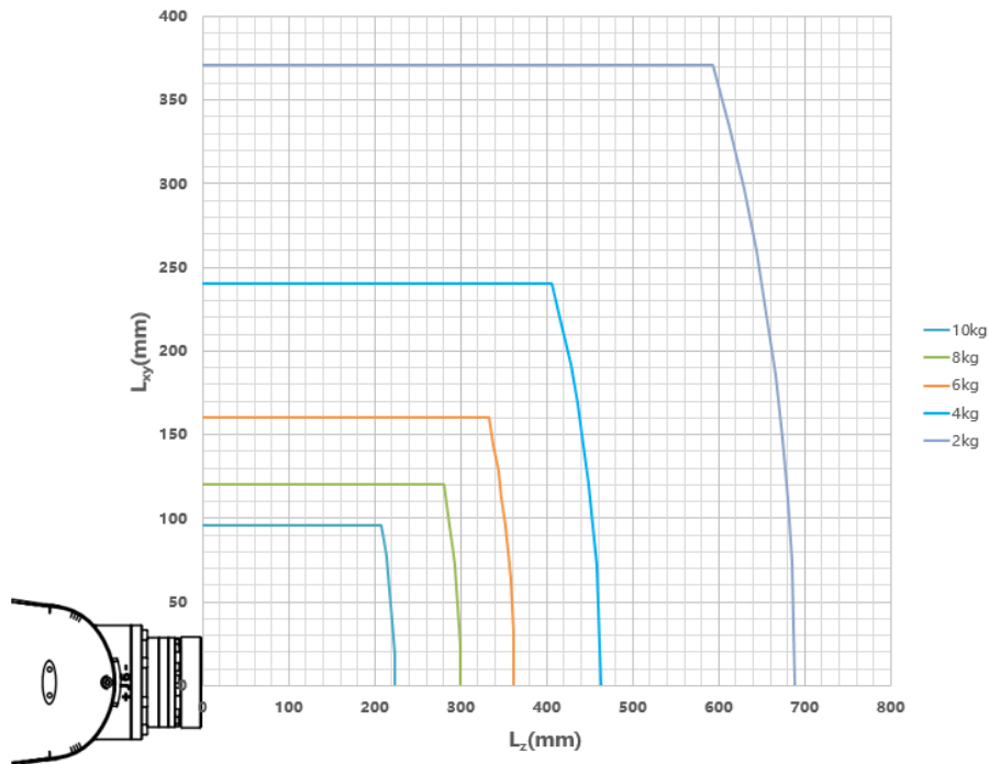
(b) AIR10-1210C-HW 负载质心位置允许范围示意图
