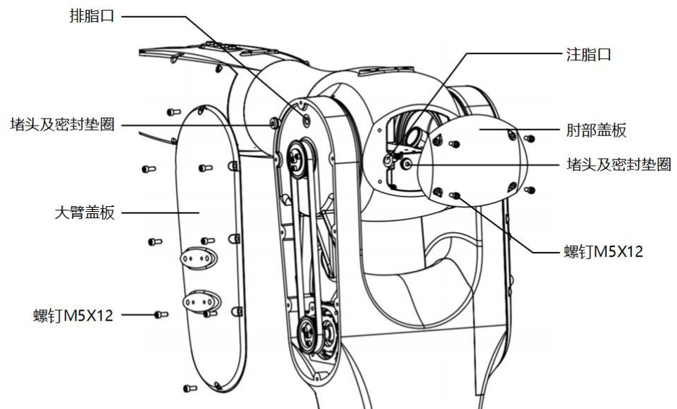
图 12-6 更换 J3 轴减速器润滑脂
