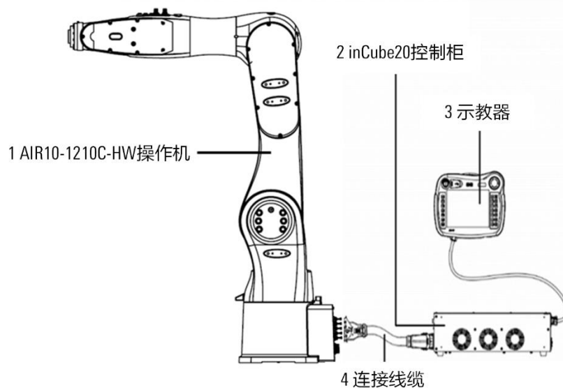
图 1-2 AIR10-1210C-HW 工业机器人系统的构成
