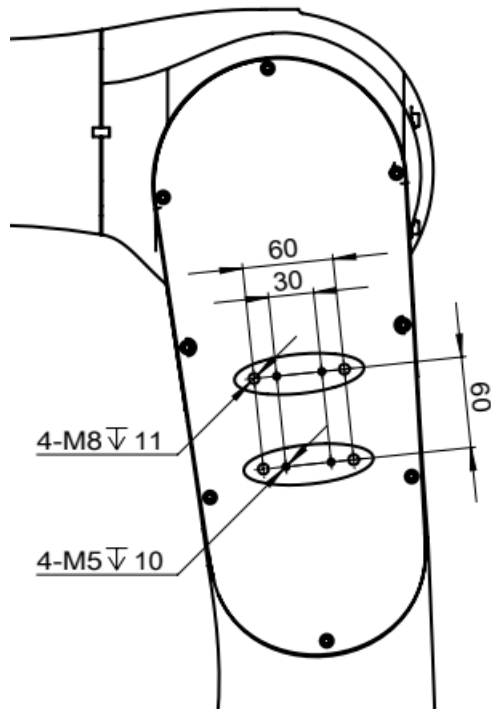
图 7-12 操作机大臂接口尺寸图
