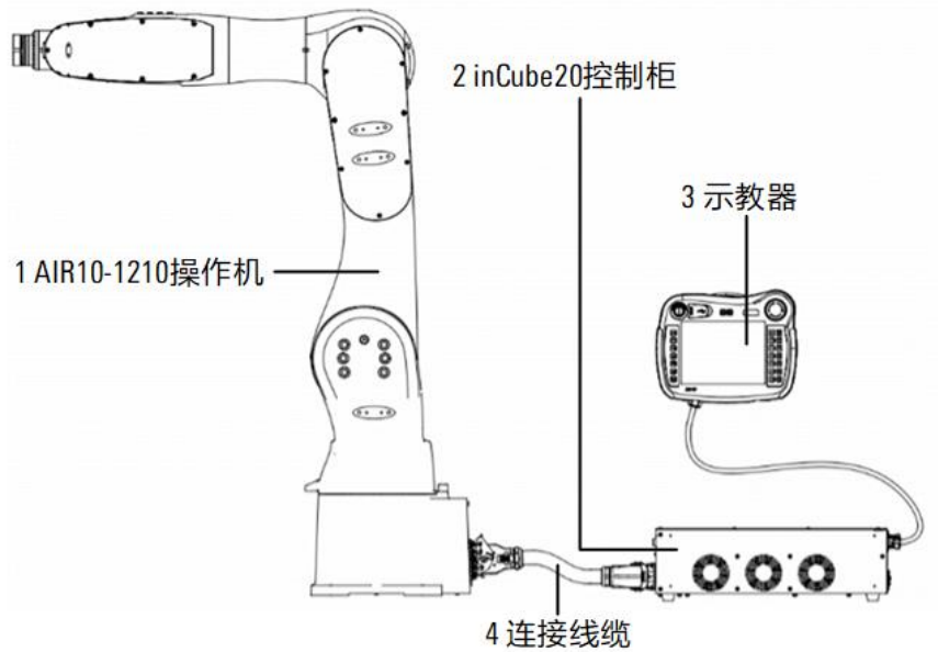
图 1-1 AIR10-1210C 工业机器人系统的构成
