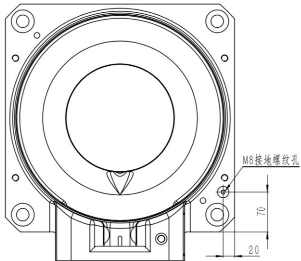
图 6-6 操作机底座接地示意图
