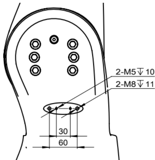
图 7-13 操作机肩部接口尺寸图
