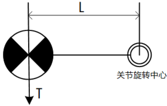
图 7-6 负载离心率示意图
