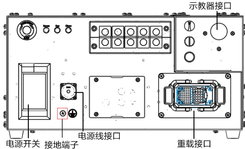
图 6-4 AIR10-1210C(-HW)控制柜示意图
