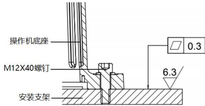
(b)剖面图
