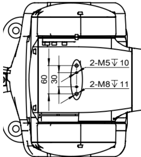
图 7-11 操作机肘部接口尺寸图
