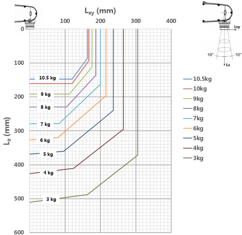
图 7-8 AIR10-1210C(-HW)操作机腕部向下时的负载质心位置示意图
