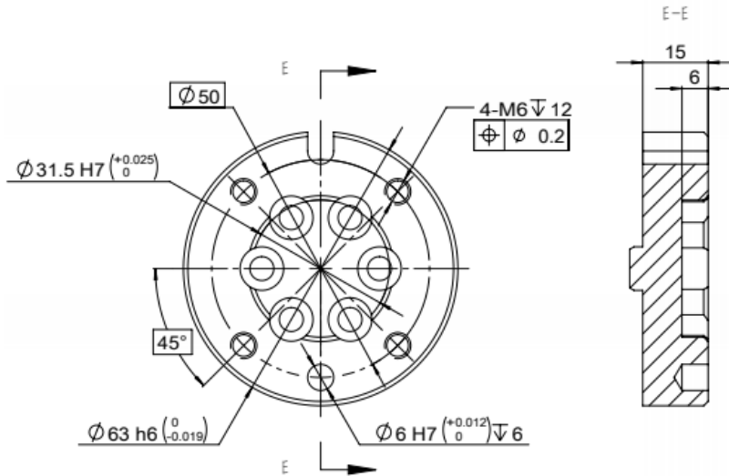
图 7-4 AIR10-1210C 操作机腕部法兰尺寸示意图
