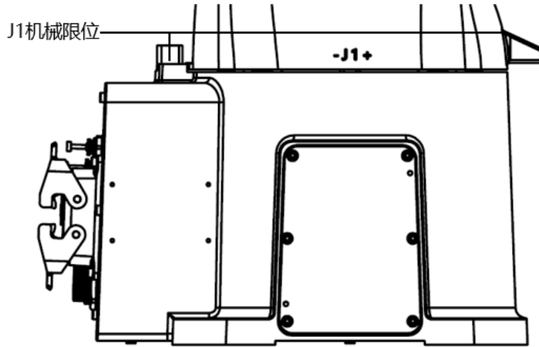
图 7-3 操作机上机械式制动器
