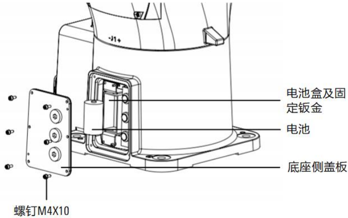
图 12-4 更换电池示意图
