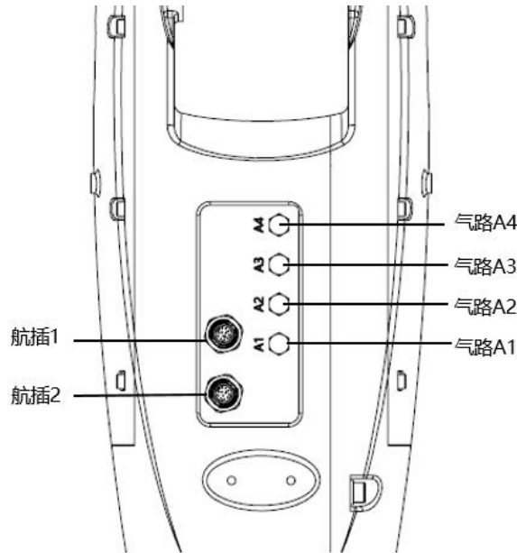
图 5-3 AIR10-1210C-HW 操作机小臂上接口
