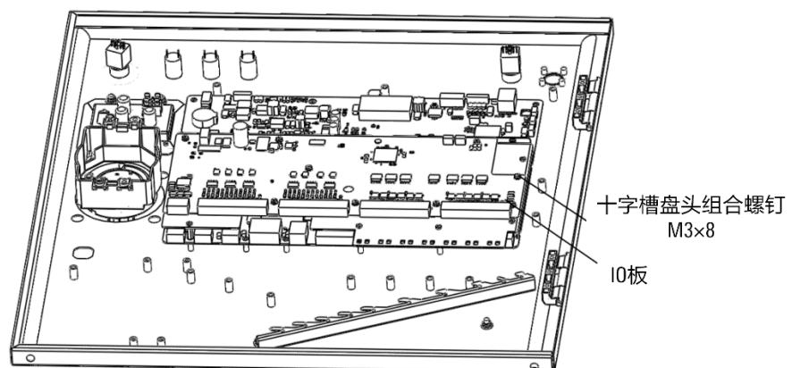
图 20-19 安装 48 路 IO 板
