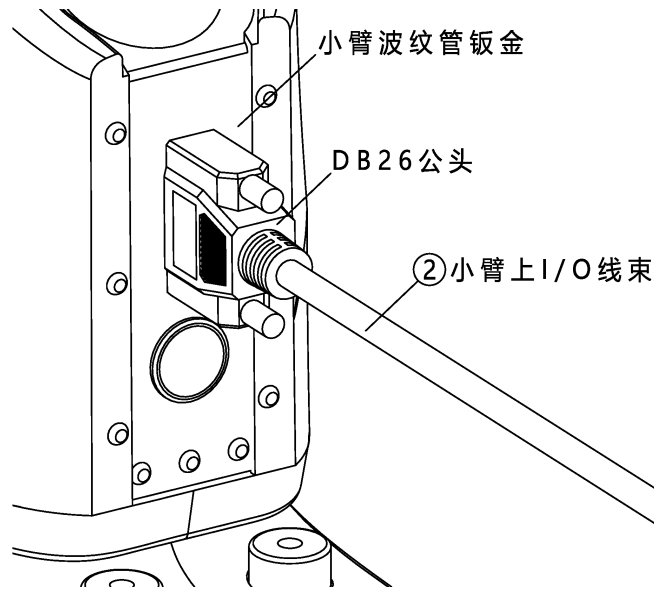
图 5-2 小臂上 I/O 线束连接示意图
