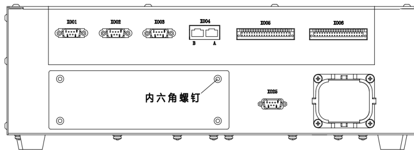
图 21-4 控制柜后面板示意图
