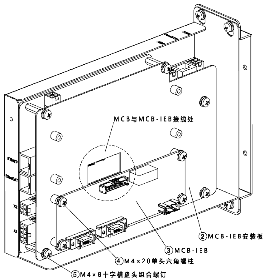
图 21-40 安装 MCB-IEB
