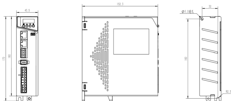
图 28-10 A2E-5R5AI-Q 驱动图纸
