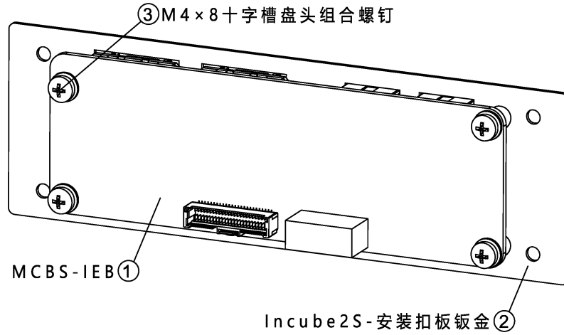
图 21-17 安装 MCBS-IEB
