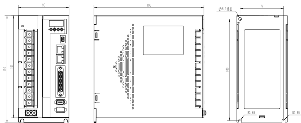
图 28-14 A2E-120AI-Q 驱动图纸
