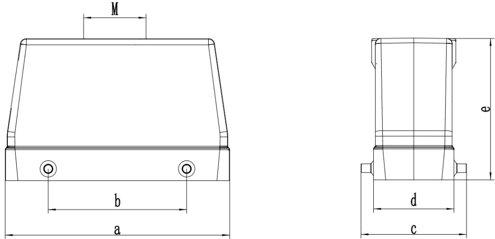
图 9-35 动力线重载接头尺寸
