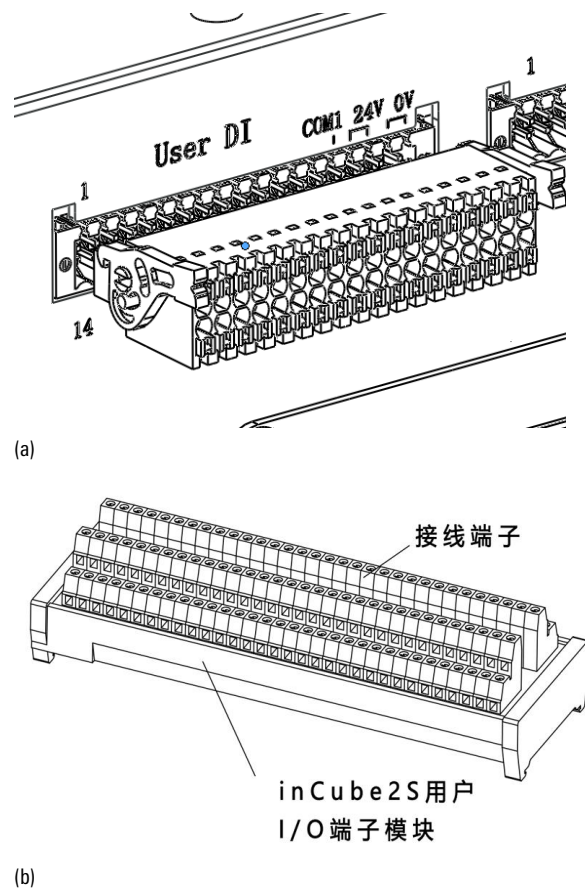
图 19-5 inCube20/22 控制柜用户 DI 模块接线示意图
