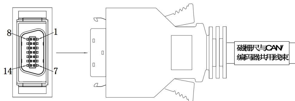
图 21-14 磁栅尺与 CAN_编码器共用线束及 SCSI 引脚示意图
