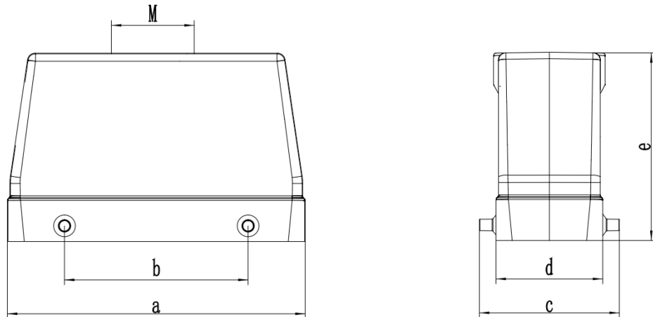
图 9-13 动力线重载接头尺寸
