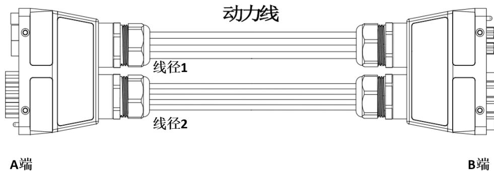
图 9-34 AIR165 动力固定线与 AIR50/75/165 动力拖链线外形示意图
