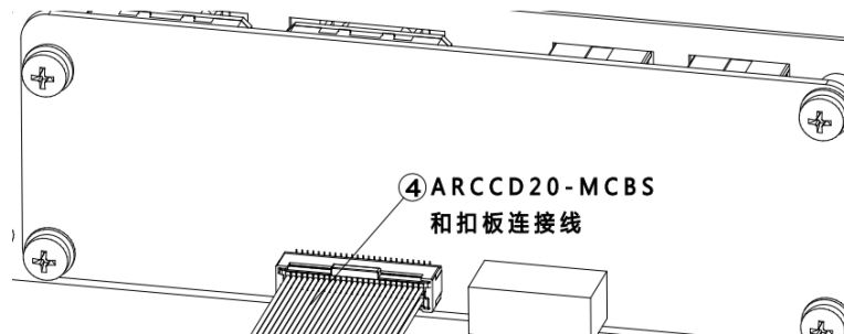
图 21-6 安装 ARCCD20-MCBS 和扣板连接线
