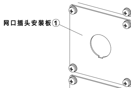
图 12-4 网口插头安装板
