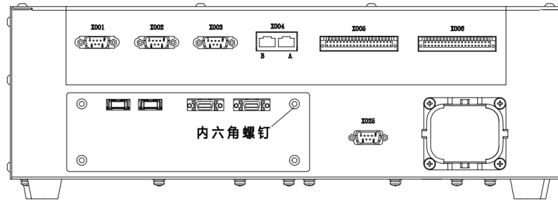
图 21-7 ARCCD20-安装扣板钣金固定后示意图
