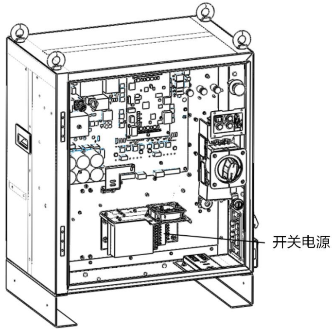
图 20-20 开关电源
