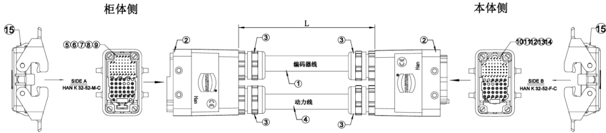
图 9-9 inCube20T 标准重载线示意图
