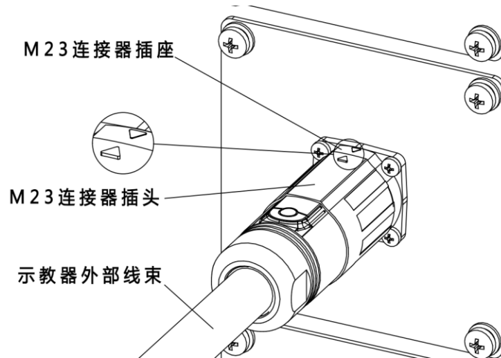
图 10-8 示教器连接接口
