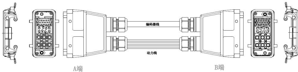
图 9-26 inCube22 重载拖链线外形示意图
