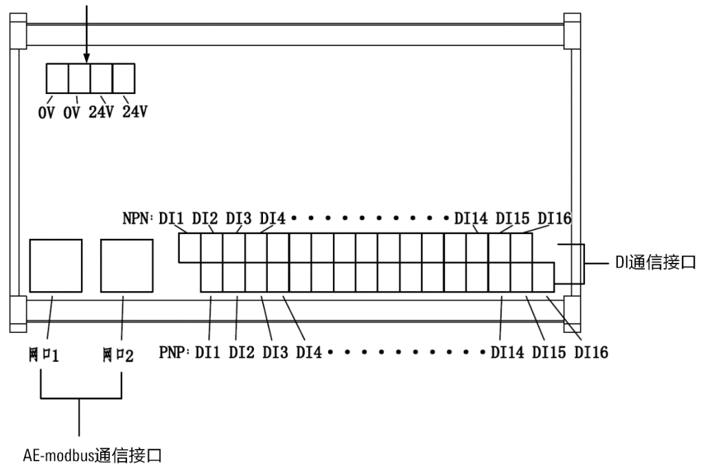
图 20-12 BDI 模块接口示意图
