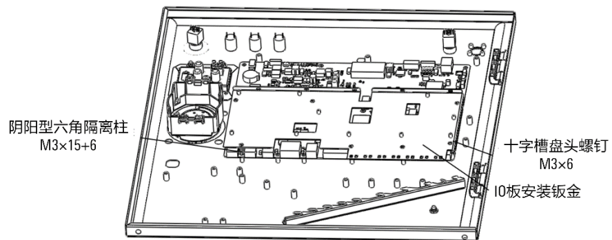
图 20-18 安装 IO 板安装板
