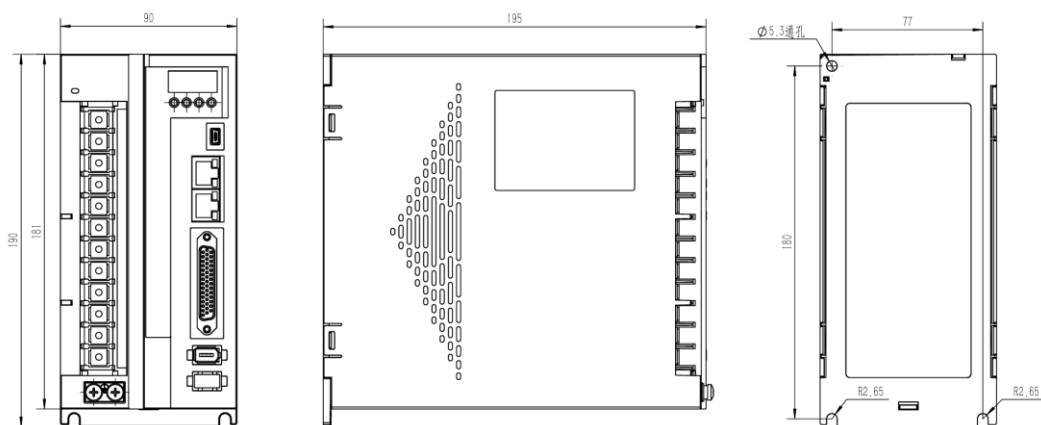
图 28-16 A2E-8R5AI-Q 驱动图纸
