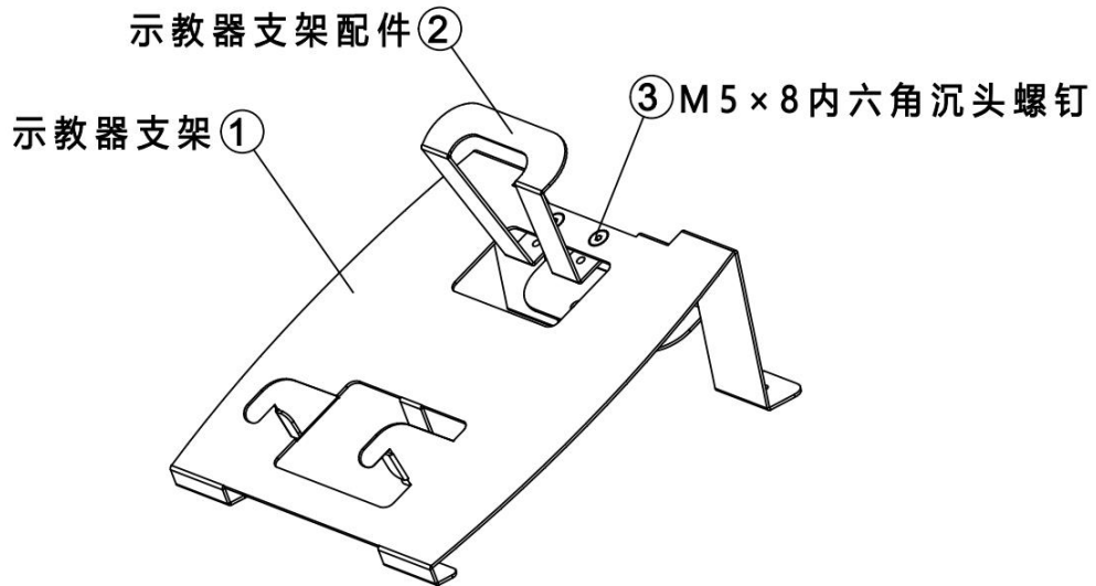
图 26-1 示教器固定装置示意图
