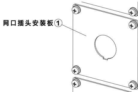
图 16-10 网口插头安装板
