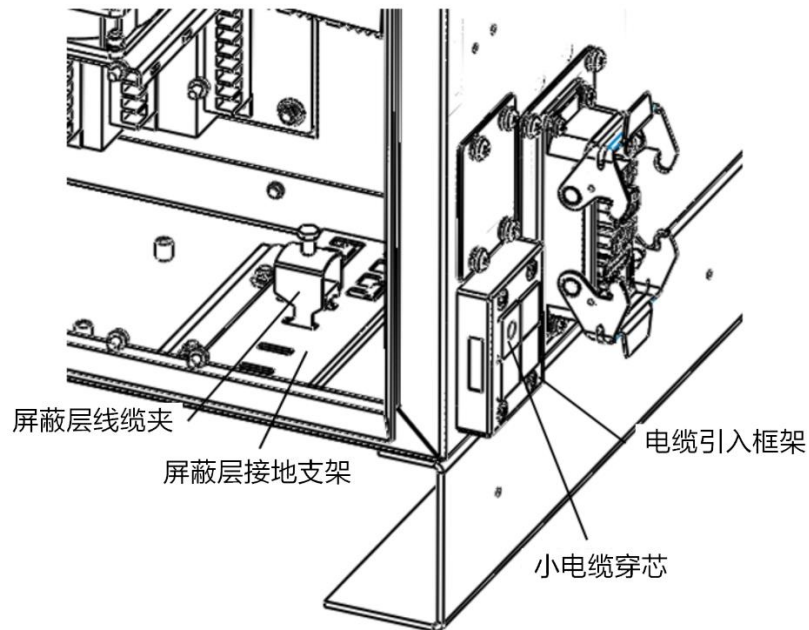
图 8-2 电缆引入的使用
