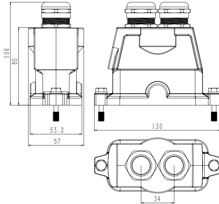
图 9-22 AIR6L-A 本体端重载尺寸图
