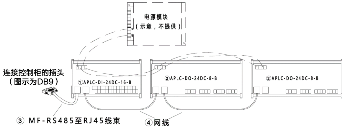
图 20-14 “16 路 DI+16 路 DO” 的连接示意图
