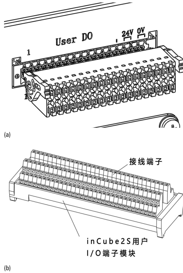
图 19-6 inCube20/22 控制柜用户 D0 模块接线示意图
