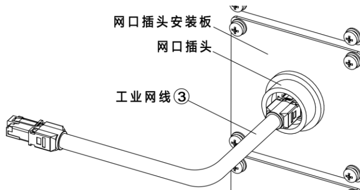
图 14-6 工业网线连接网口插头示意图
