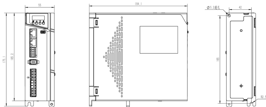
图 28-12 A2E-8R0AI-Q 驱动图纸
