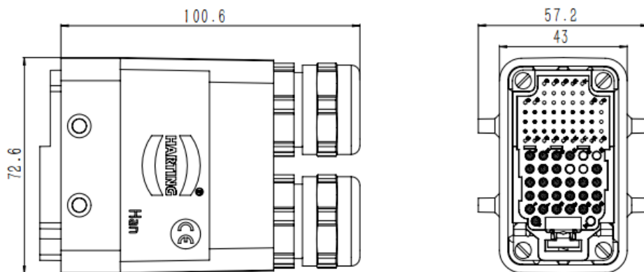
图 9-30 inCube20T 重载接头尺寸
