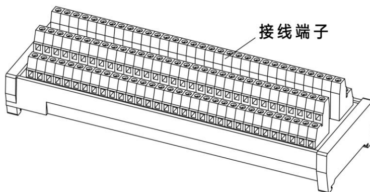
图 19-4 inCube20/22/ARC5 用户 I/O 连接端子台示意图
