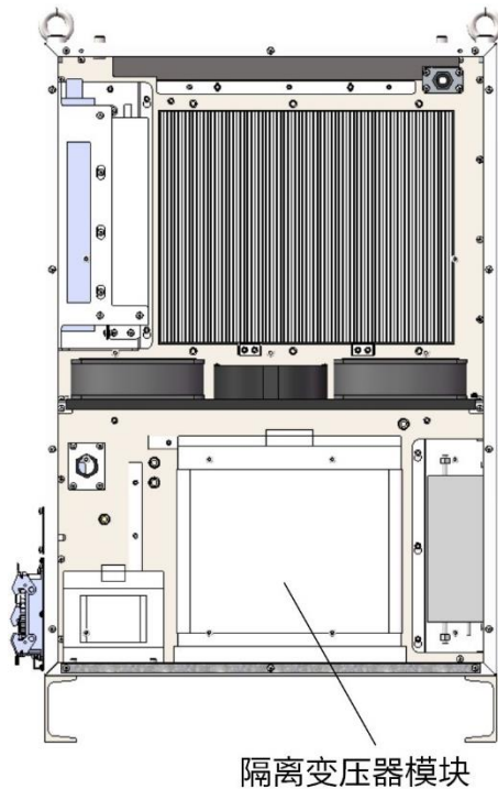
图 7-1 隔离变压器在 ARC5-280 柜内示意图
