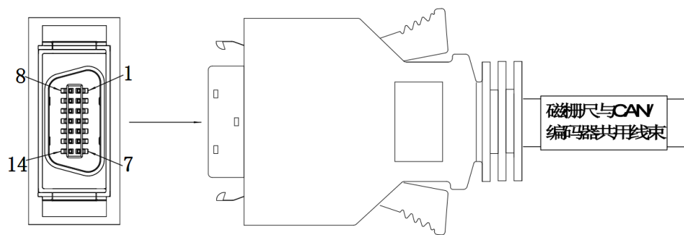
图 21-26 磁栅尺与 CAN_编码器共用线束及 SCSI 引脚示意图
