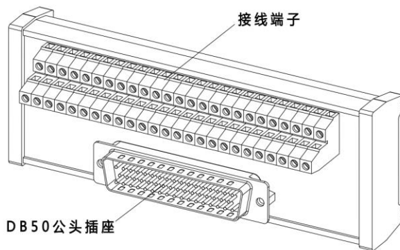
图 19-9 用户 I/O 端子模块
