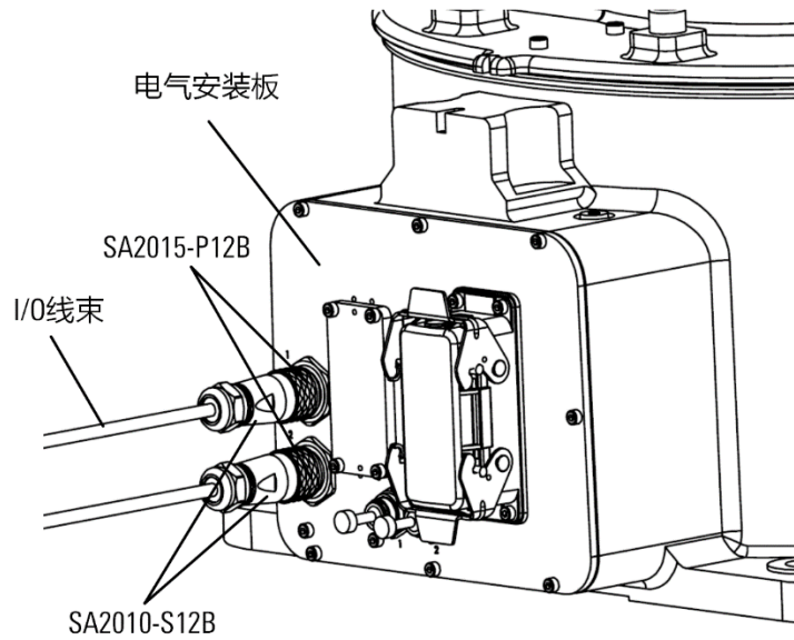
图 5-3 基座上 I/O 线束连接示意图
