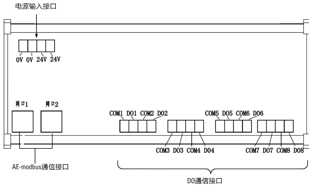
图 20-13 BDO 模块接口示意图
