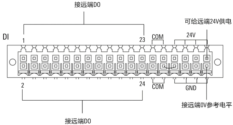
图 20-16 User DI 接口使用说明（PNP 输入）
