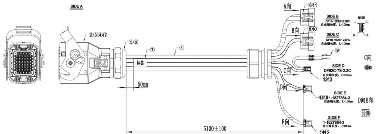
图 9-29 inCube2S-20 拖链重载线示意图
