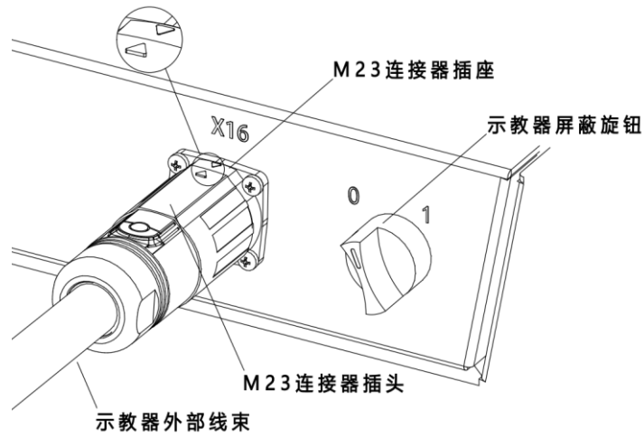
图 10-2 示教器连接接口
