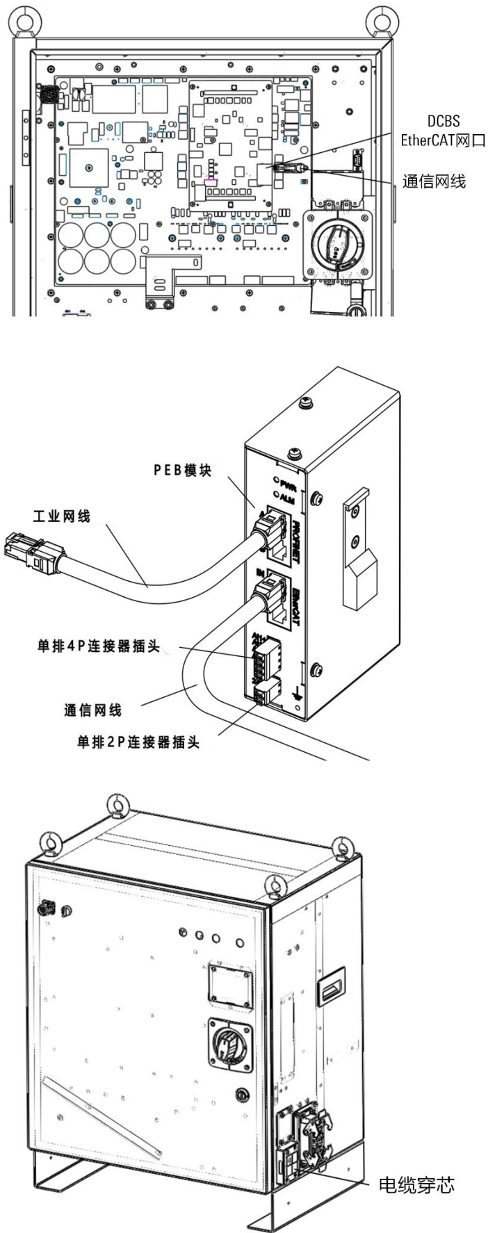
图 16-8 PEB 模块接线
