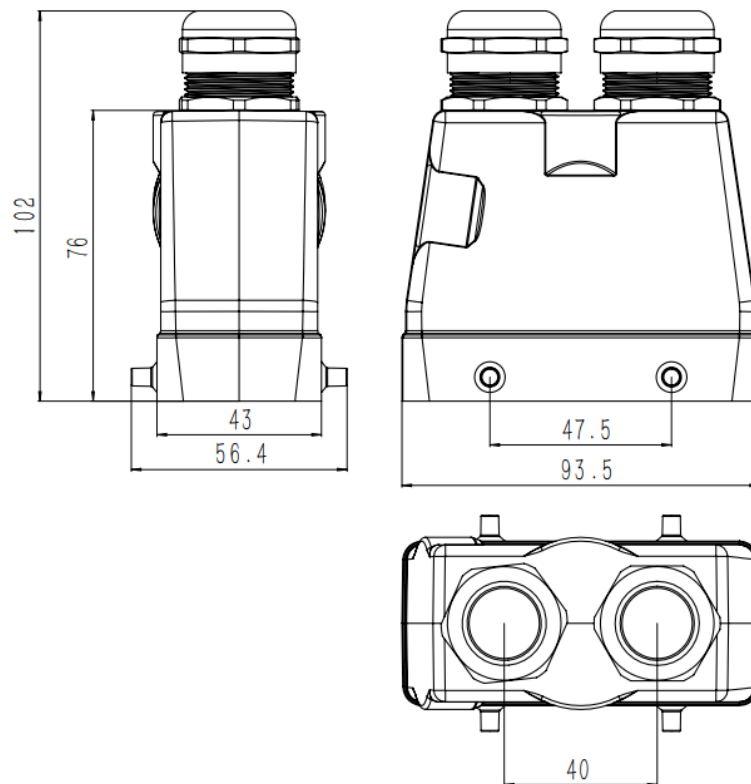
图 9-21 AIR8-710A/AIR10-1420A 机型本体端重载插头尺寸
