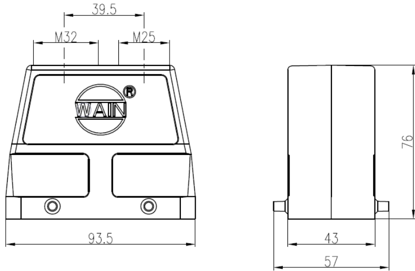
图 9-24 inCube22 重载接头尺寸
