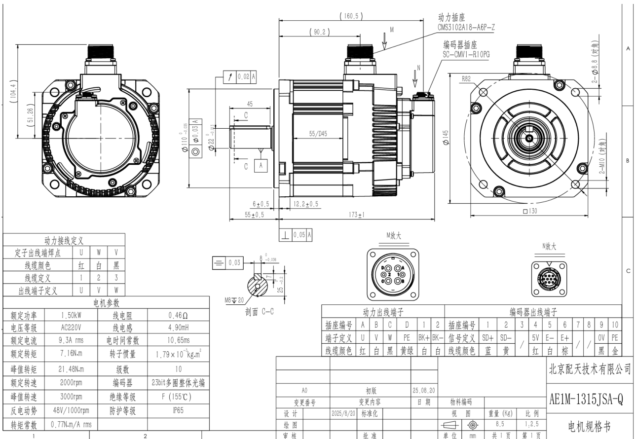
图 28-11 AE1M-1315JSA-Q 电机图纸
