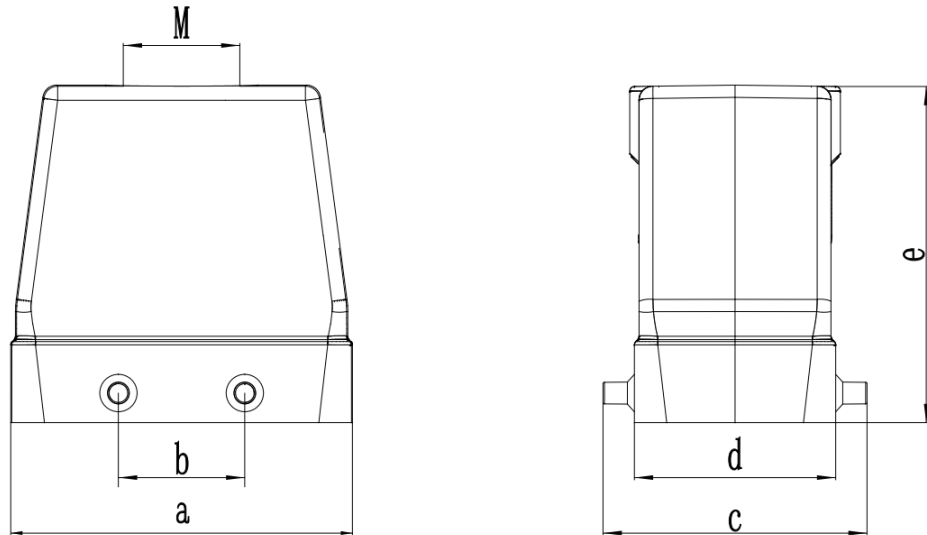
图 9-33 编码器线重载接头尺寸
