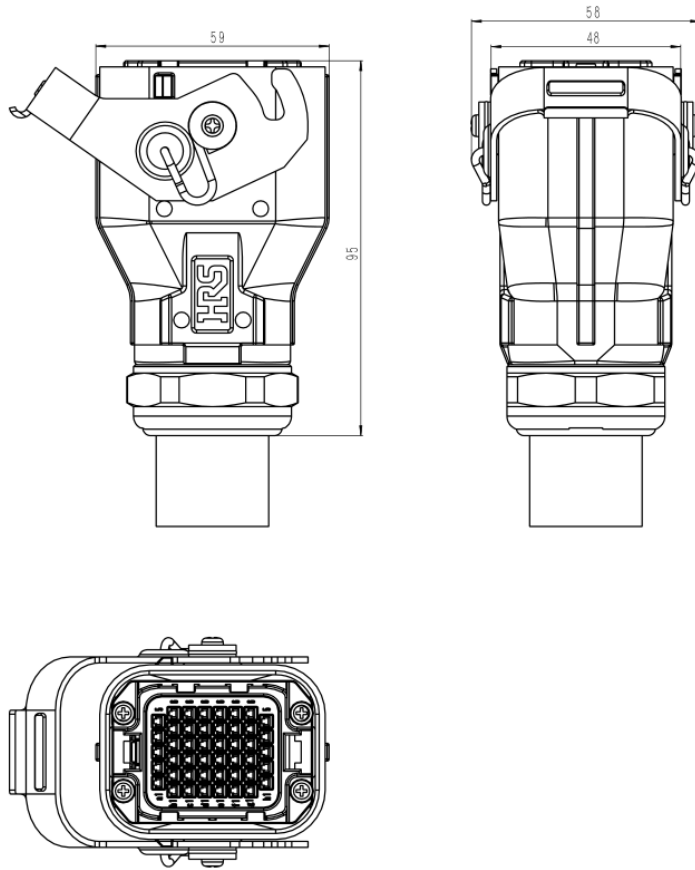
图 9-2 inCube20/inCube2S/inCube20-HP/ARC5-12 重载接头尺寸
