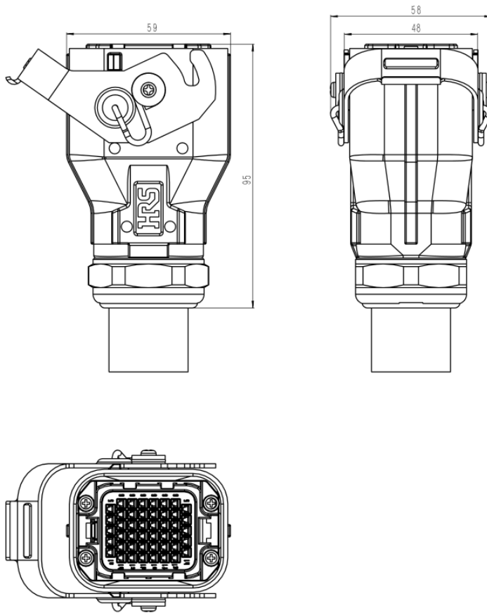
图 9-27 inCube20/2S 重载接头尺寸
