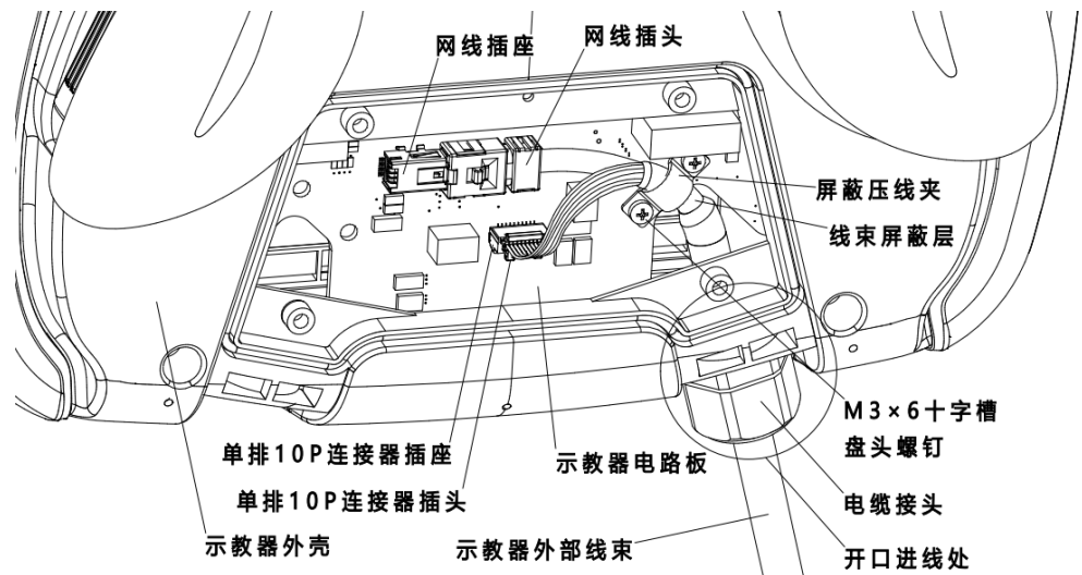
图 10-7 更换示教器外部线束示意图 2
