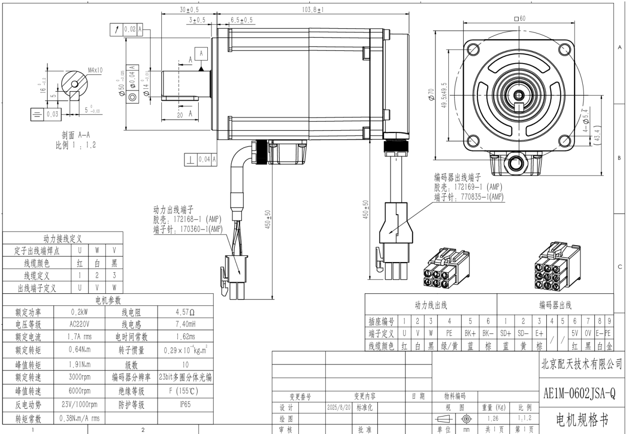
图 28-3 AE1M-0602JSA-Q 电机图纸
