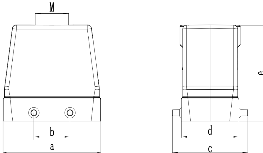
图 9-11 编码器线重载接头尺寸
