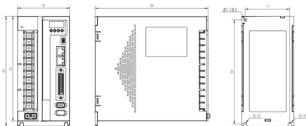
图 28-18 A2E-160AI-Q 驱动图纸
