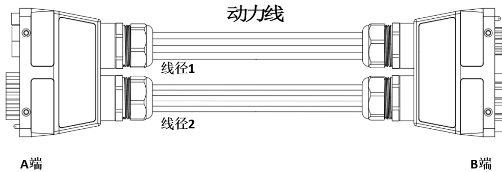
图 9-14 ARC4-165 动力线示意图
