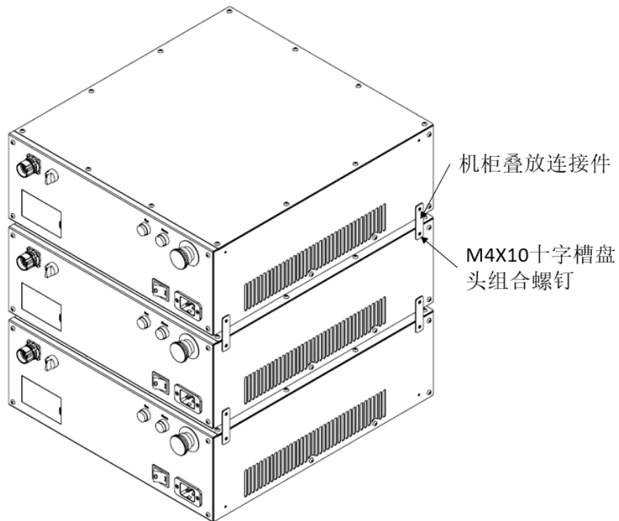
图 25-2 inCube20/22 控制柜叠放效果
