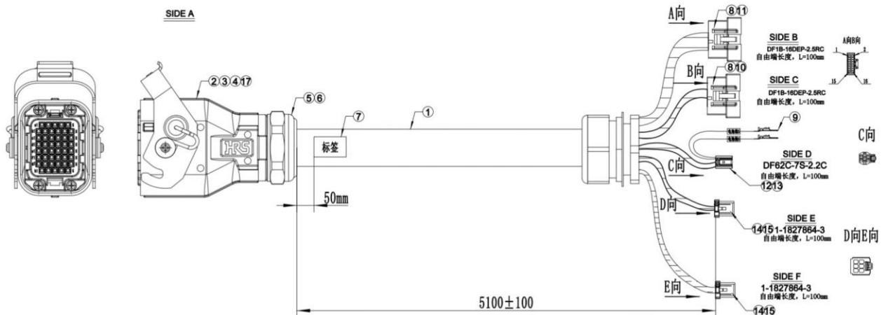
图 9-8 inCube2S-20 标准重载线 (AIR12SC/AIR20SC 机型) 示意图
