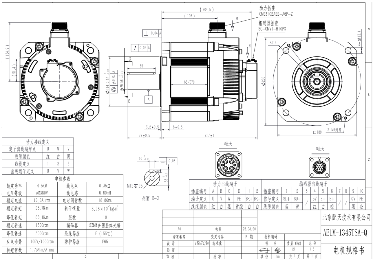
图 28-21 AE1M-1345TSA-Q 电机图纸
