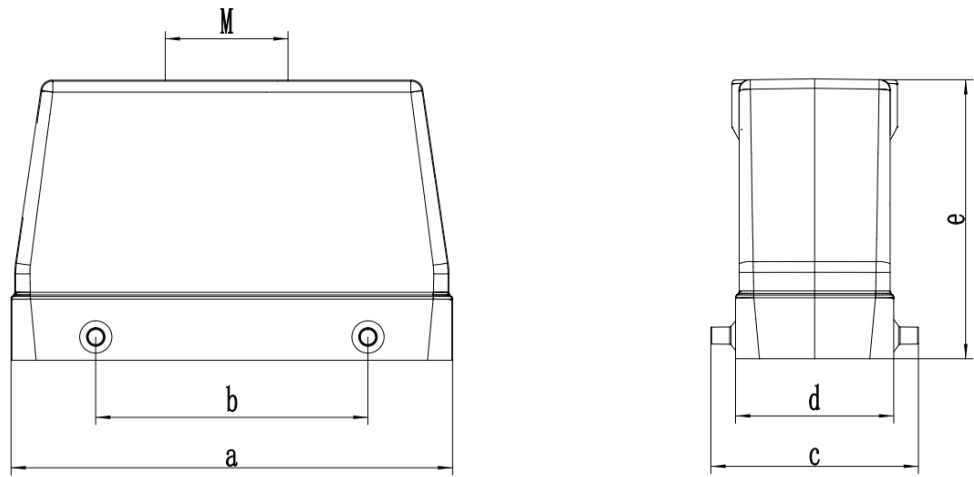
图 9-16 动力线重载插头尺寸示意图
