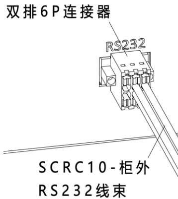
图 13-1 SCRC10-柜外 RS232 线束接线示意图
