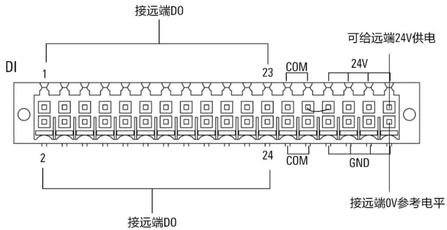
图 20-15 User DI 接口使用说明 (NPN 输入)
