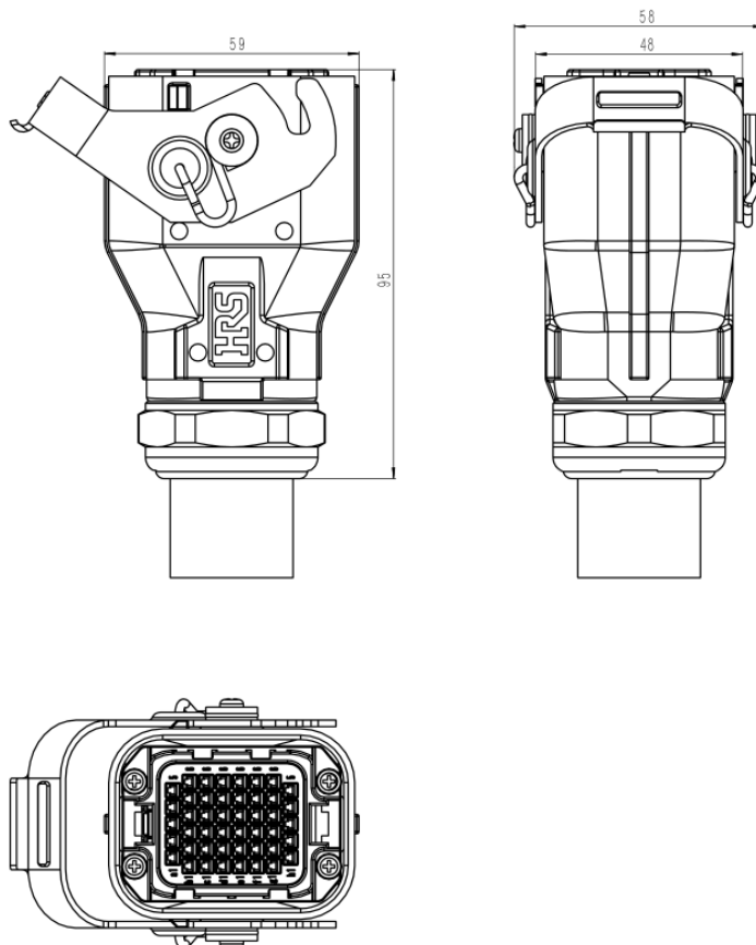
图 9-23 inCube20/2S 重载接头尺寸
