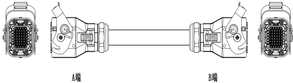
图 9-5 inCube20 标准重载线（适配 AIR4-560A/AIR6-1450A 机型）示意图
