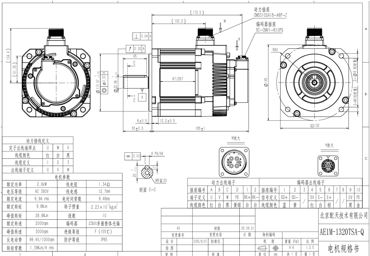
图 28-15 AE1M-1320TSA-Q 电机图纸
