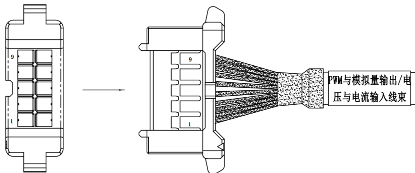
图 21-27 PWM 与模拟量输出_电压与电流输入线束(5m)示意图
