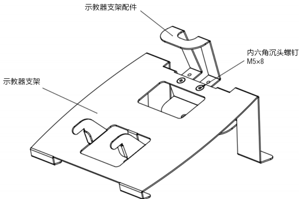
图 26-4 示教器固定装置示意图
