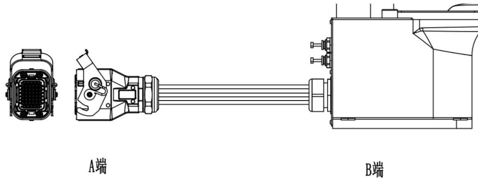
图 9-28 inCube2S-6 拖链重载线示意图
