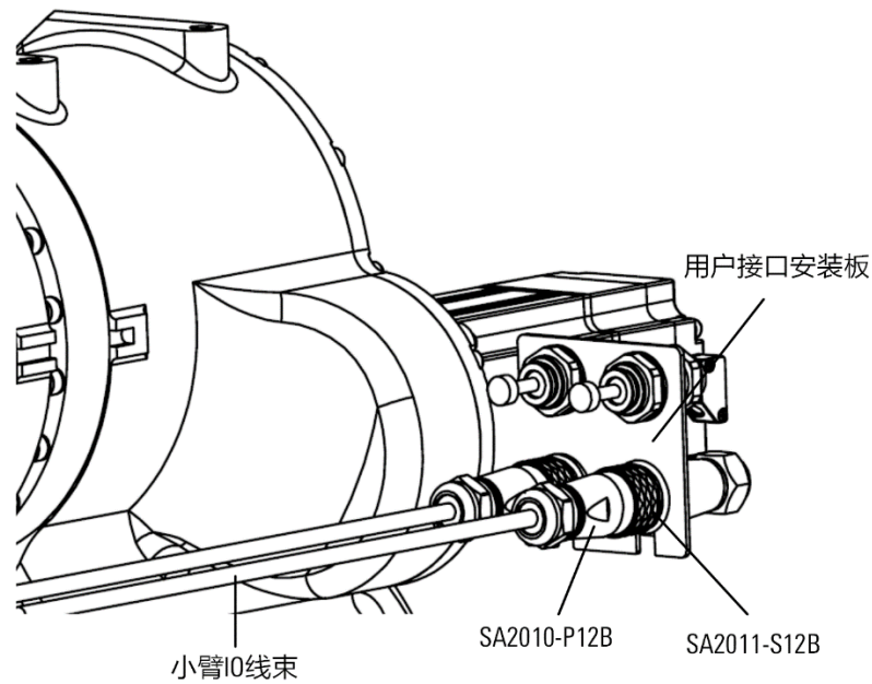
图 5-4 小臂上 I/O 线束连接示意图
