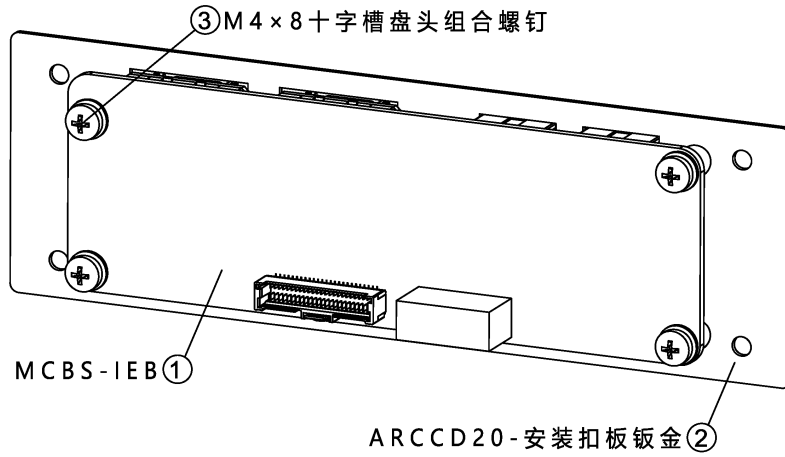
图 21-5 安装 MCBS-IEB
