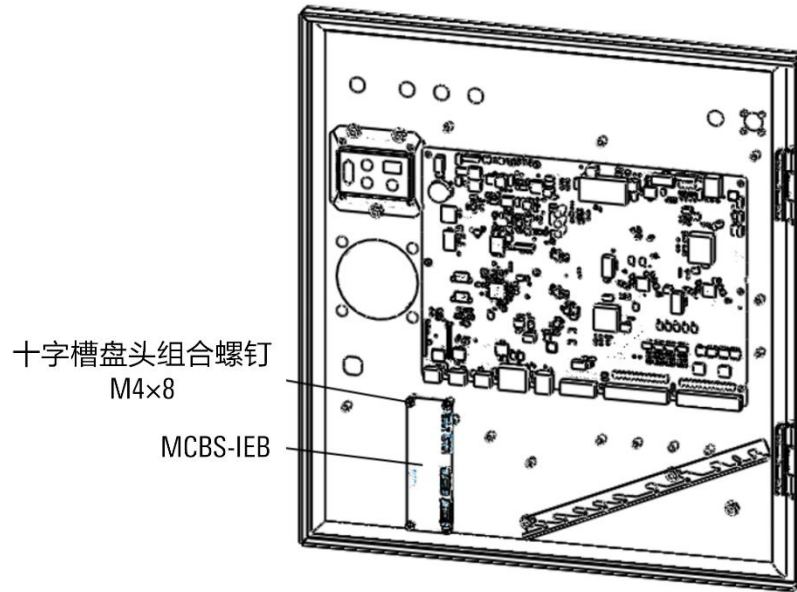
图 21-30 MCBS-IEB 安装示意图
