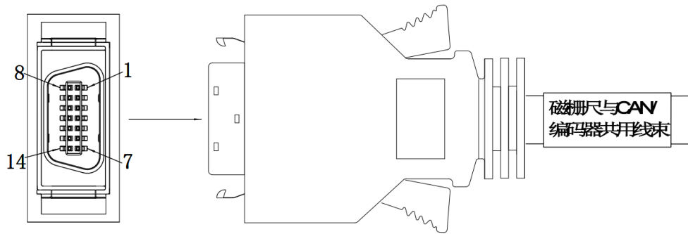
图 21-2 磁栅尺与 CAN_编码器共用线束及 SCSI 引脚示意图
