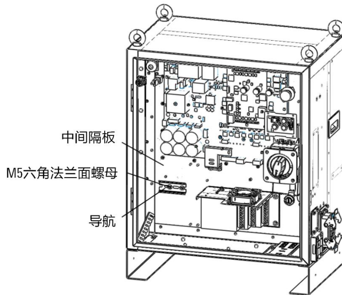
图 16-6 安装导轨
