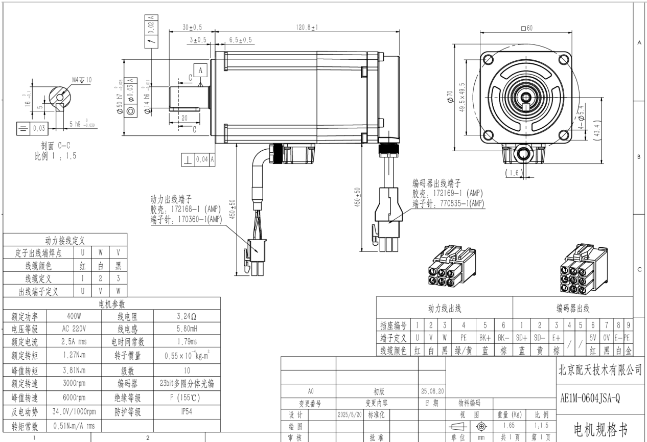
图 28-5 AE1M-0604JSA-Q 电机图纸
