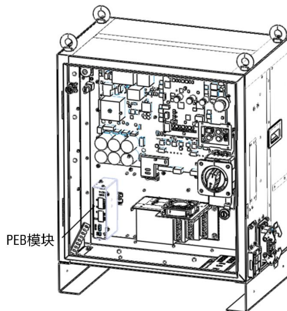
图 16-7 将 PEB 模块安装在导轨上
