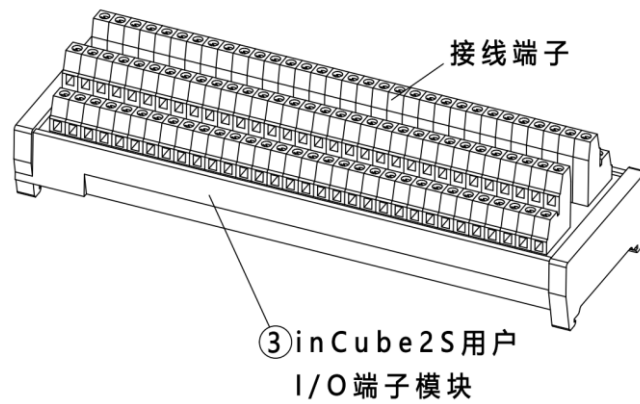
图 19-3 inCube2S 控制柜用户 D0 模块接线示意图
