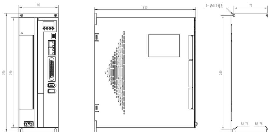
图 28-20 A2E-100TI-0 驱动图纸
