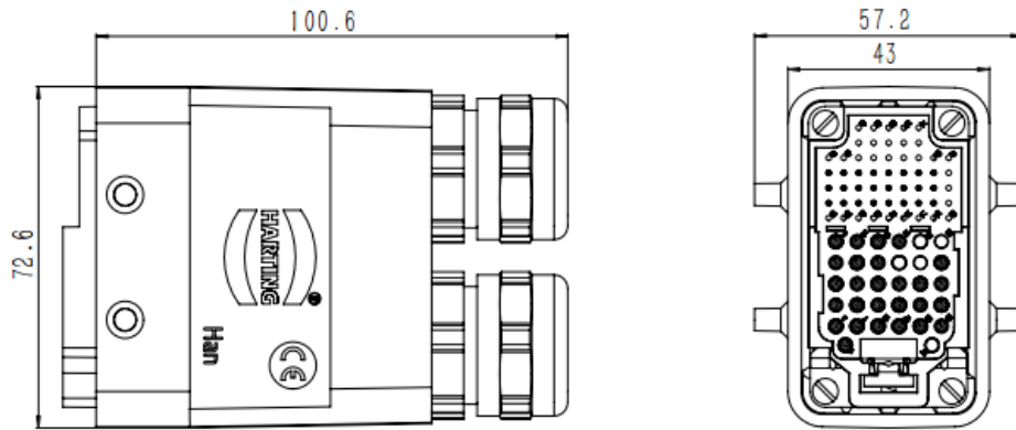
图 9-4 inCube20T/inCube20T-HP/ARC5-12T 重载插头尺寸图
