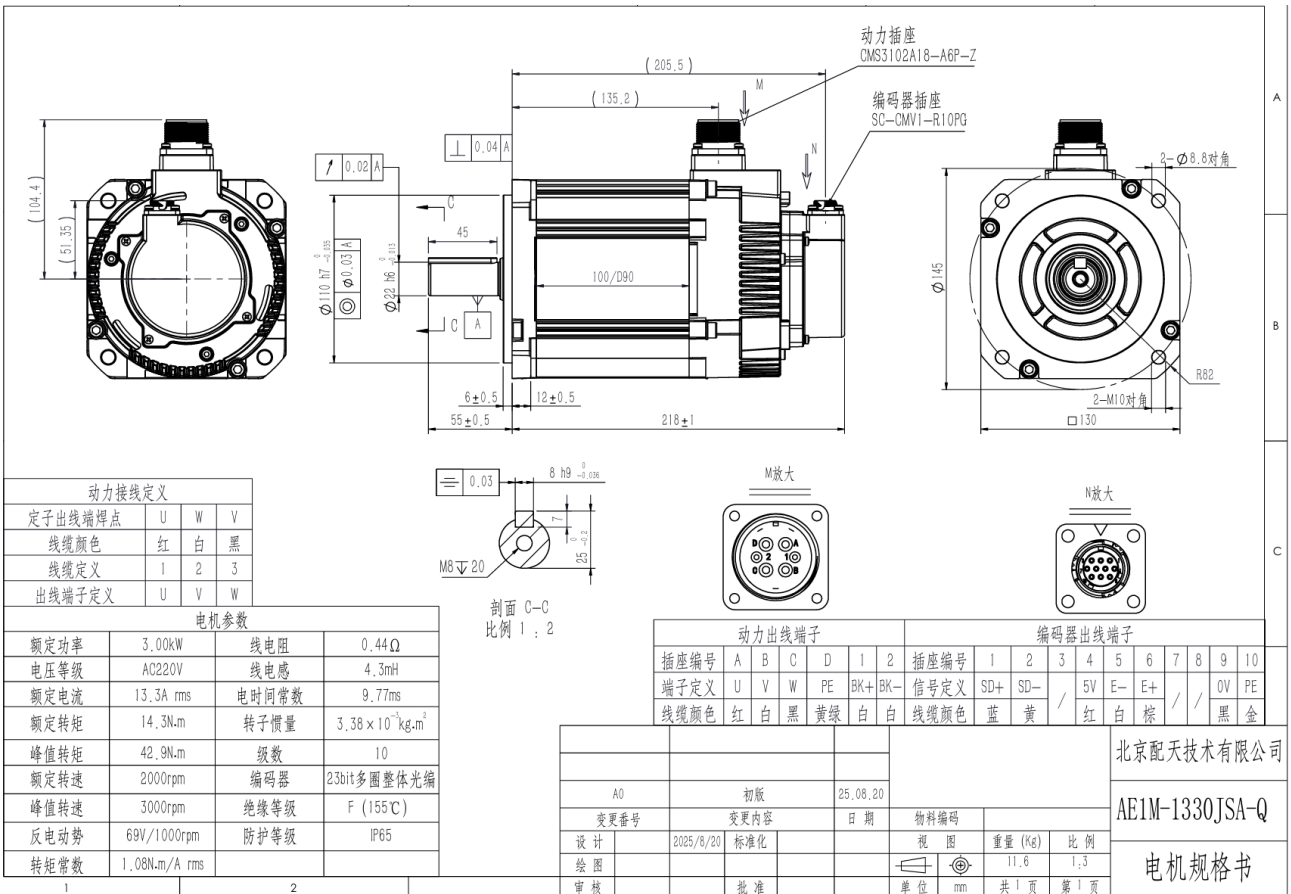
图 28-17 AE1M-1330JSA-Q 电机图纸
