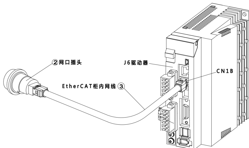
图 16-12 连接 J6 驱动器的 CN1B 接口示意图
