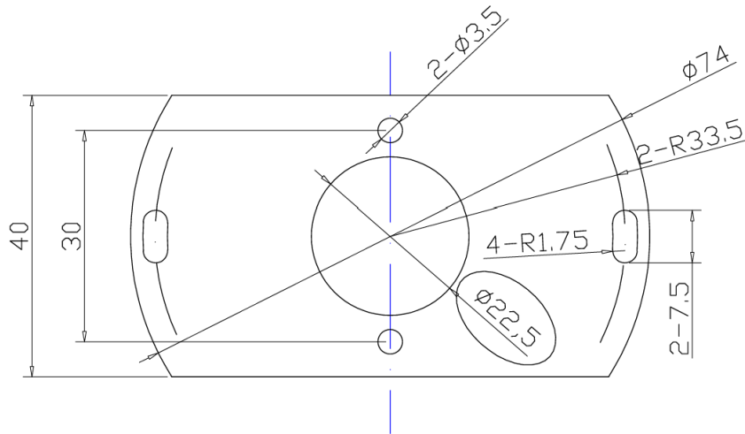
图 29-1 安装支架尺寸图
