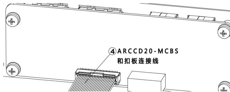
图 21-18 安装 ARCCD20-MCBS 和扣板连接线
