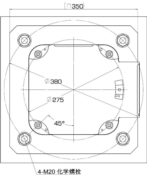
(a) 平面布置尺寸
