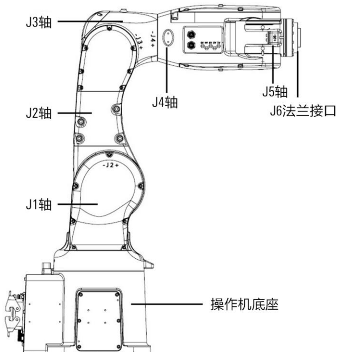
图 2-4 AIR7-920C-HW 型机器人本体及其各个部分
