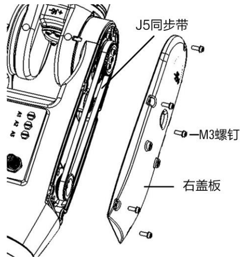
图 9-8 AIR7-920C(-HW)拆卸盖板
