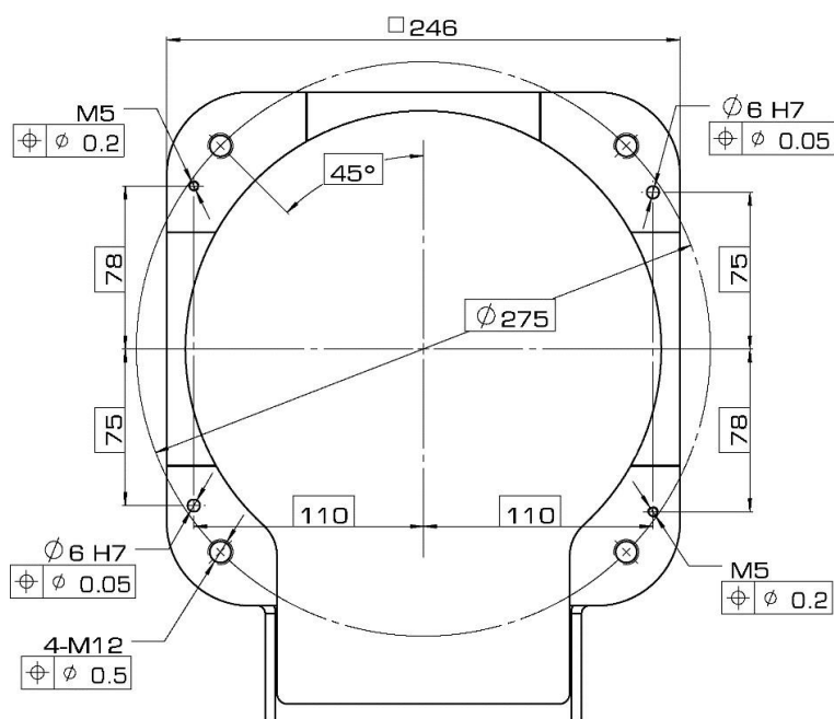
图 3-8 AIR7-920C(-HW)型操作机基座接口尺寸
