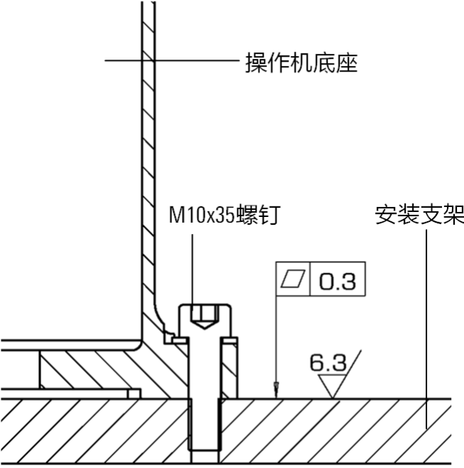
(b) 剖面图
