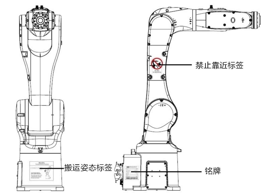
图 2-5 AIR7-920C(-HW)标签位置示意图
