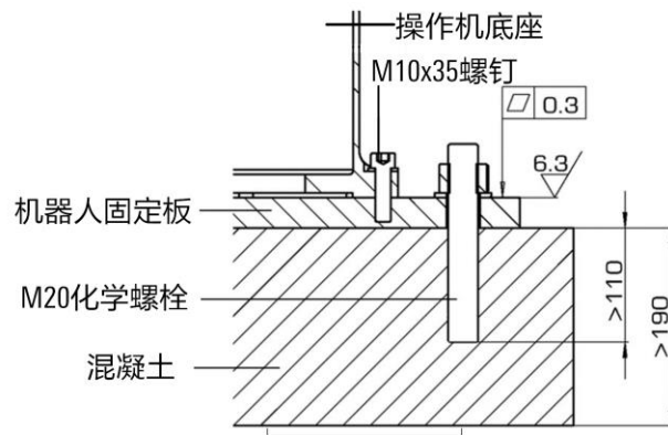
(b) 剖面图
