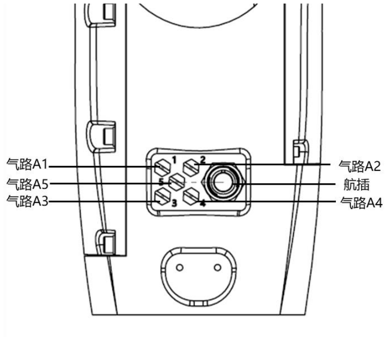
图 4-3 AIR7-920C 型操作机小臂上接口
