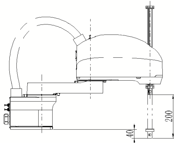
(b) 正视图
