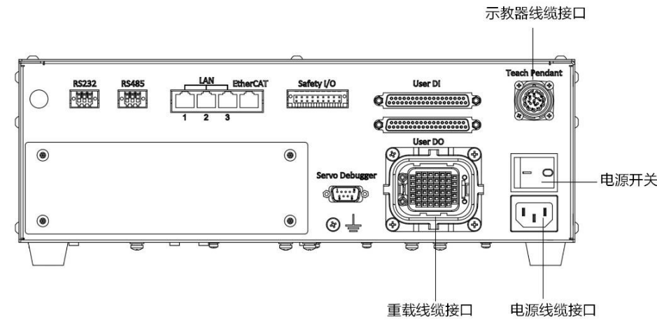
图 4-4 AIR6SC-500A 控制柜示意图
