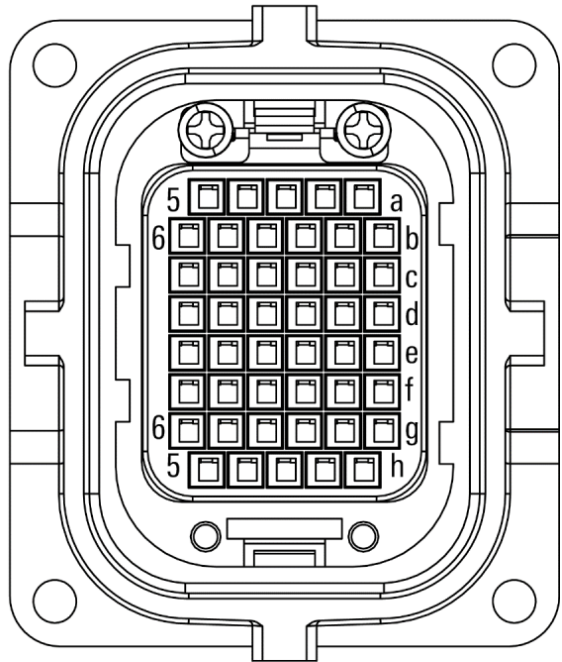
图 4-3 AIR6SC-500A 型操作机重载接口
