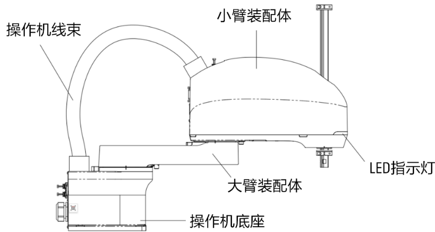
图 2-2 AIR6SC-500A 型机器人本体及其各个部分
