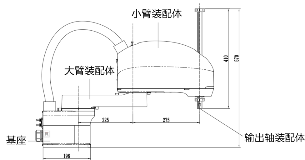
图 5-1 AIR6SC-500A 操作机组件装配体尺寸
