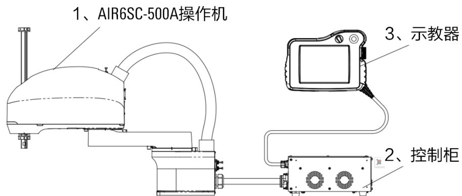
图 2-1 AIR6SC-500A 工业机器人系统的构成
