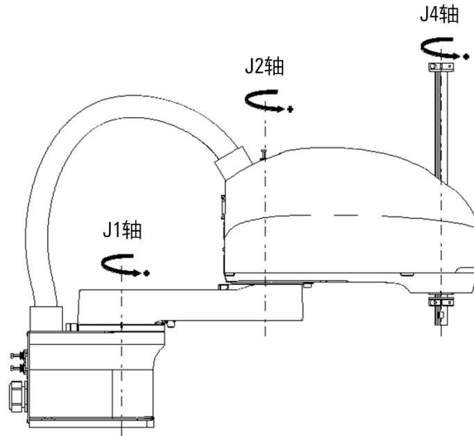
图 5-8 AIR6SC-500A 操作机各轴运动方向示意图
