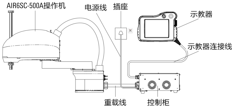
图 4-9 AIR6SC-500A 工业机器人系统接线概览
