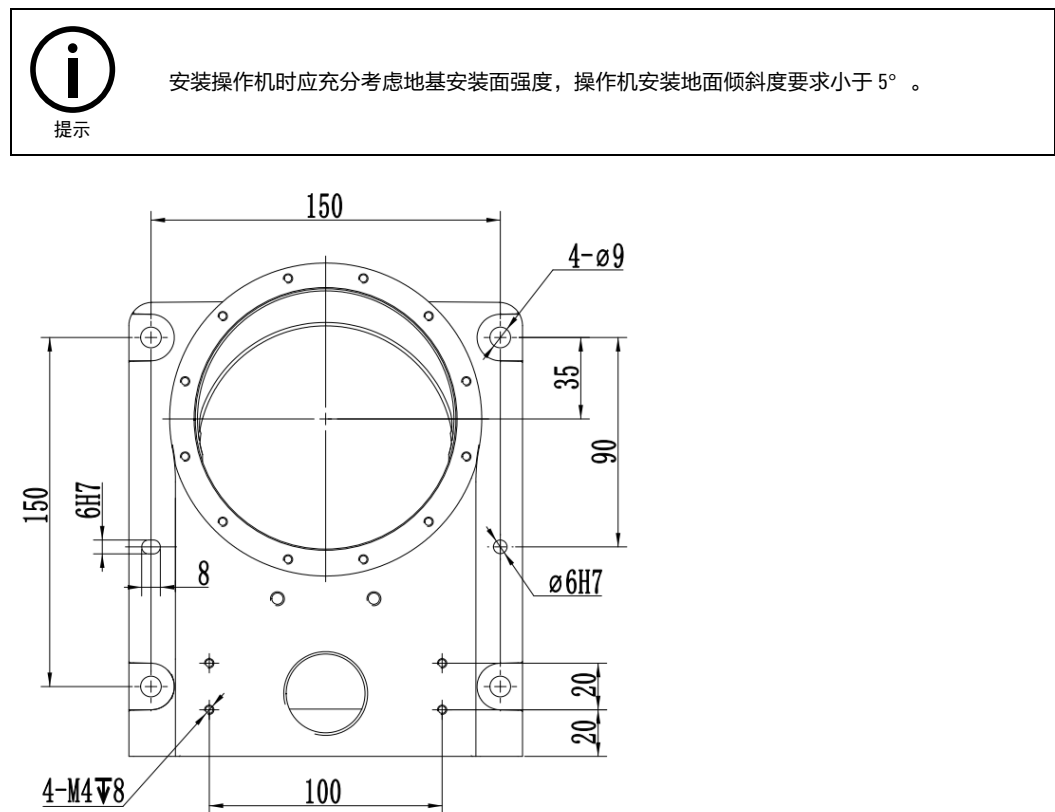
图 3-2 AIR6SC-500A 型操作机基座接口尺寸
