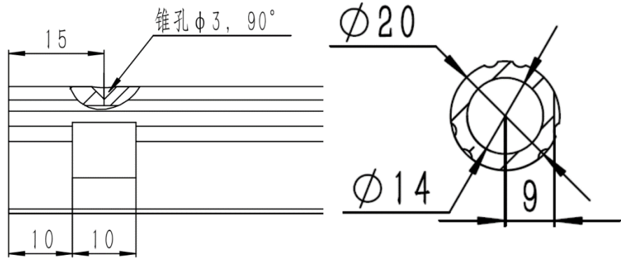
图 5-9 AIR6SC-500A 型操作机腕部法兰尺寸示意图
