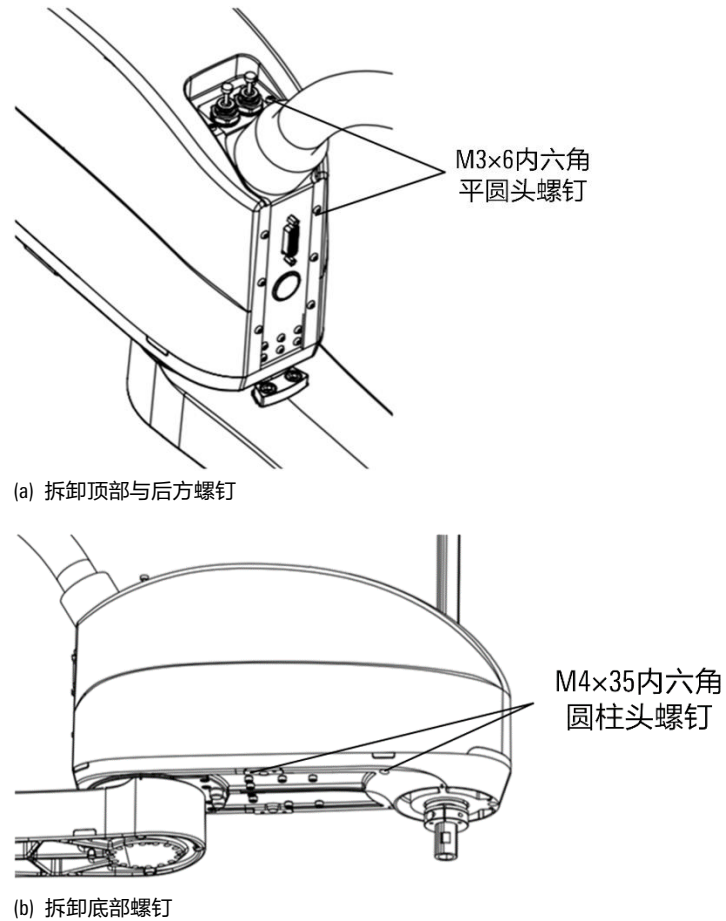
图 8-12 拆卸小臂外壳螺钉示意图
