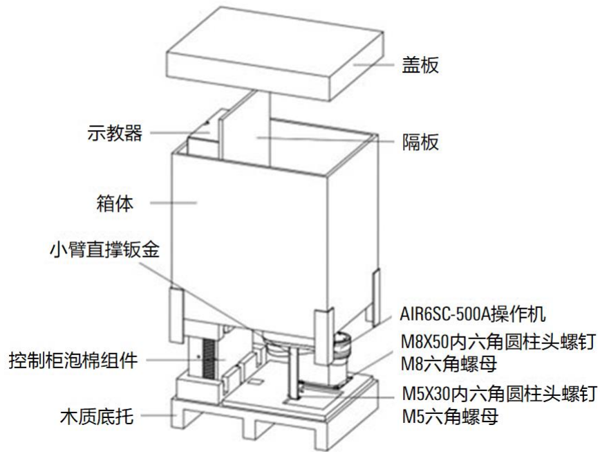
图 3-1 操作机包装示意图
