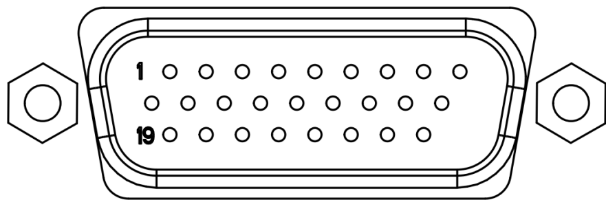
图 4-7 AIR6SC-500A 型操作机基座 I/O 输入接口
