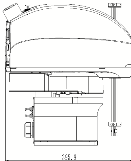
(b) 左视图
