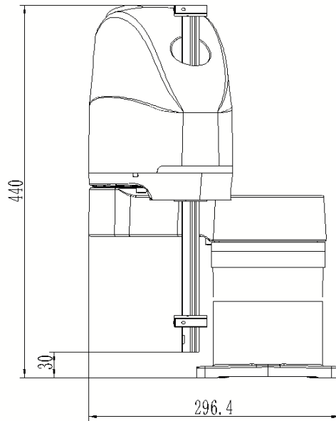
(a) 主视图
