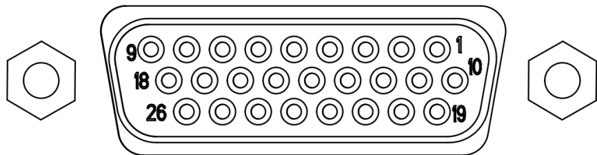
图 4-8 AIR6SC-500A 型操作机小臂 I/O 输出接口
