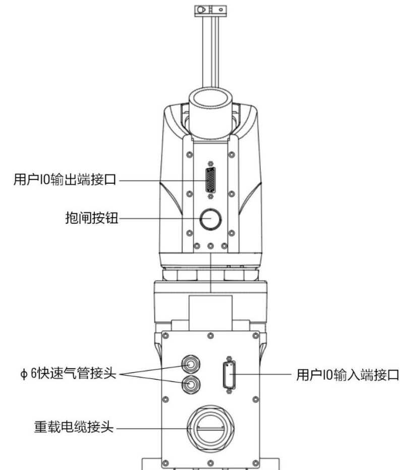
(a) 后视图
