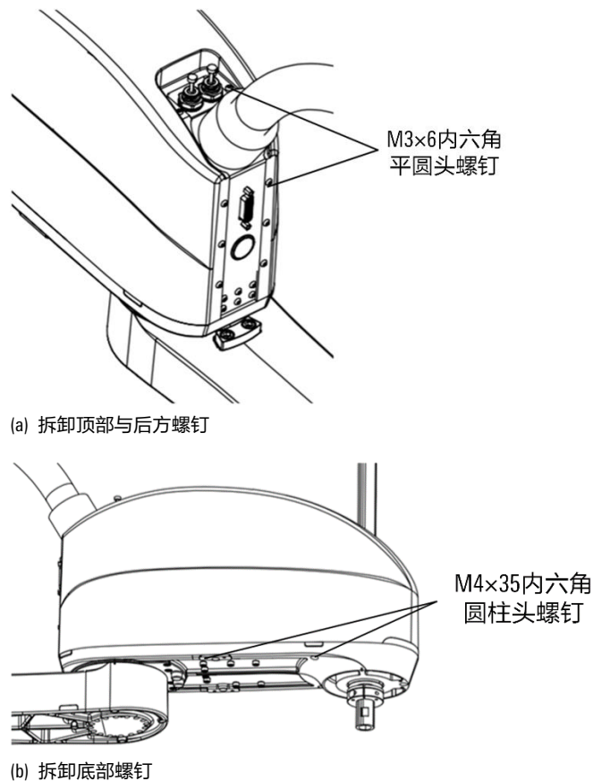
图 8-10 拆卸小臂外壳螺钉示意图
