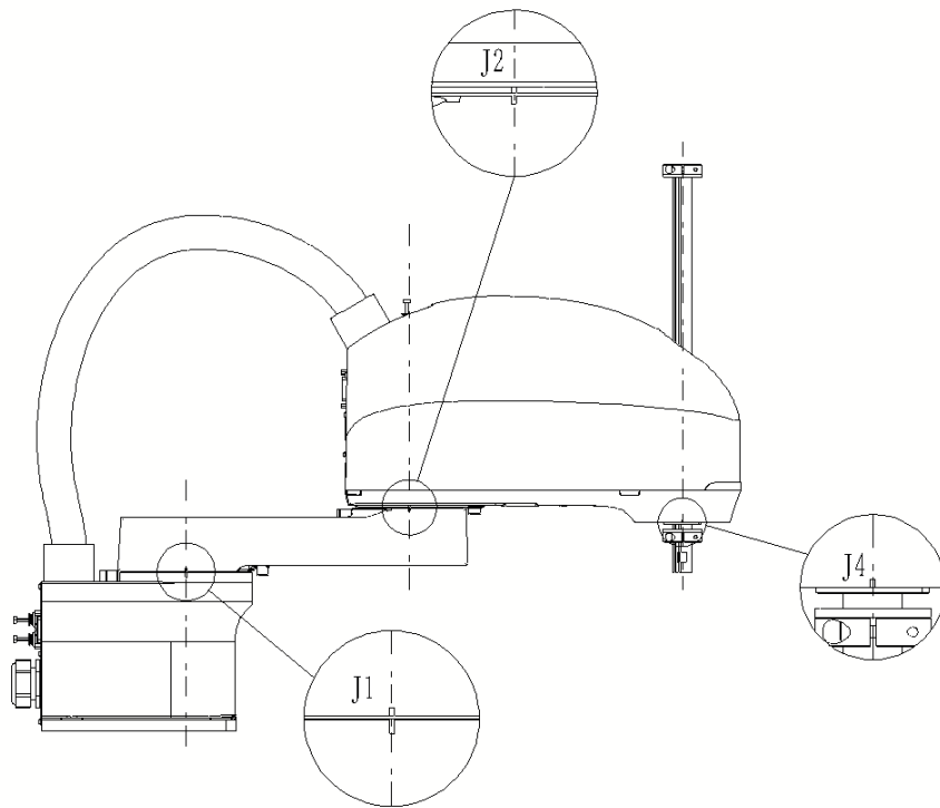
图 5-4 AIR6SC-500A 各轴零点示意图
