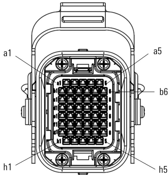
图 3-2 ARC5-12 控制柜重载控制柜接口
