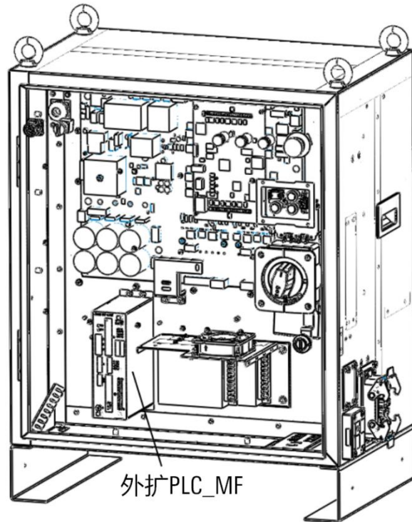
图 5-8 外扩 PLC_MF 模块
