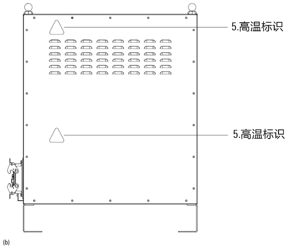
图 1-3 控制柜所含标签位置示意图
