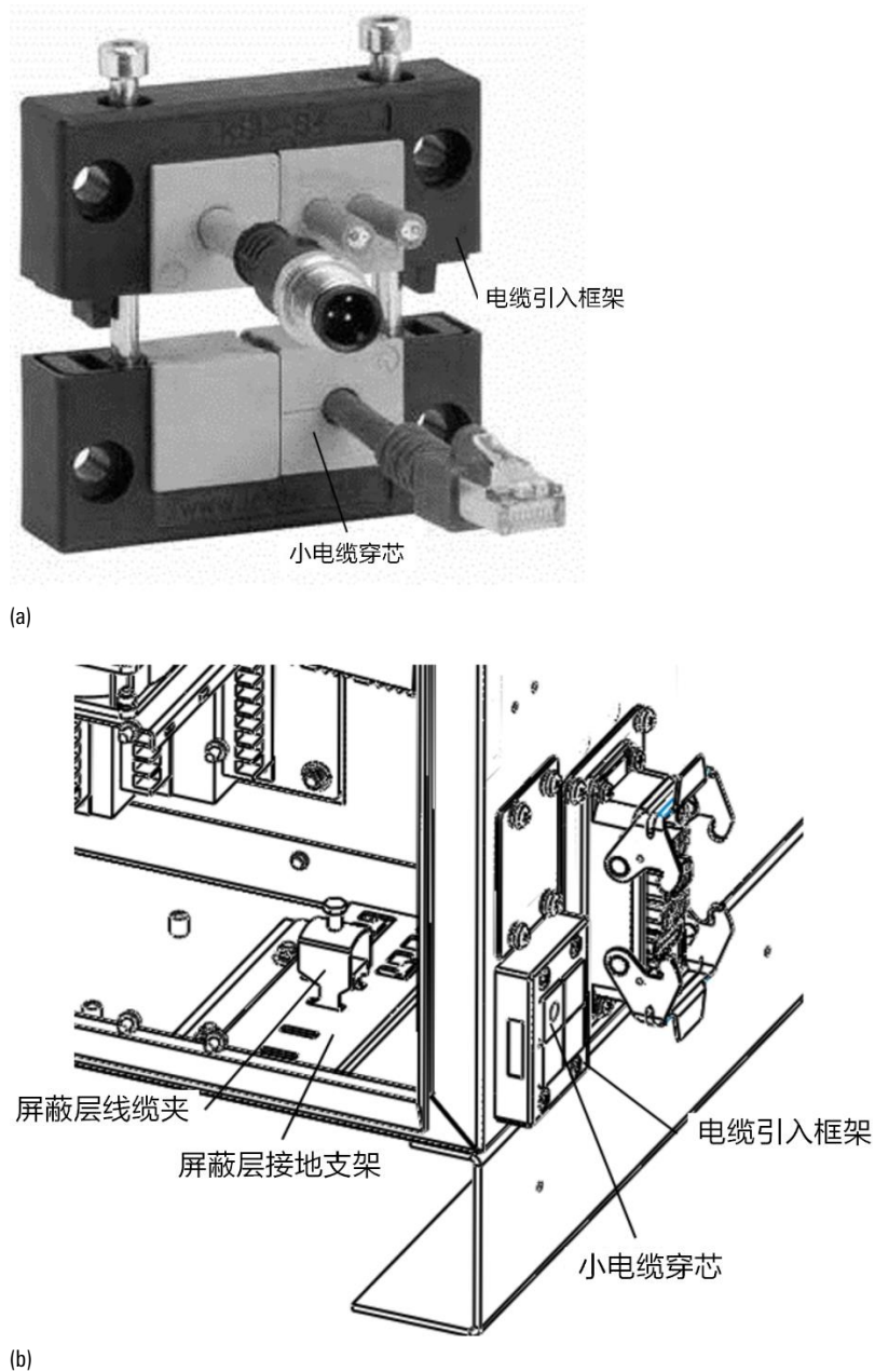
附图 8-1 电缆引入的使用
