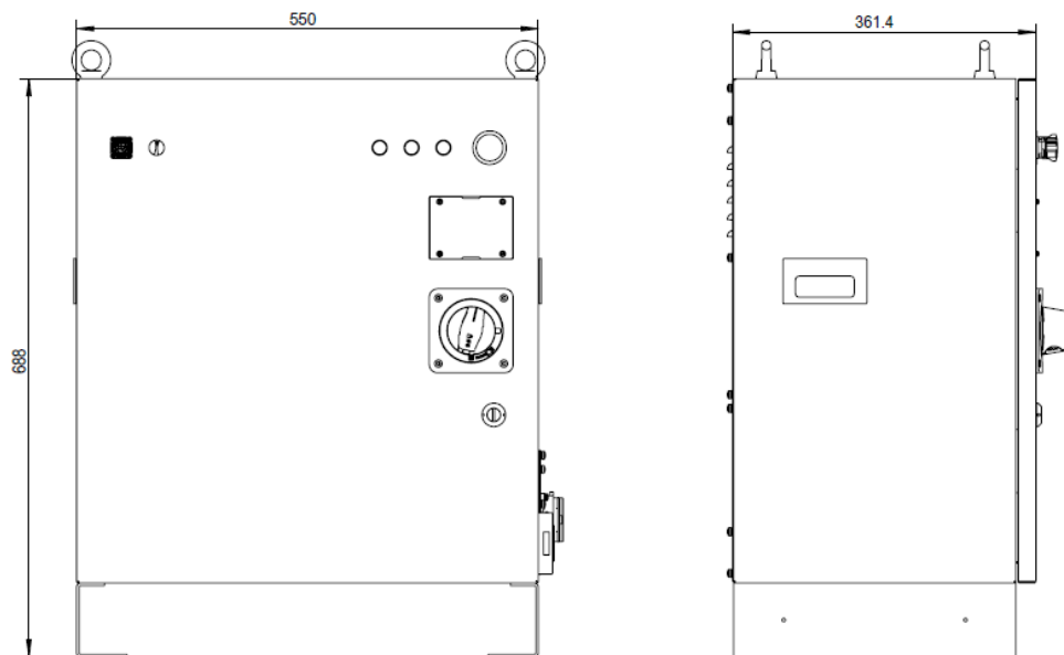
图 3-1 控制柜外观
