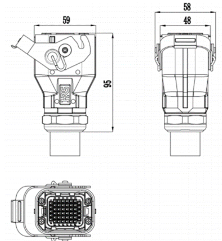
图 3-2 ARC5-12 动力线编码器接口
