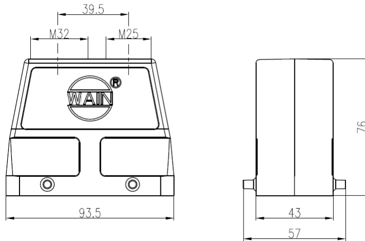
图 3-3 ARC5-25 重载插头尺寸
