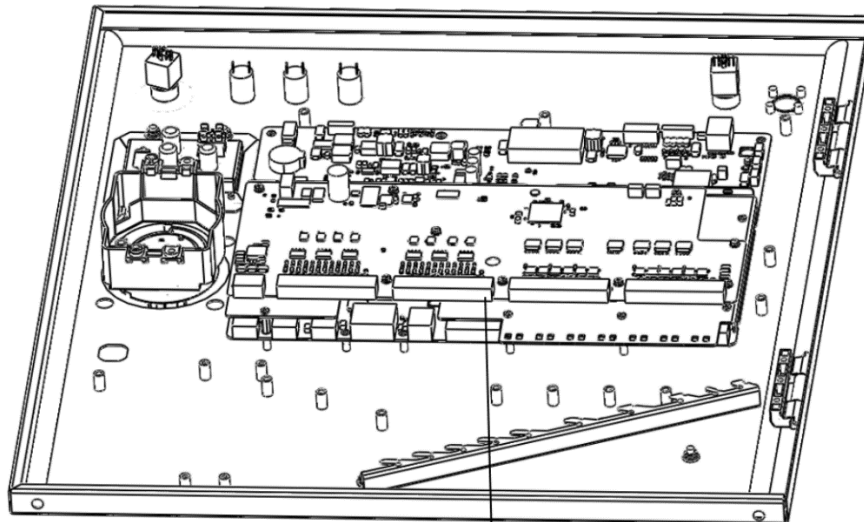
ARC5外扩48路IO模块 (NPN型)
