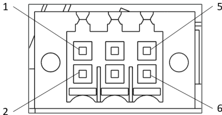
图 6-12 PLC-RS485 接口引脚标识图
