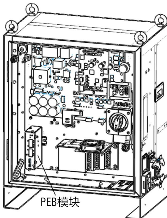
图 5-7 PEB 模块
