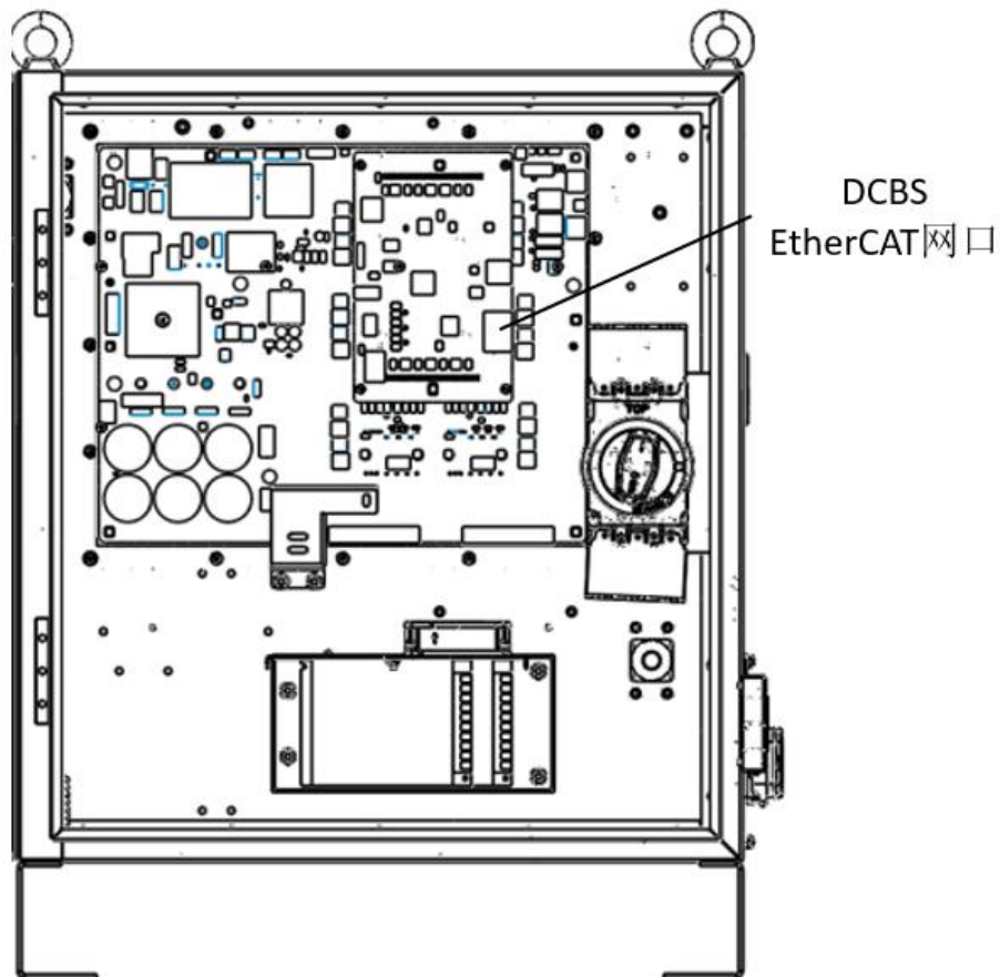
图 6-3 DCBS 接口示意图
