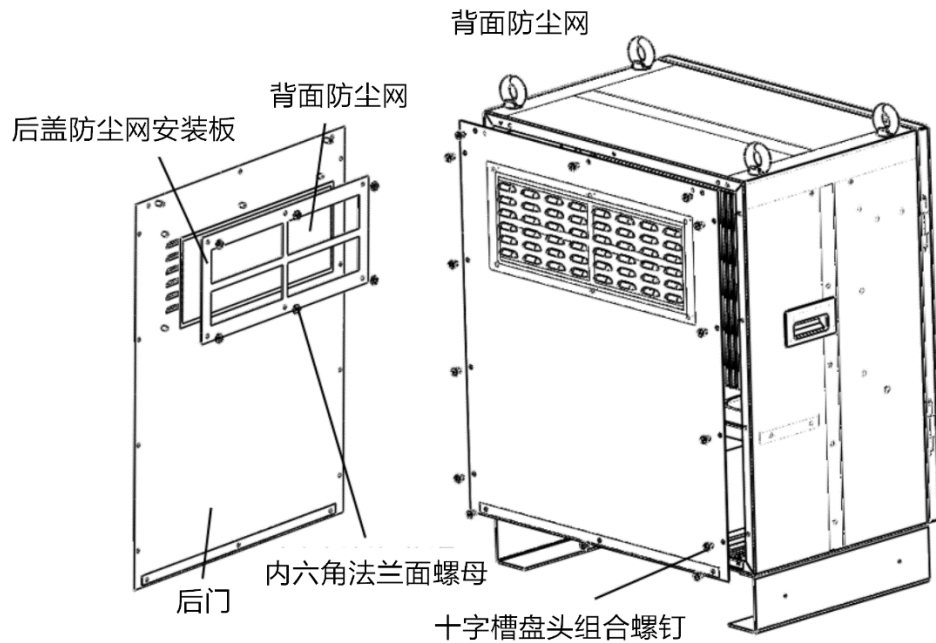
图 7-2 背面防尘网更换或清洗
