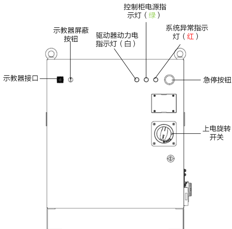
图 5-1 控制柜指示灯
