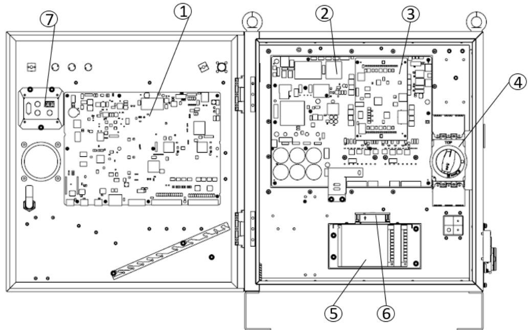
图 1-2 控制柜内部器件示意图
