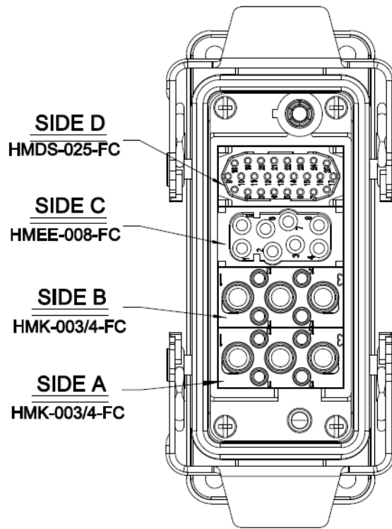
图 3-1 动力线编码器接口
