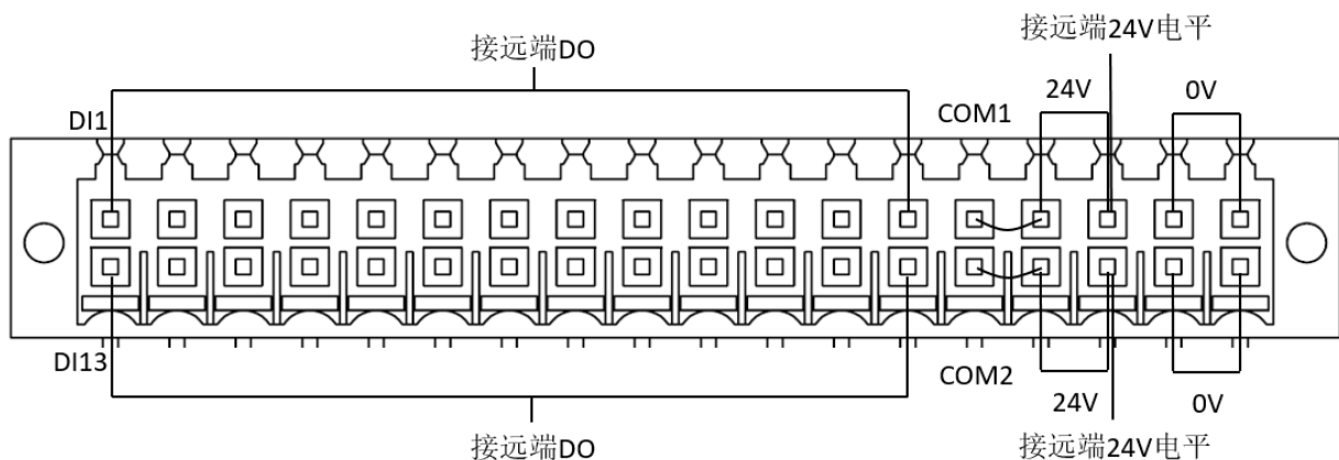
图 6-7 User DI 接口使用说明（NPN 输入）
