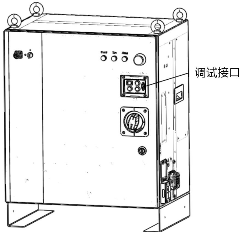
图 7-1 控制柜多轴驱动调试接口
