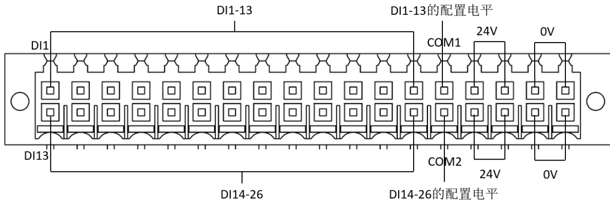
图 6-6 DI 接口和引脚标识图
