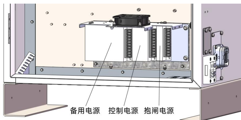
图 5-5 开关电源位置示意
