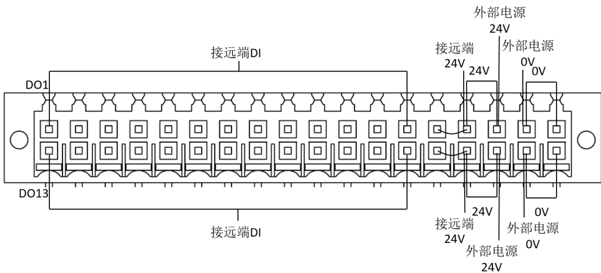
图 6-9 User DO 接口使用说明
