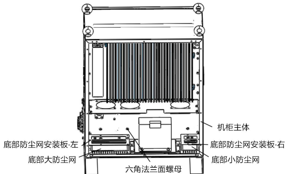
图 7-3 底部防尘网更换或清洗
