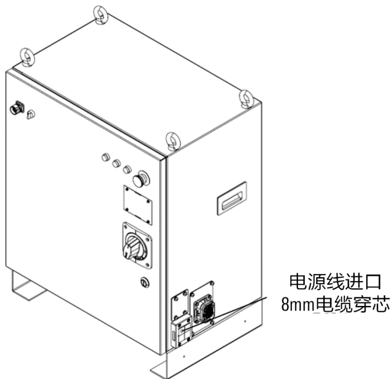
图 3-4 电源线进线示意图
