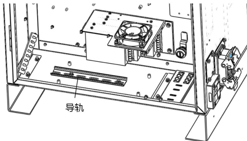
图 5-11 导轨安装
