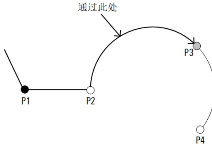
图 3-3 圆弧朝向判断程序示意图
