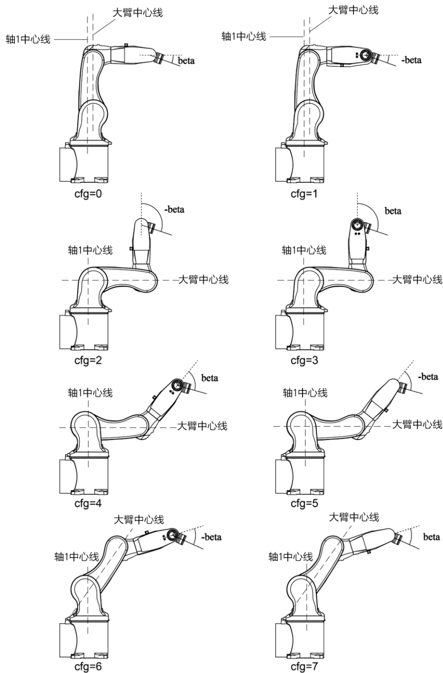
图 2-1 cfg 参数值姿态说明
