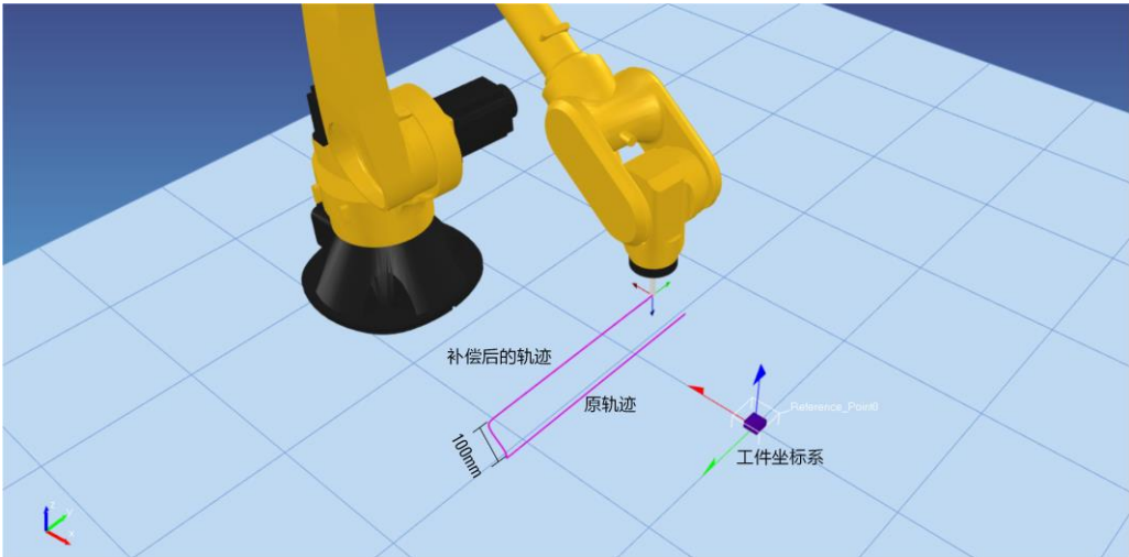
图 3-7 轨迹补偿示意图
