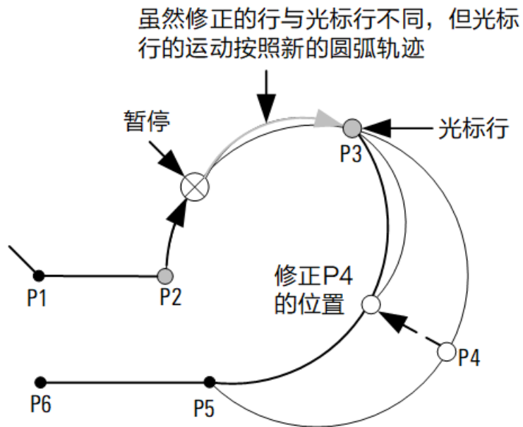
图 3-5 下一个目标点的修正示意图
