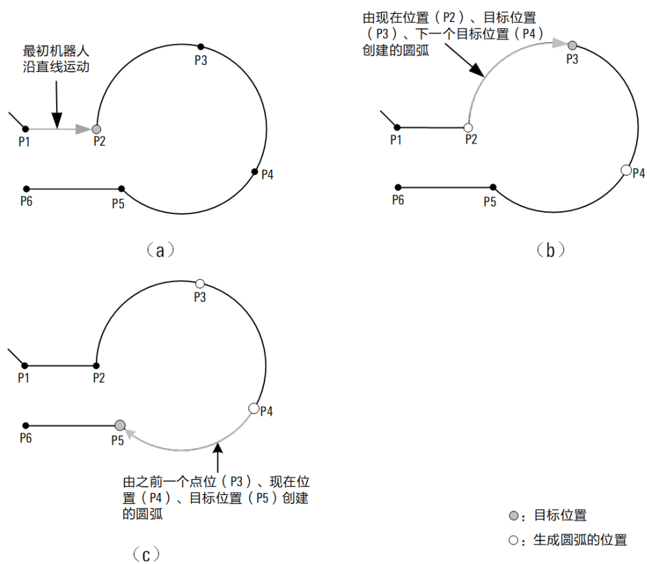
图 3-2 程序分布执行示意图
