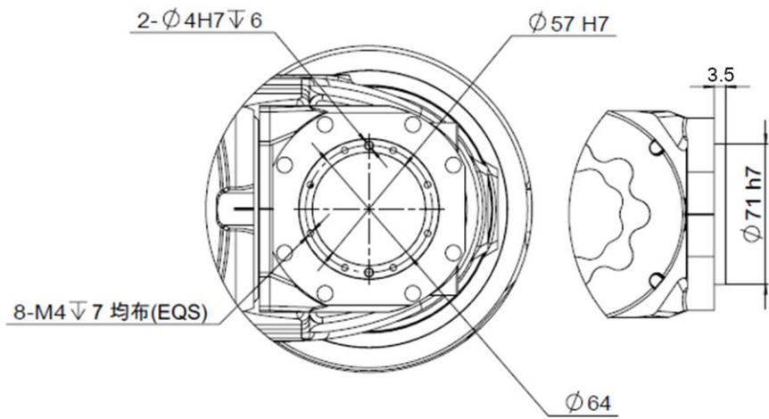
图 8-4 AIR10-1700A-HW 操作机腕部法兰尺寸示意图
