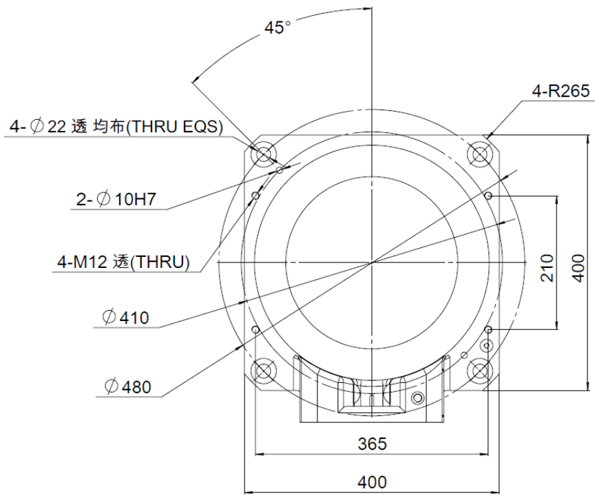
图 5-1 AIR10-1700A-HW 操作机底座接口尺寸
