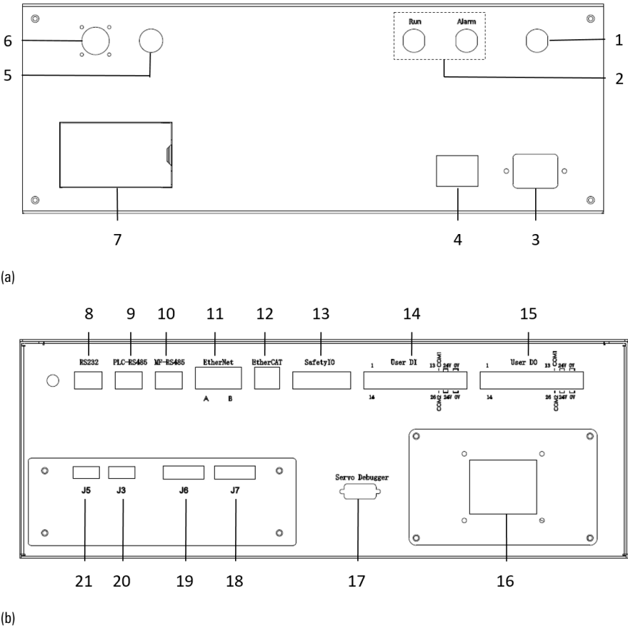
图 4-4 inCube20T 各接口所在位置示意图
