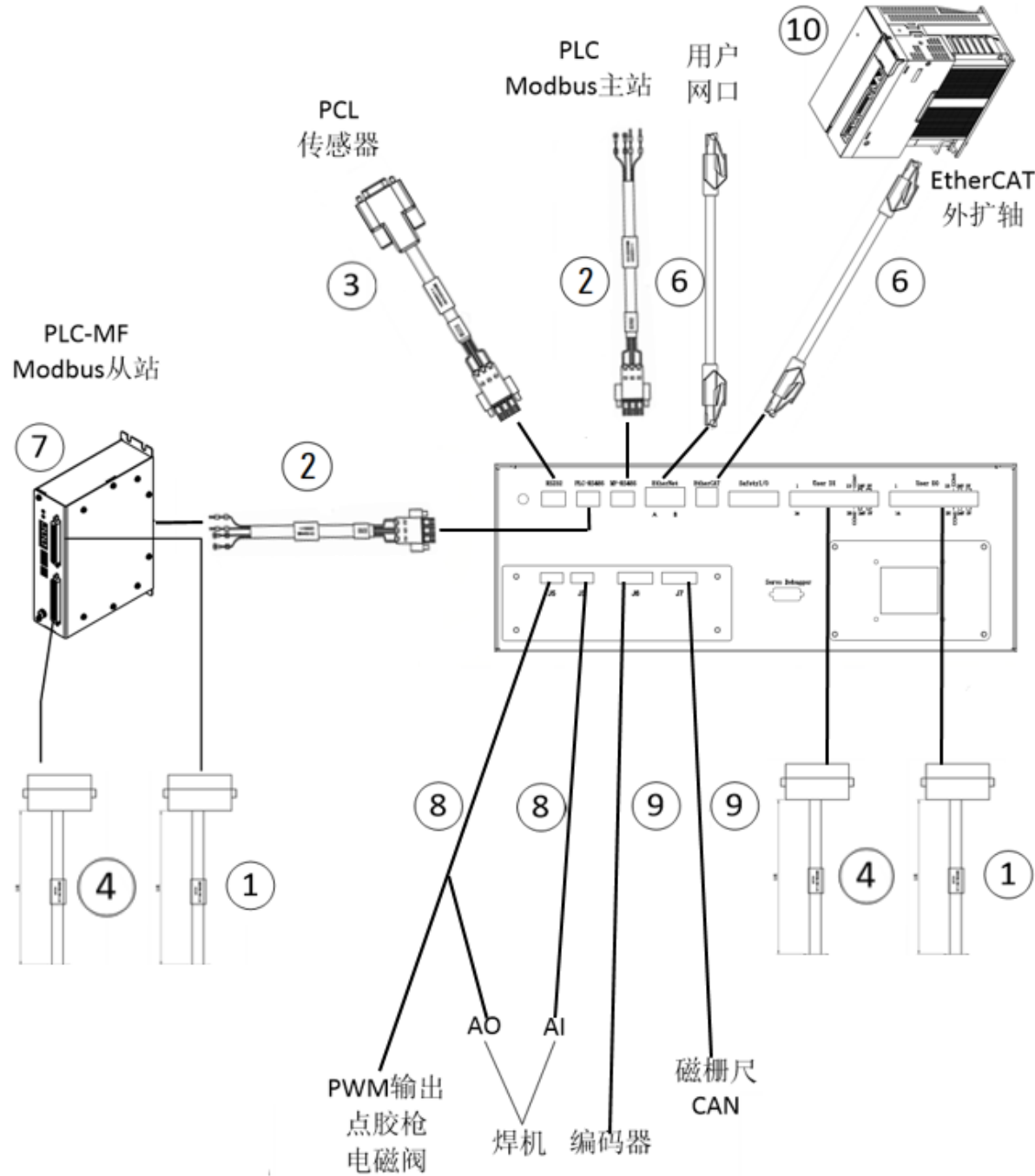
附图 1 inCube20T 控制柜配件图
