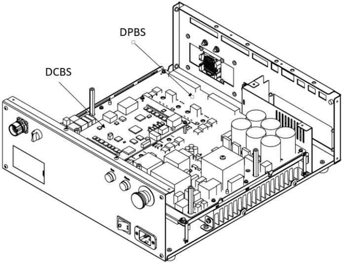
图 1-4 下腔内部器件示意图
