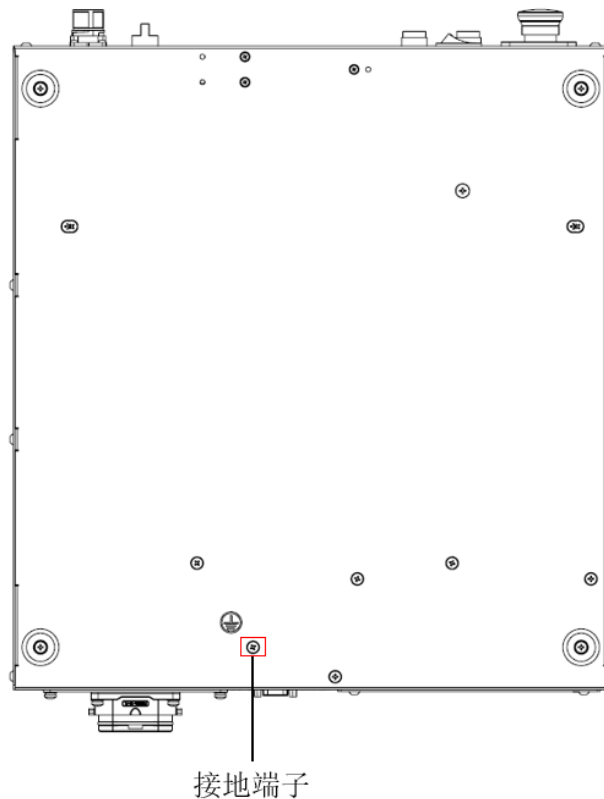
图 6-1 inCube20T 型控制柜地线接入点示意图
