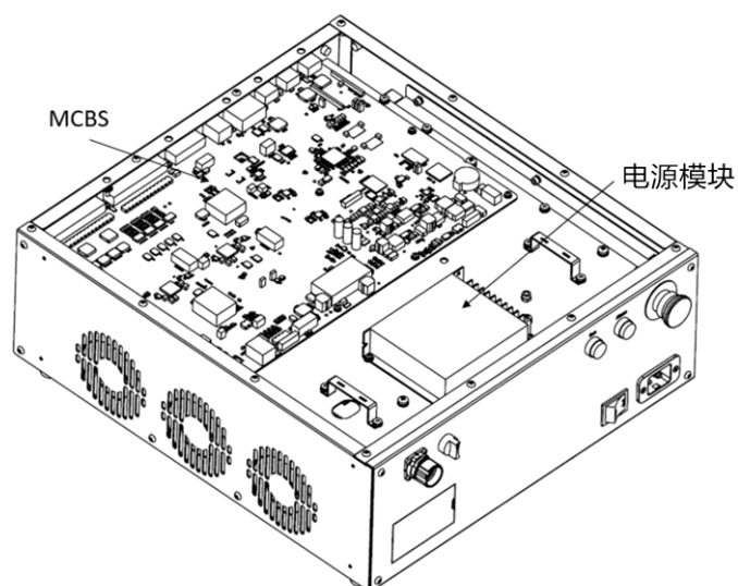
图 1-3 上腔内部器件示意图
