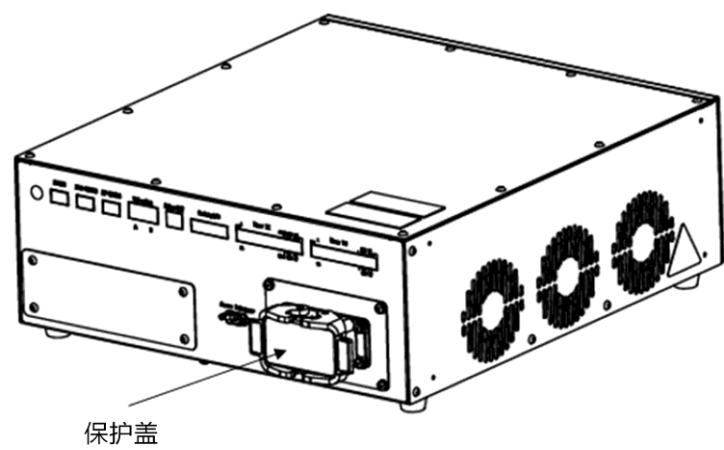
(c) 图 1-5 控制柜所含标签位置示意图
