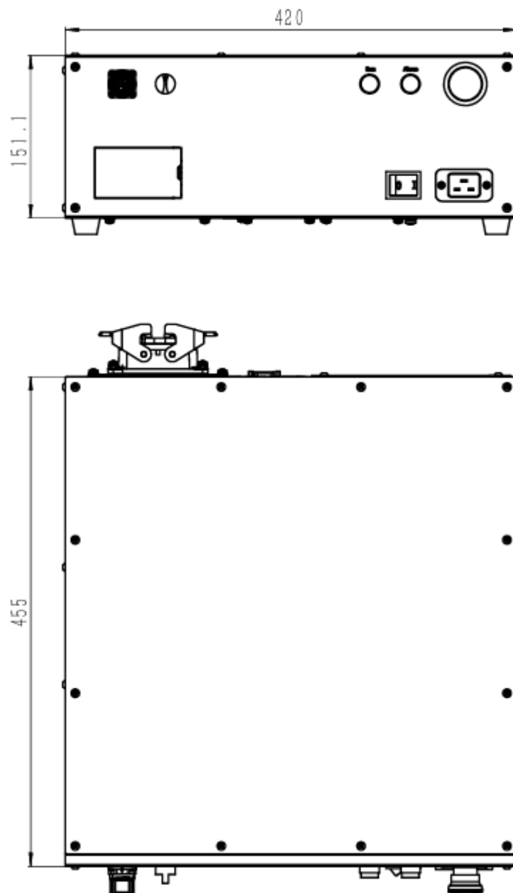
图 4-1 机柜外形尺寸图
