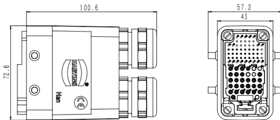
图 4-6 重载插头尺寸图
