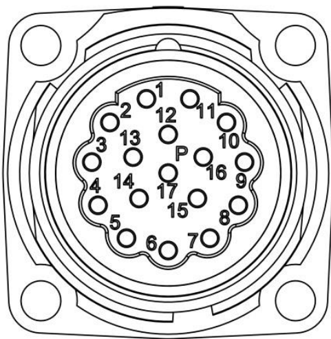
图 4-7 示教器接口
