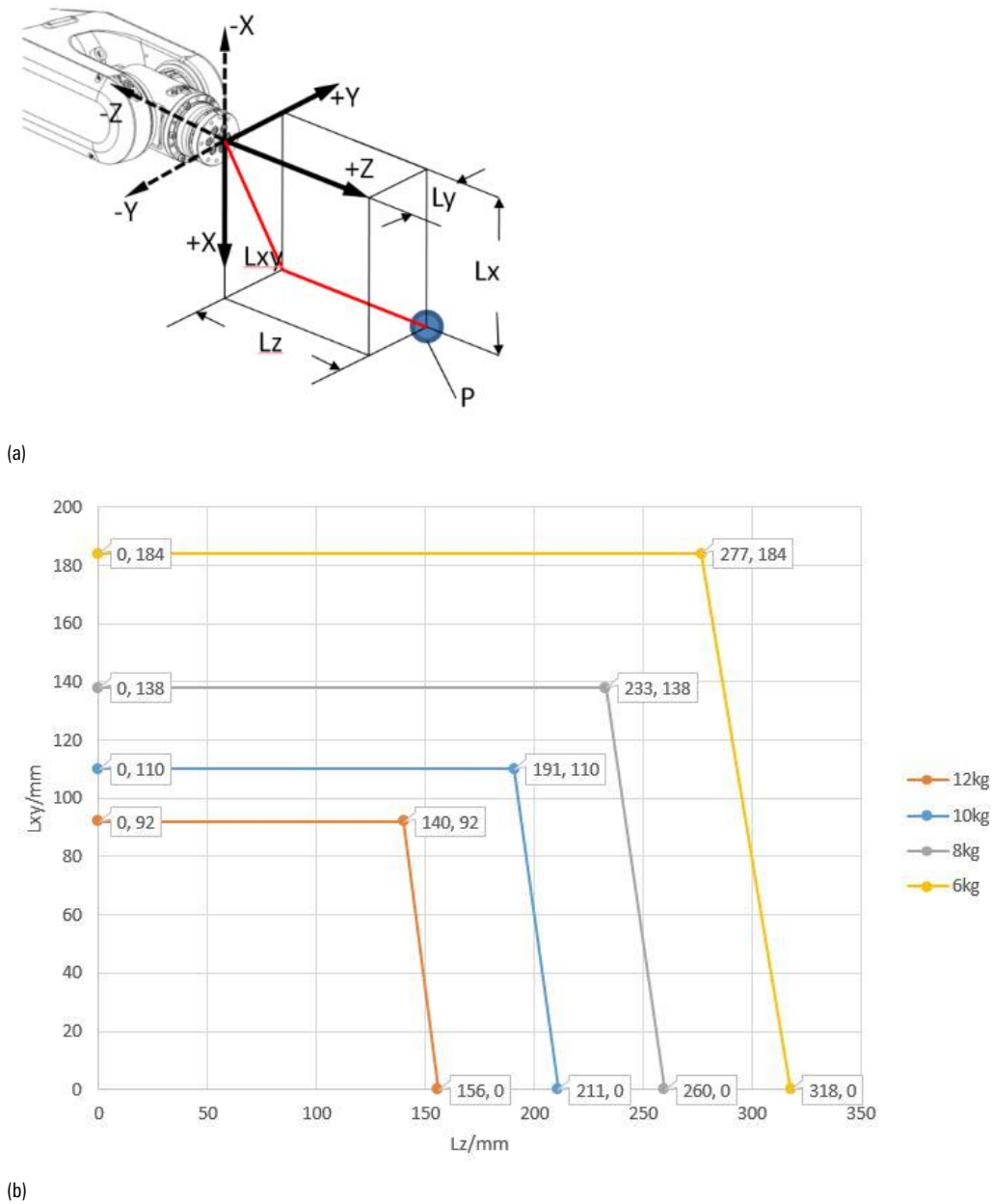
图 7-5 操作机腕部负载质心位置示意图
