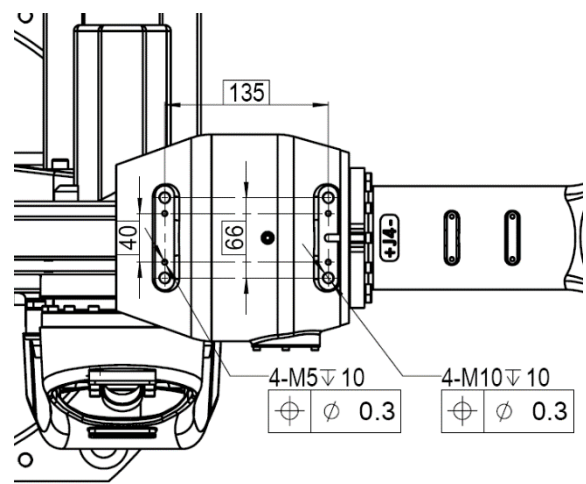
图 7-6 操作机肘部负载接口尺寸示意图
