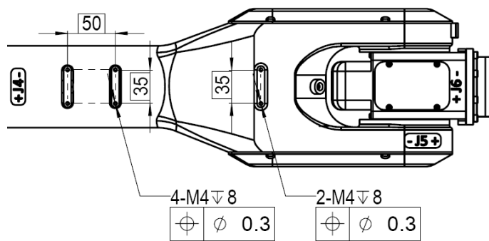
图 7-7 操作机小臂接口尺寸图
