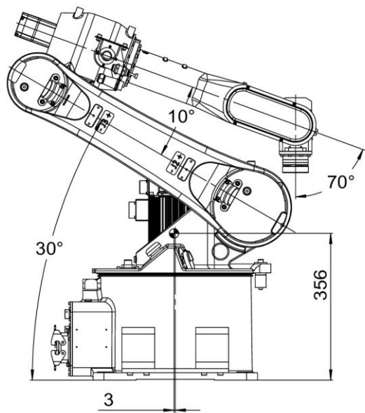
图 9-2 AIR12-1420B 操作机搬运位姿图
