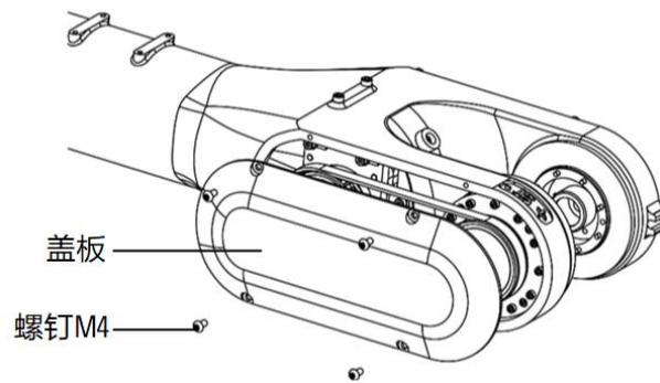
图 12-11 拆卸盖板
