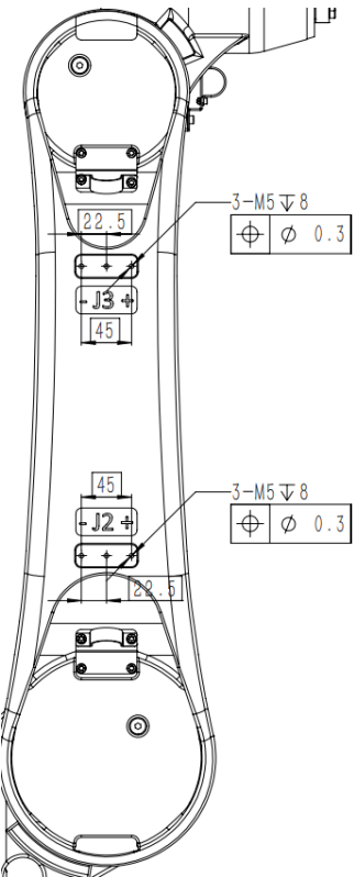
图 7-8 AIR12-1420B 大臂接口尺寸图
