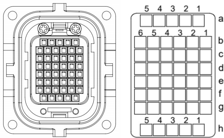
图 5-5 操作机本体重载连接器 HDD-072-MC
