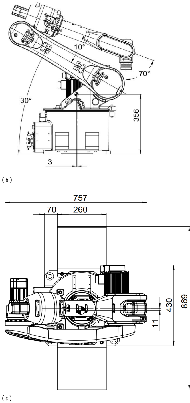
图 9-3 AIR12-1420B 搬运时操作机尺寸
