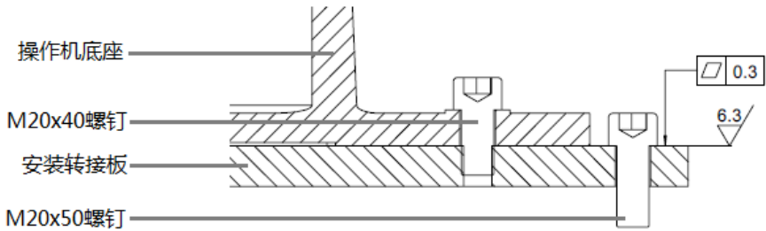
(b) 图 4-3 AIR12-1420B 操作机支架固定示意图
