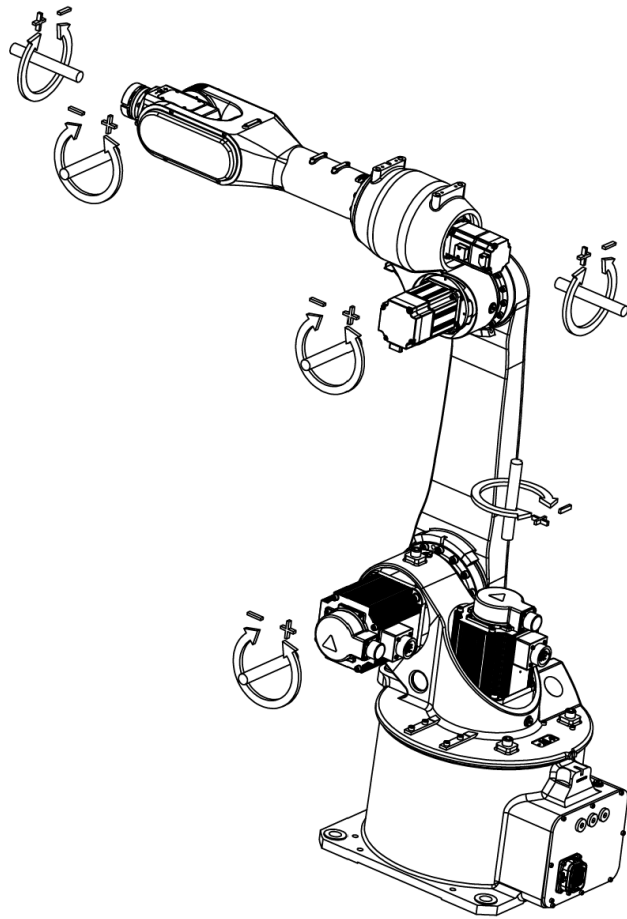
图 8-4 操作机各轴的运动方向
