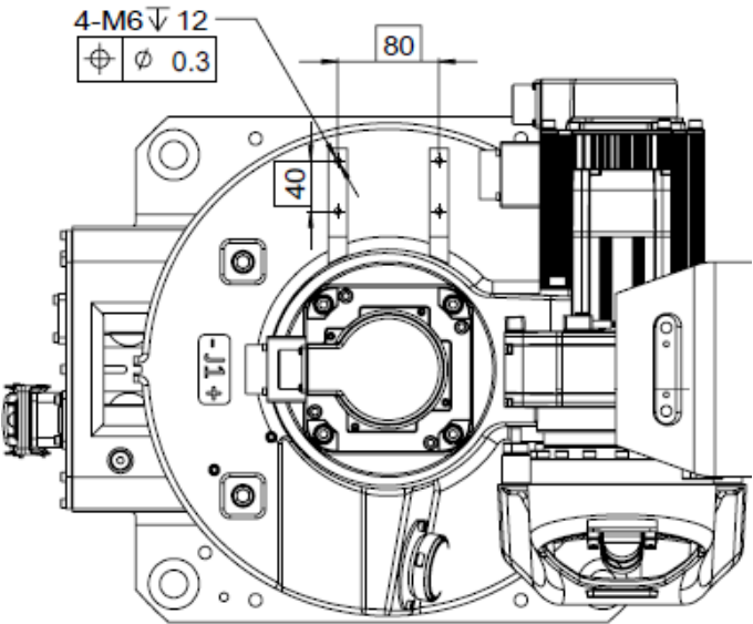
图 7-9 AIR12-1420B 肩部接口尺寸图
