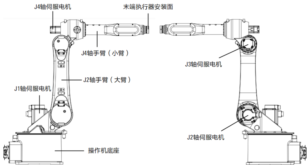
图 1-2 AIR12-1420B 机器人本体及其各个部分
