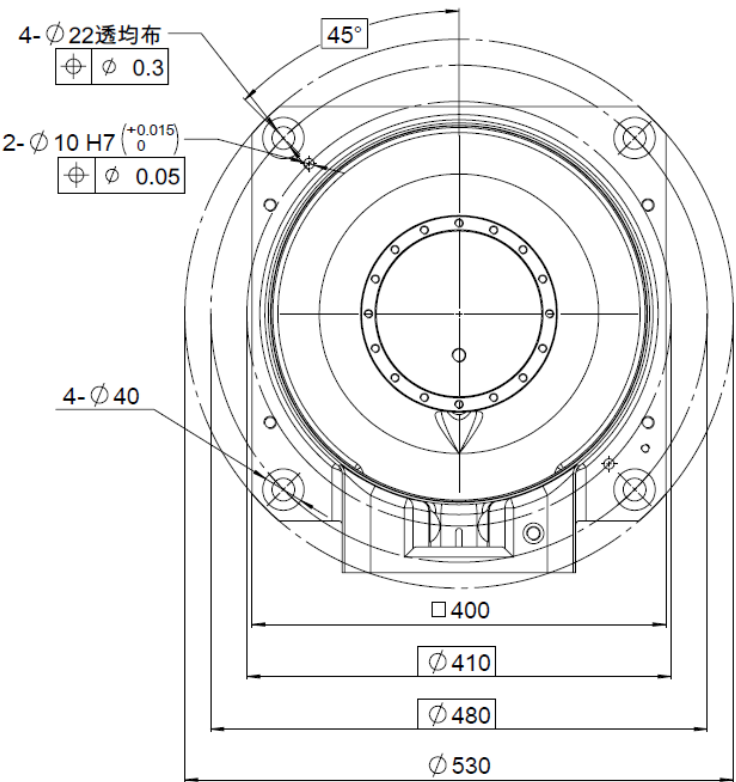
图 4-1 操作机底座接口尺寸
