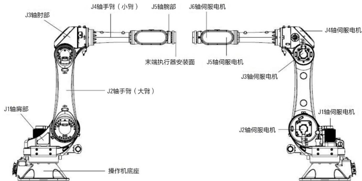
图 1-2 AIR50-2260/AIR80-2260 机器人本体及其各个部分
