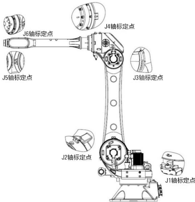
图 8-4 AIR35-2700 各轴零点示意图
