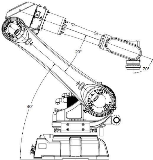
图 9-3 AIR50-2700 操作机搬运位姿图
