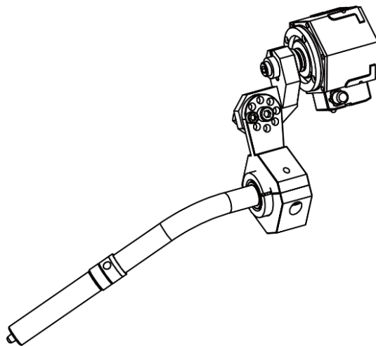
图 6-3 工业机器人用弧焊枪
