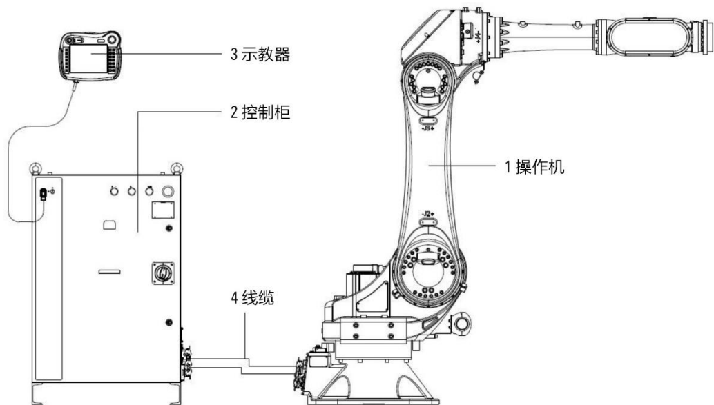
图 1-1 中负载机器人系统构成
