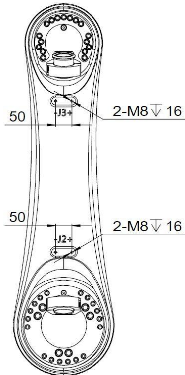
图 7-22 AIR50-2260/AIR80-2260 操作机大臂接口尺寸图
