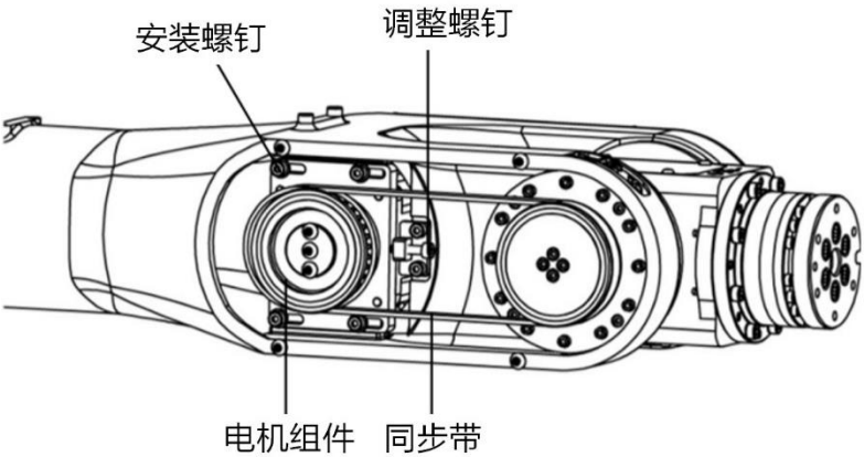
图 12-24 AIR35-2700/AIR20-3100 拆卸同步带
