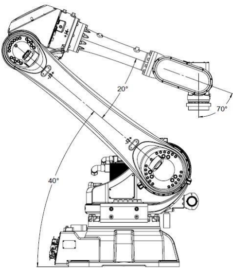
图 9-4 AIR80-2560 操作机搬运位姿图
