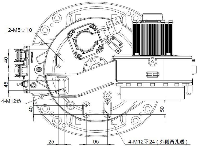
图 7-24 AIR50-2260/AIR80-2260/AIR35-2700/AIR20-3100 操作机肩部接口尺寸图
