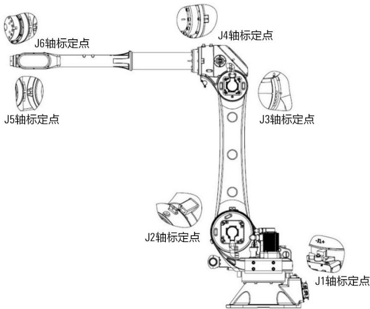
图 8-5 AIR20-3100 各轴零点示意图
