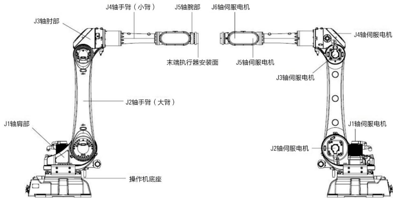
图 1-4 AIR50-2700 机器人本体及其各个部分
