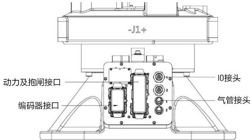
图 5-1 AIR50-2260/AIR80-2260/AIR35-2700/AIR20-3100 等操作机底座电气接口
