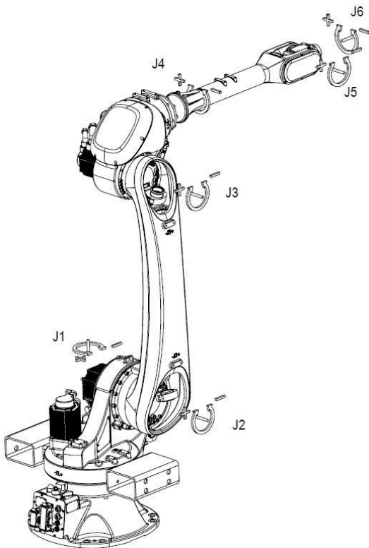
图 7-3 AIR35-2700/AIR20-3100 操作机各轴运动方向
