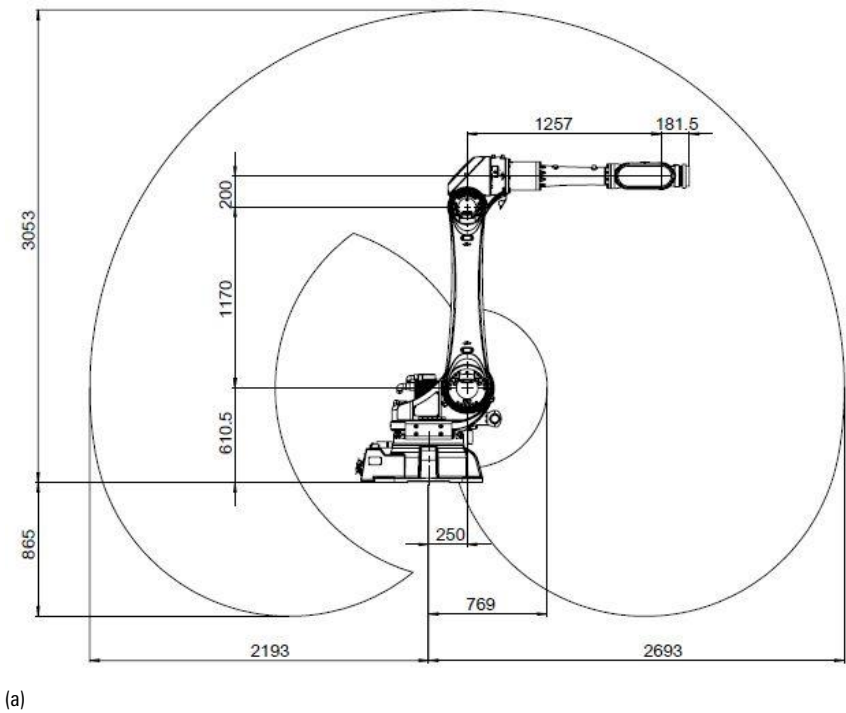
图 7-5 AIR80-2560 操作机工作范围
