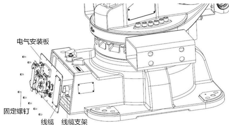
图 12-5 AIR50-2700/AIR80-2560 底座内部线缆
