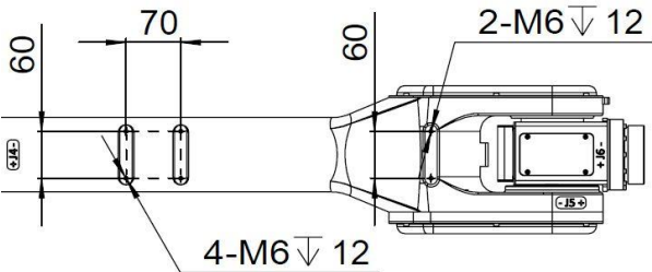
图 7-21 AIRAIR35-2700/AIR20-3100 操作机小臂接口尺寸图
