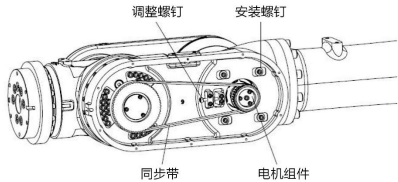
图 12-22 AIR80-2260/AIR80-2560 拆卸同步带
