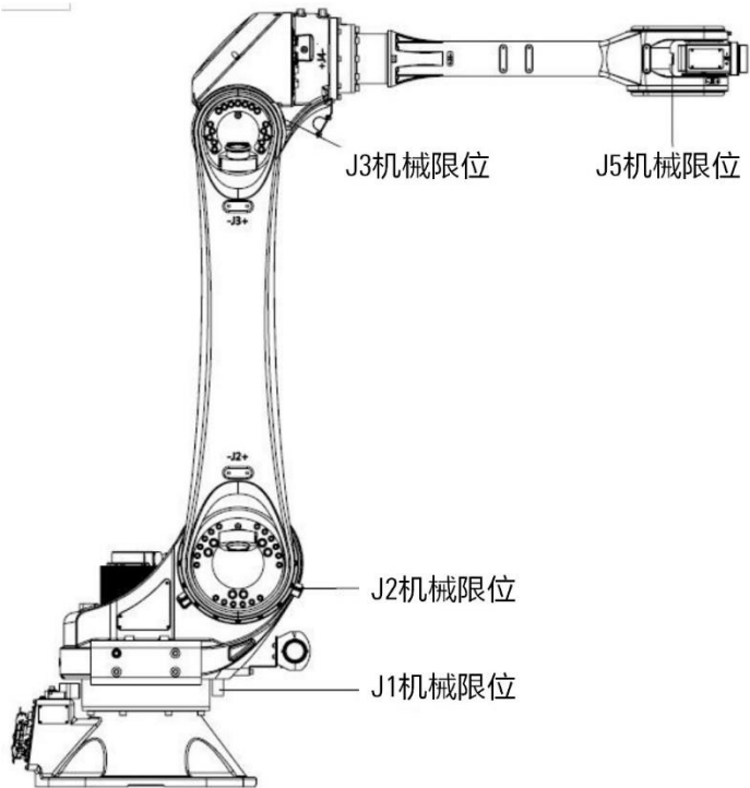
图 7-11 AIR35-2700/AIR20-3100 操作机上机械式制动器
