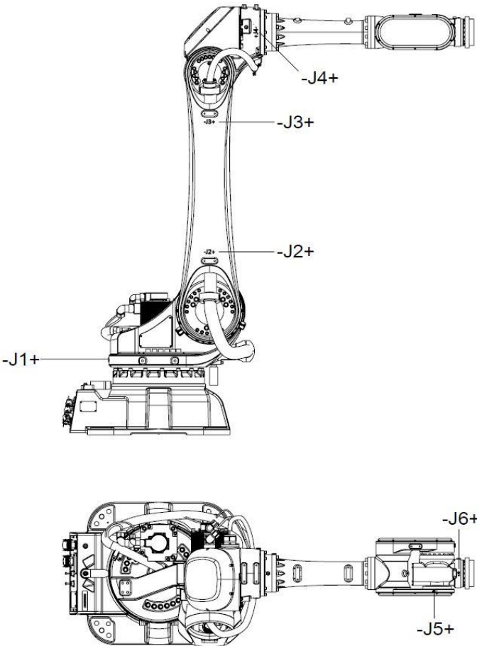
图 2-4 AIR80-2560 操作机上各轴方向标识
