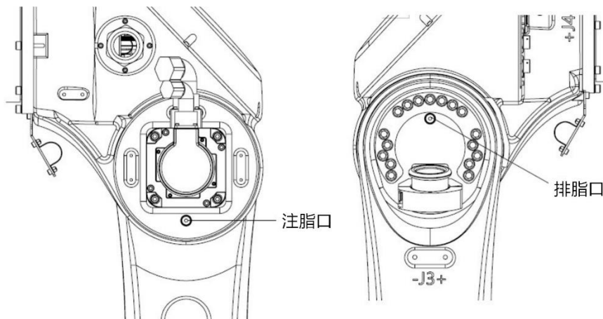
图 12-14 更换 J3 轴减速器润滑脂
