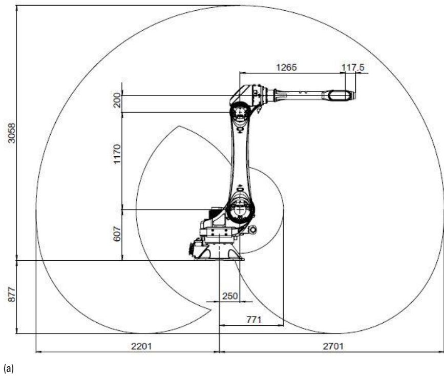
图 7-6 AIR50-2700 操作机工作范围
