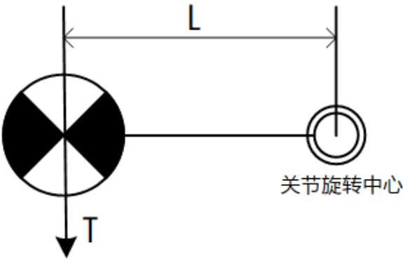
图 7-14 负载离心率示意图
