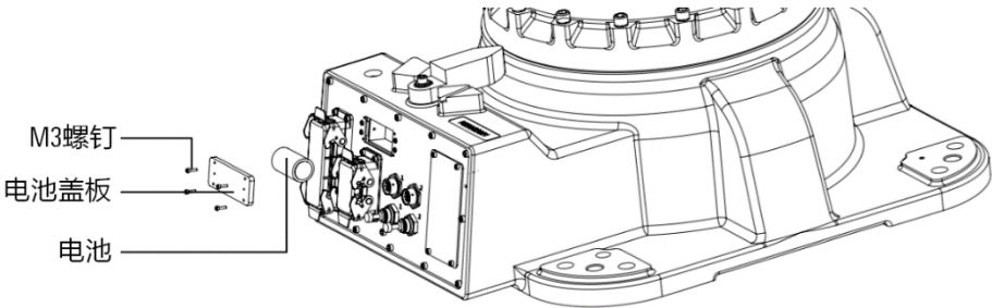
图 12-10 AIR50-2700/AIR80-2560 更换电池
