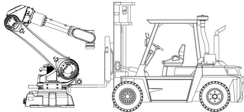
图 9-13 AIR50-2700/AIR80-2560 叉车搬运示意图
