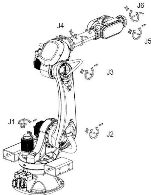
图 7-1 AIR50-2260/AIR80-2260 操作机各轴运动方向
