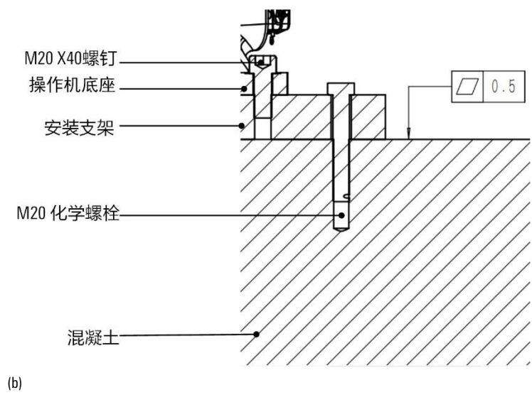
图 4-4 操作机支架固定示意图
