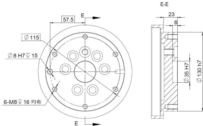
图 7-12 AIR50-2260/AIR80-2260/AIR50-2700/AIR80-2560 操作机腕部法兰尺寸示意图
