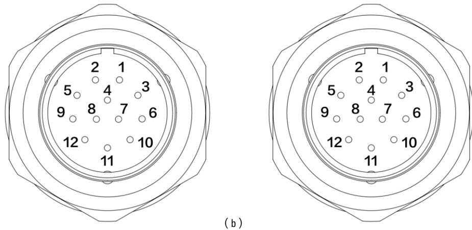
图 5-6 中负载操作机底座 I/O 航插接口 (左) 及小臂 I/O 航插接口 (右)
