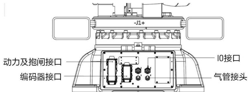
图 5-2 AIR50-2700/AIR80-2560 操作机底座电气接口
