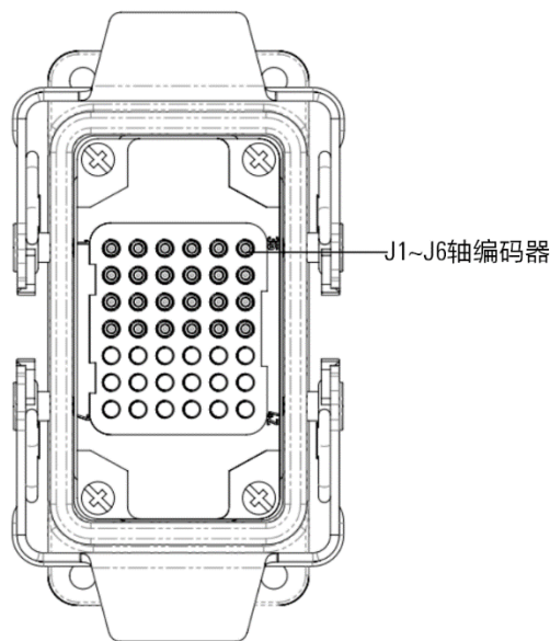
图 5-5 中负载操作机编码器线重载连接器
