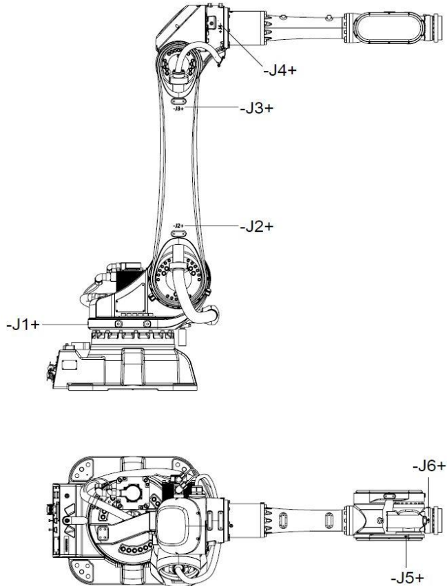
图 2-5 AIR50-2700 操作机上各轴方向标识
