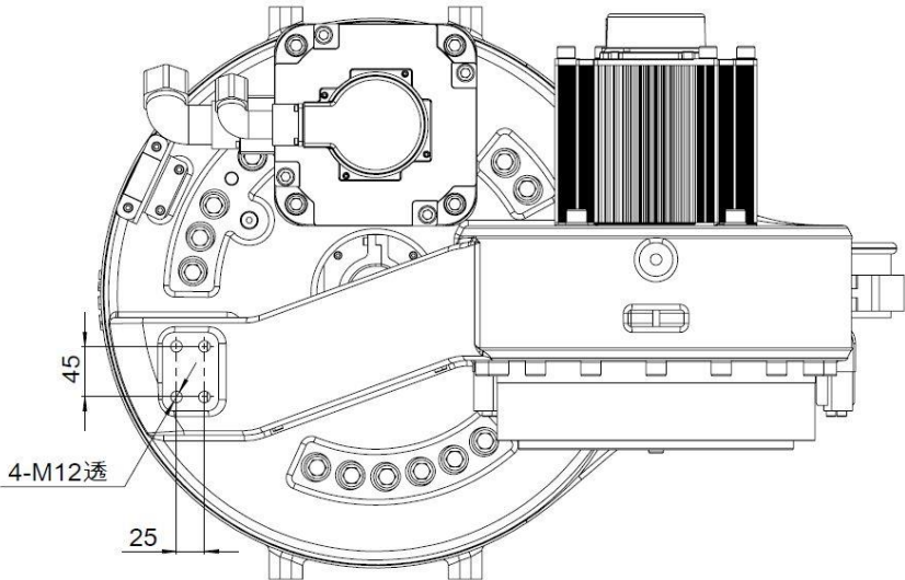
图 7-25 AIR50-2700/AIR80-2560 操作机肩部接口尺寸图
