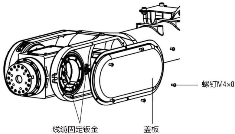
图 12-8 AIR35-2700/AIR20-3100 腕部内部线缆
