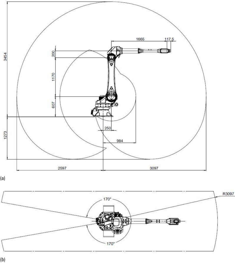
图 7-8 AIR20-3100 操作机工作范围
