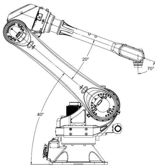
图 9-5 AIR35-2700 操作机搬运位姿图
