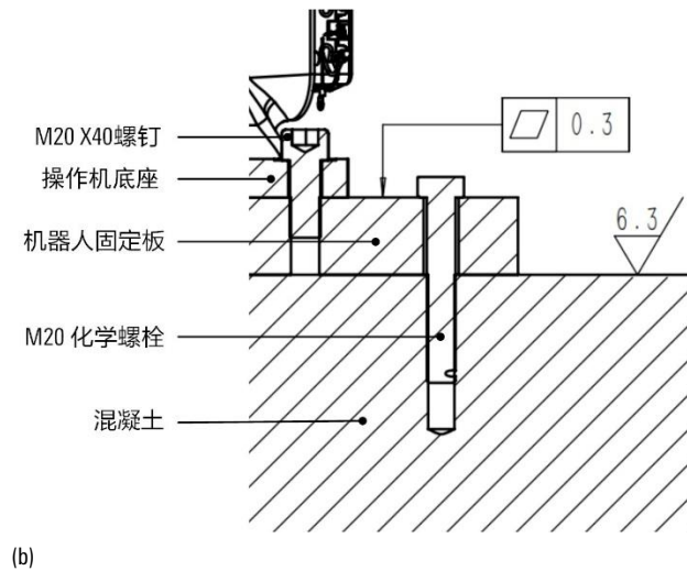
图 4-3 操作机地面固定示意图
