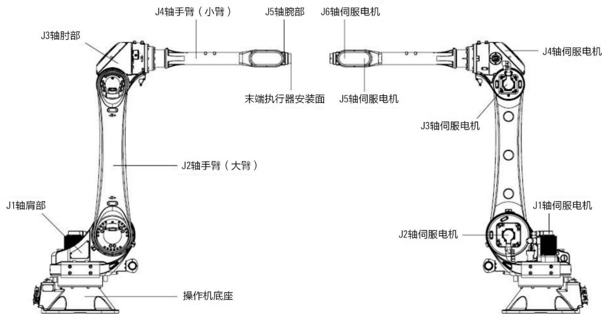
图 1-5 AIR35-2700 机器人本体及其各个部分
