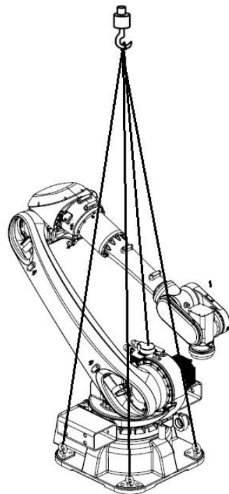
图 9-15 AIR50-2700/AIR80-2560 吊环搬运示意图
