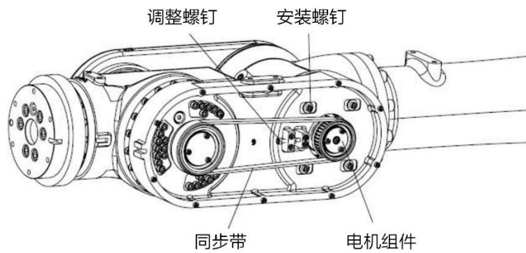
图 12-20 AIR50-2260/AIR50-2700 拆卸同步带
