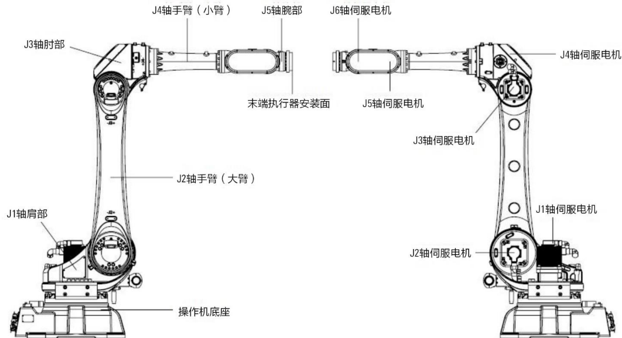
图 1-3 AIR80-2560 机器人本体及其各个部分
