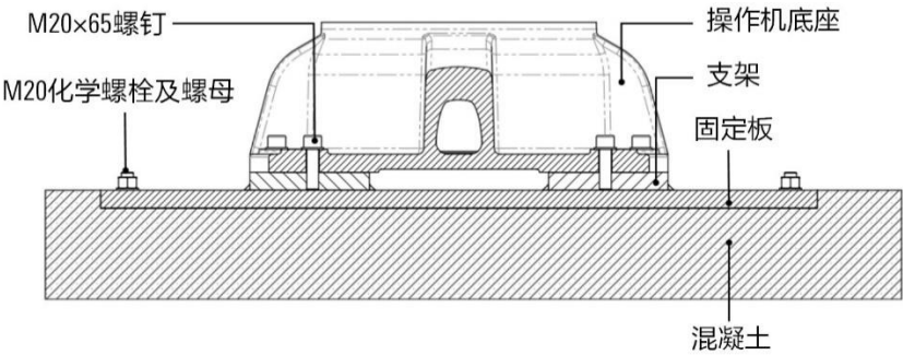
(b) 支架固定剖面图
