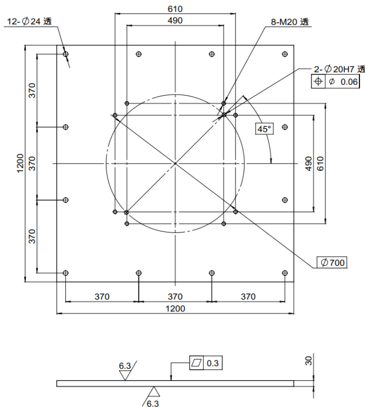
(a) 固定板尺寸
