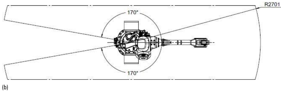
图 7-7 AIR35-2700 操作机工作范围
