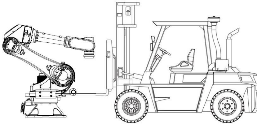
图 9-12 AIR50-2260/AIR80-2260/AIR35-2700/AIR20-3100 叉车搬运示意图
