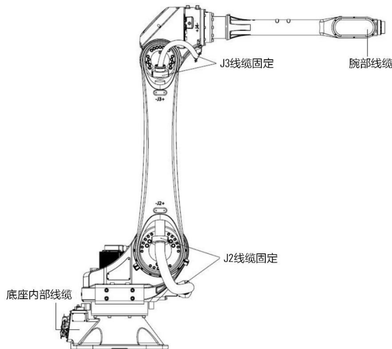
图 12-3 AIR35-2700/AIR20-3100 操作机线缆布局示意图
