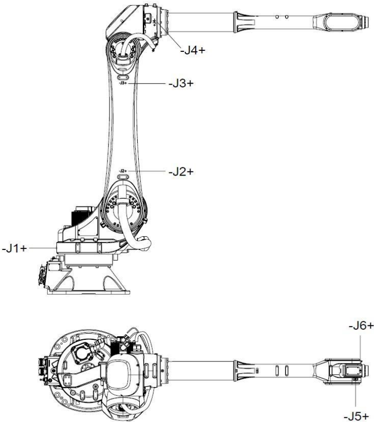
图 2-7 AIR20-3100 操作机上各轴方向标识
