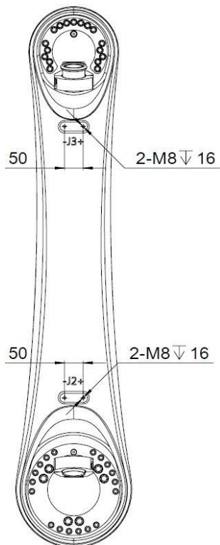
图 7-23 AIR80-2560/AIR50-2700/AIR35-2700/AIR20-3100 操作机大臂接口尺寸图
