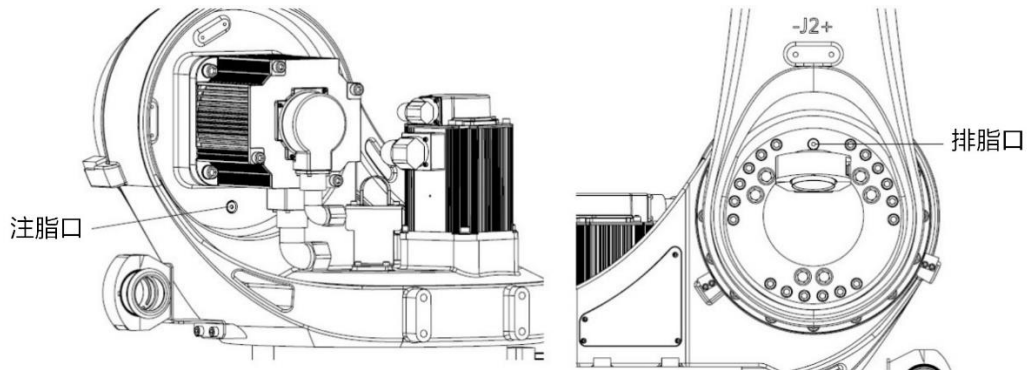
图 12-13 更换 J2 轴减速器润滑脂
