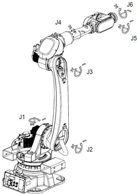
图 7-2 AIR50-2700/AIR80-2560 操作机各轴运动方向
