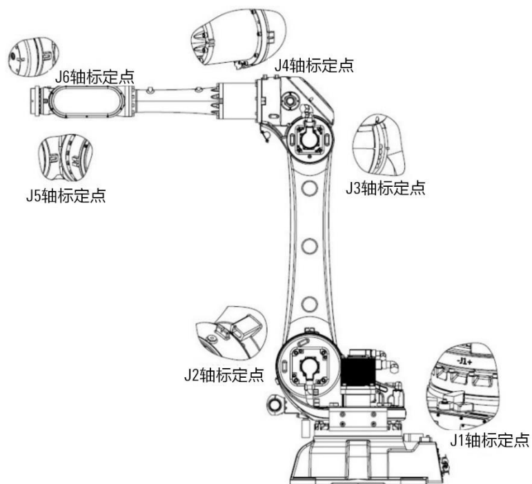
图 8-2 AIR50-2700 各轴零点示意图
