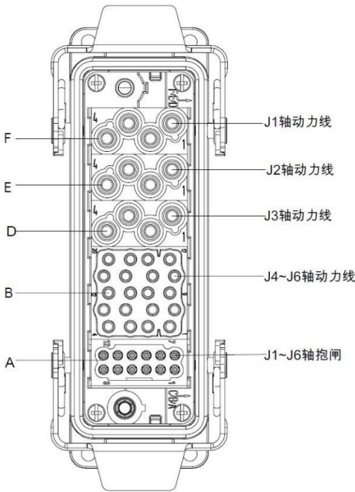
图 5-4 中负载操作机动力重载连接器
