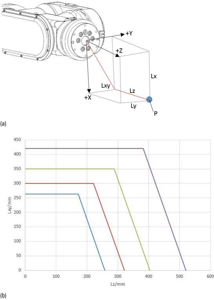
图 7-16 AIR80-2260/AIR80-2560 腕部负载质心位置示意图
