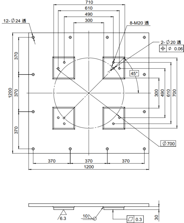
(a) 支架固定平面布置尺寸
