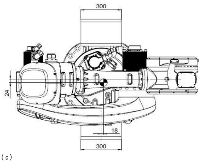
图 9-7 AIR50-2260/AIR80-2260 搬运时操作机尺寸
