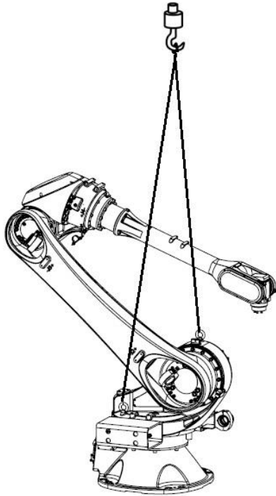
图 9-14 AIR50-2260/AIR80-2260/AIR35-2700/AIR20-3100 吊环搬运示意图
