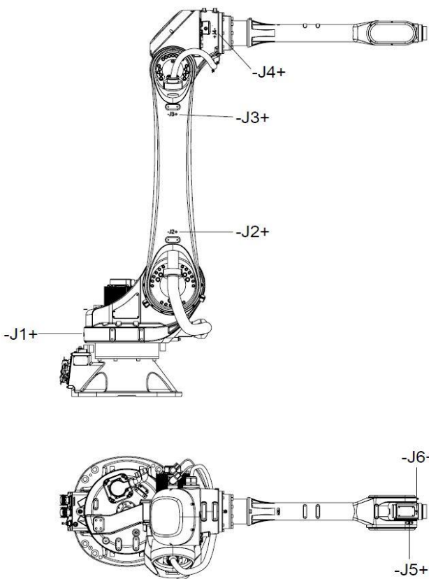
图 2-6 AIR35-2700 操作机上各轴方向标识
