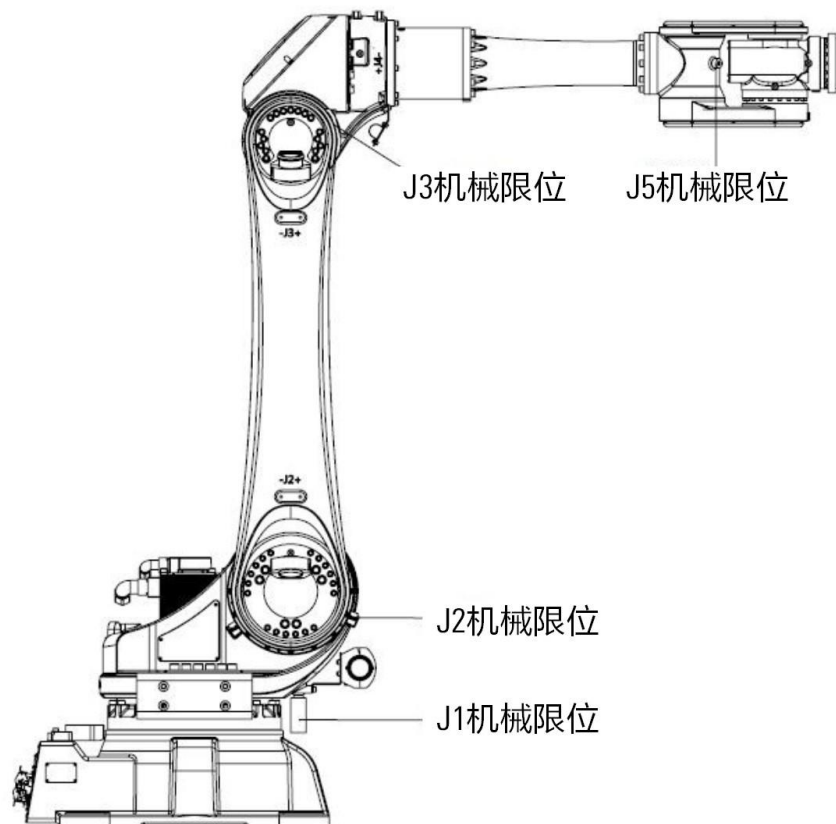
图 7-10 AIR50-2700/AIR80-2560 操作机上机械式制动器
