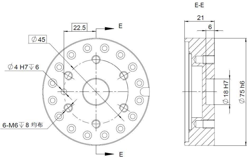
图 7-13 AIR35-2700/AIR20-3100 操作机腕部法兰尺寸示意图
