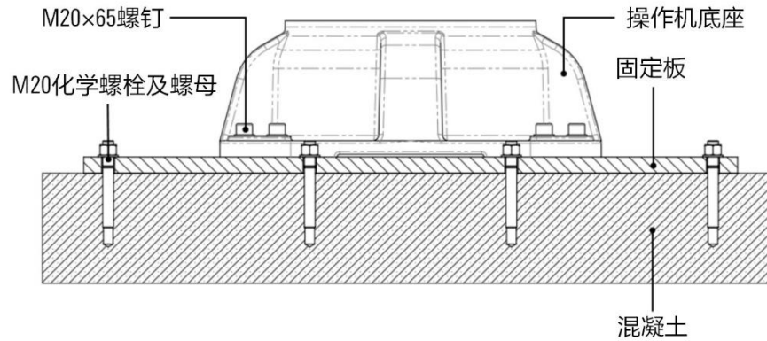
(b) 地面固定剖面图
