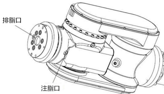
图 12-18 更换 J6 轴减速器润滑脂
