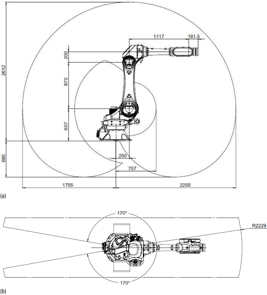
图 7-4 AIR50-2260/AIR80-2260 操作机工作范围
