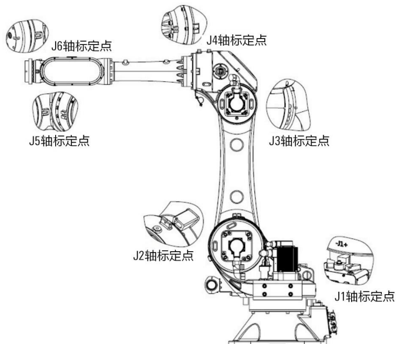
图 8-1 AIR50-2260/AIR80-2260 各轴零点示意图
