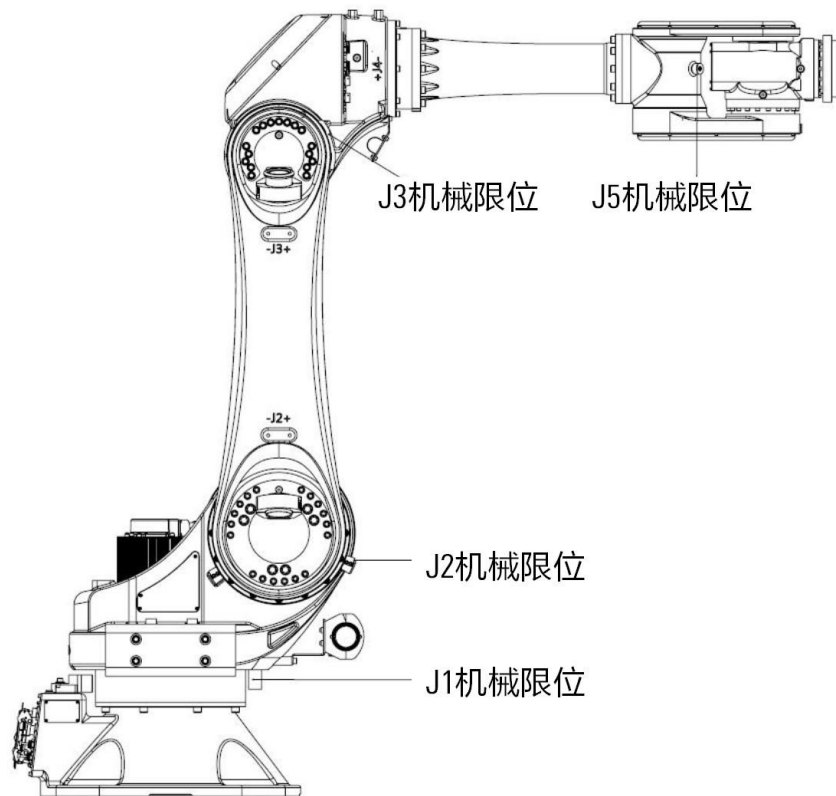
图 7-9 AIR50-2260/AIR80-2260 操作机上机械式制动器
