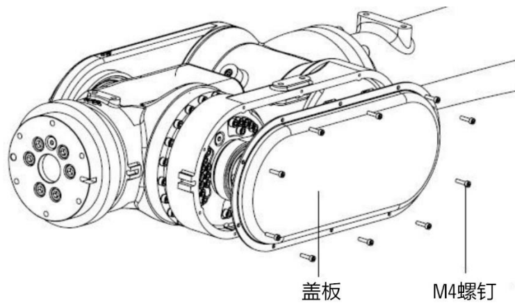
图 12-19 AIR50-2260/AIR50-2700 拆卸盖板
