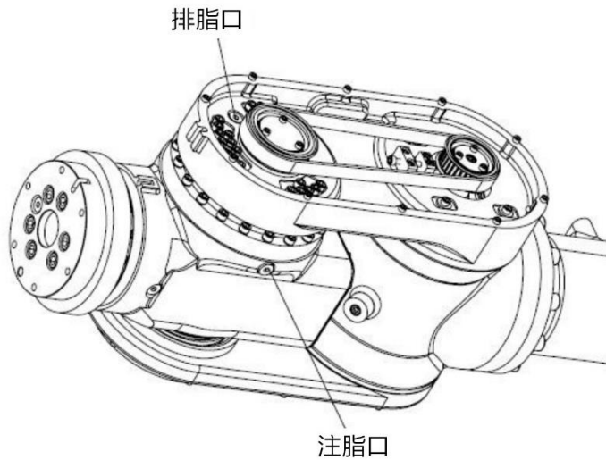
图 12-17 更换 J5 轴减速器润滑脂
