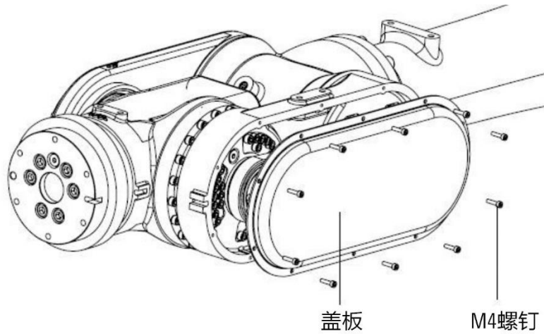
图 12-16 拆卸 J5 轴盖板
