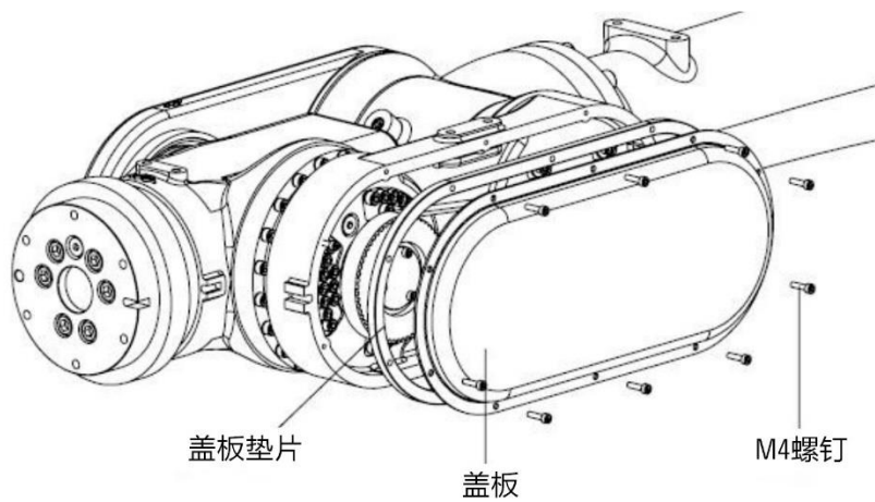
图 12-21 AIR80-2260/AIR80-2560 拆卸盖板
