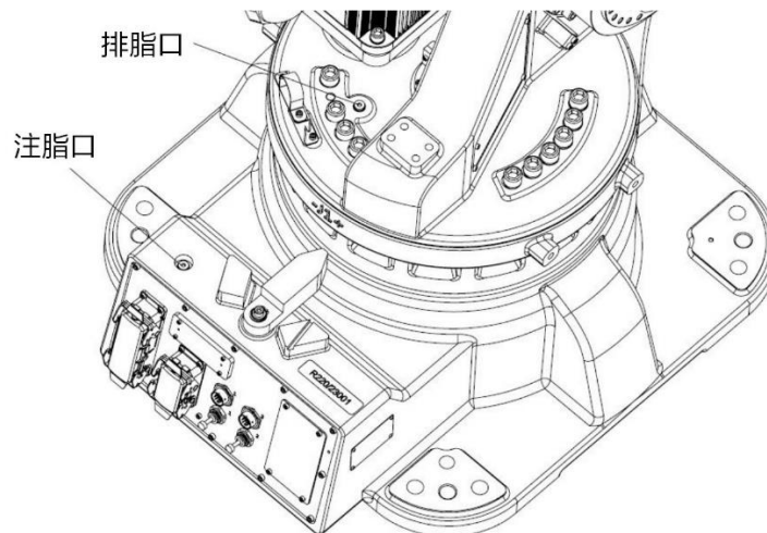
图 12-12 AIR50-2700/AIR80-2560 更换 J1 轴减速器润滑脂
