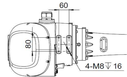
图 7-19 操作机肘部负载接口尺寸示意图
