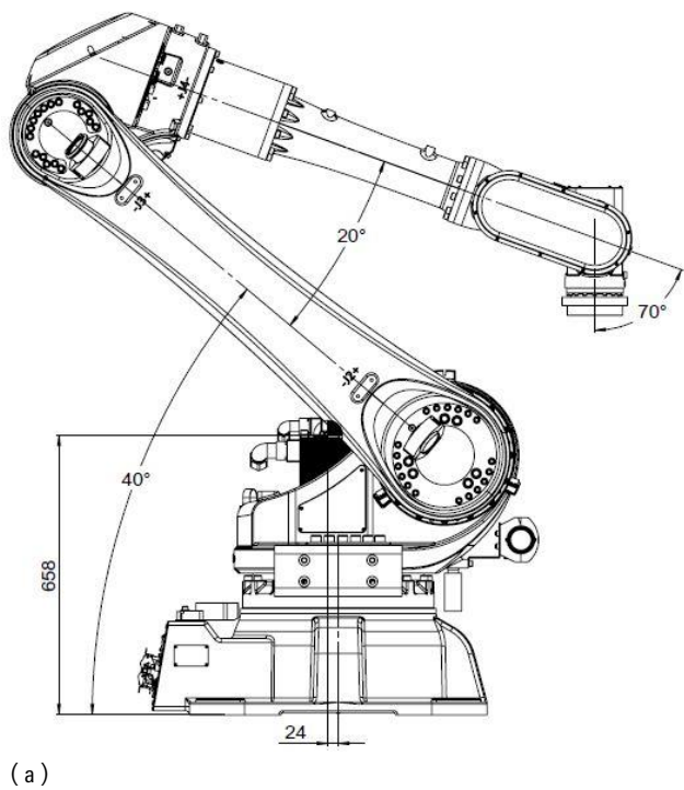
图 9-7 AIR50-2260/AIR80-2260 搬运时操作机尺寸
