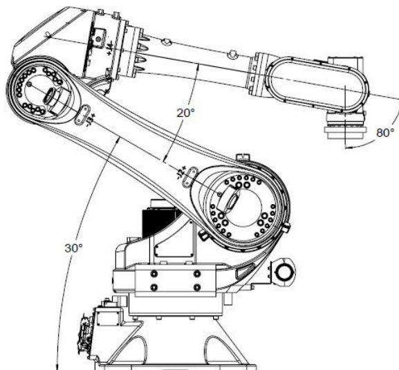
图 9-2 AIR50-2260/AIR80-2260 操作机搬运位姿图
