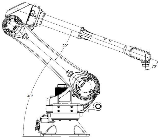
图 9-6 AIR20-3100 操作机搬运位姿图
