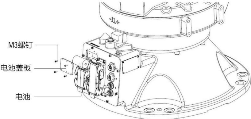
图 12-9 AIR50-2260/AIR80-2260/AIR35-2700/AIR20-3100 更换电池
