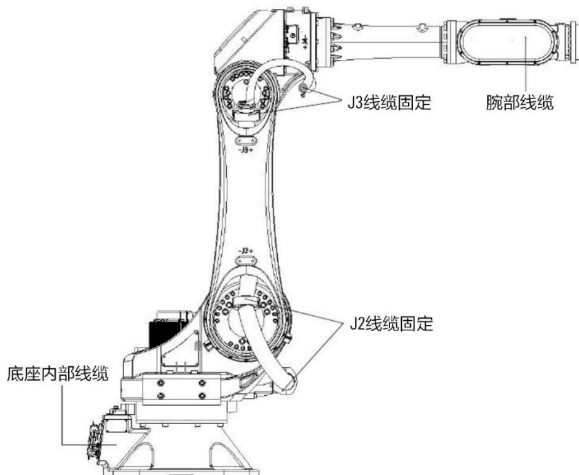
图 12-1 AIR50-2260/AIR80-2260 操作机线缆布局示意图
