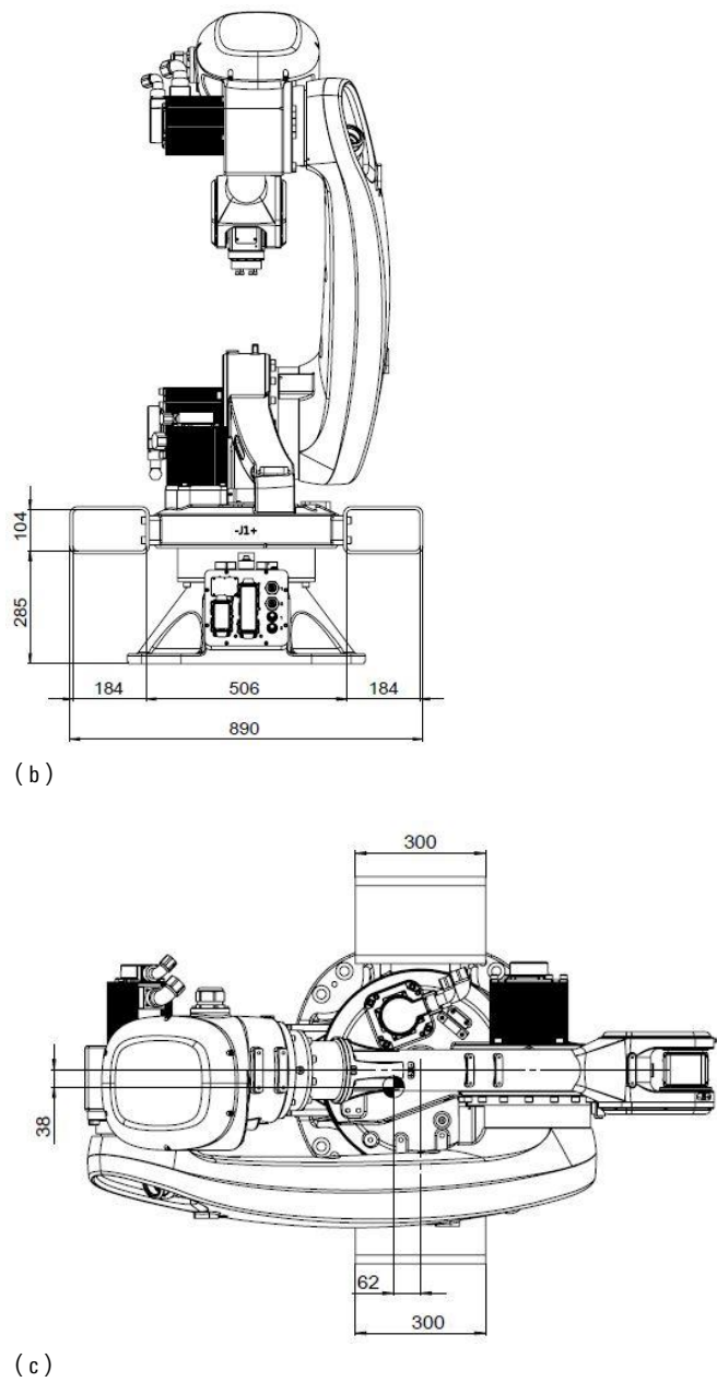
图 9-10 AIR35-2700 搬运时操作机尺寸
