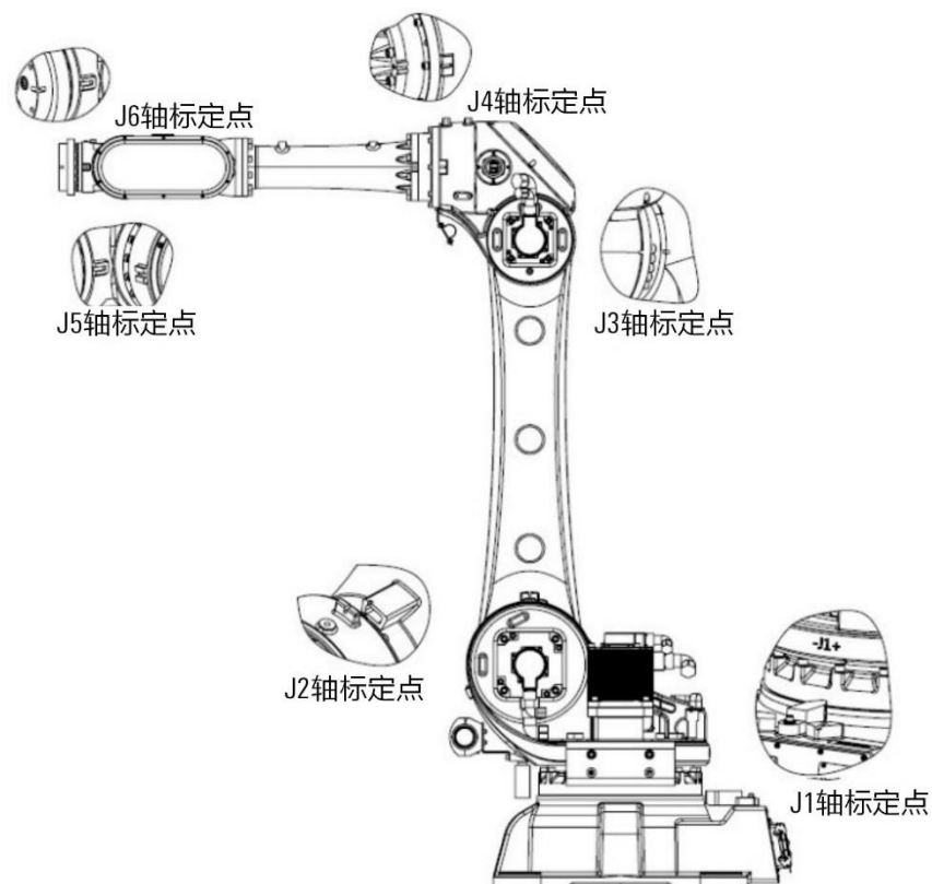
图 8-3 AIR80-2560 各轴零点示意图
