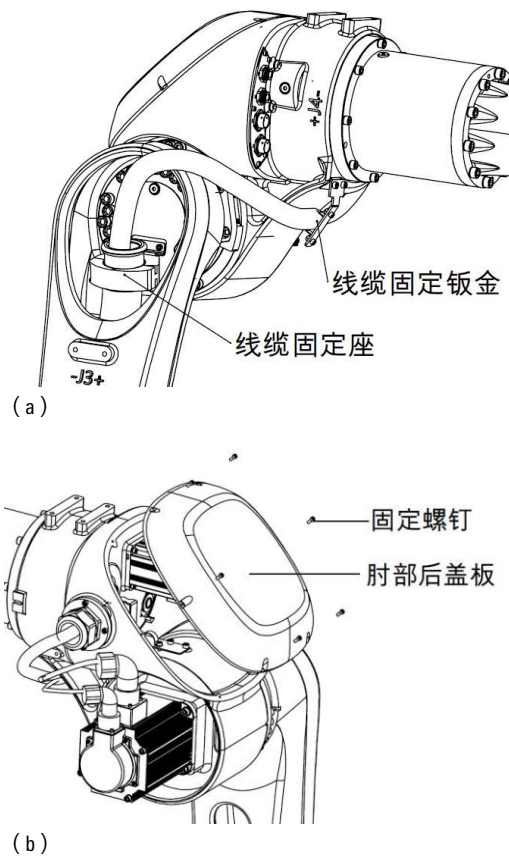
图 12-6 肘部内部线缆
