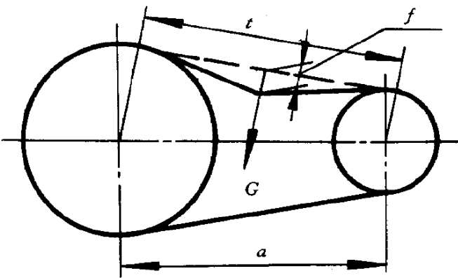
图 12-25 同步带安装挠度
