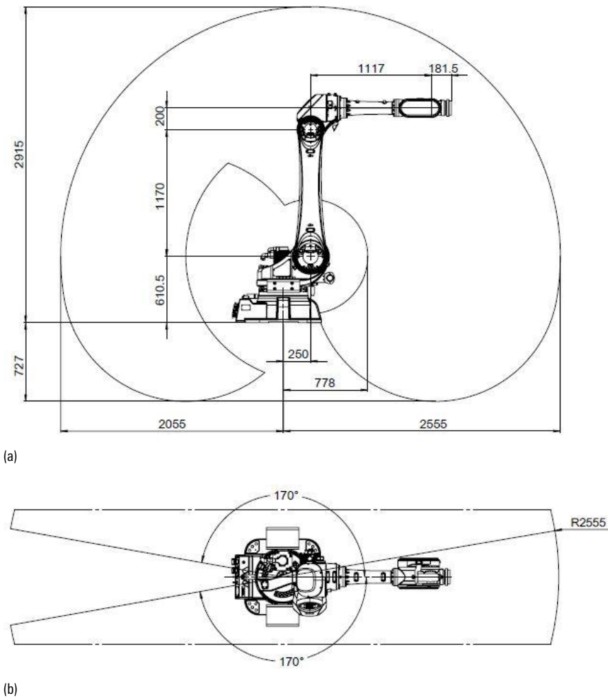
图 7-5 AIR80-2560 操作机工作范围
