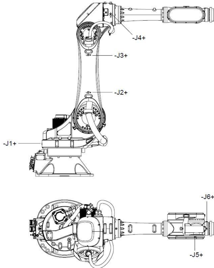
图 2-3 AIR50-2260/AIR80-2260 操作机上各轴方向标识
