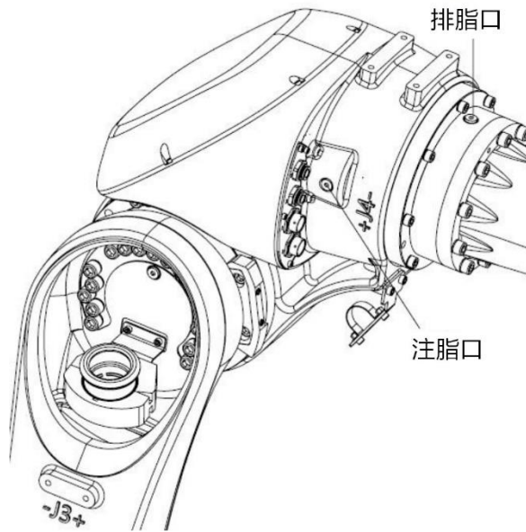
图 12-15 更换 J4 轴减速器润滑脂
