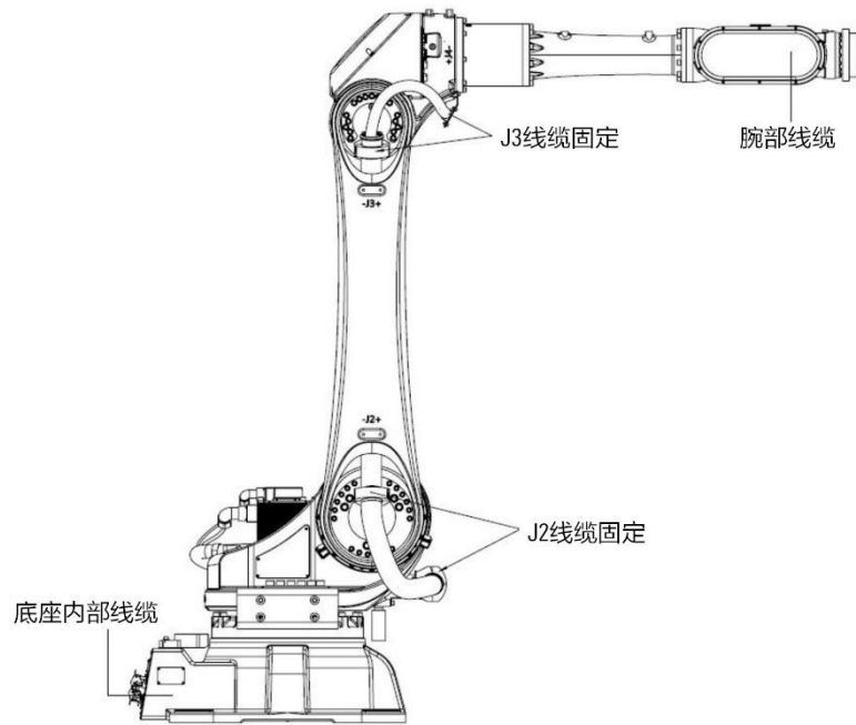
图 12-2 AIR50-2700/AIR80-2560 操作机线缆布局示意图
