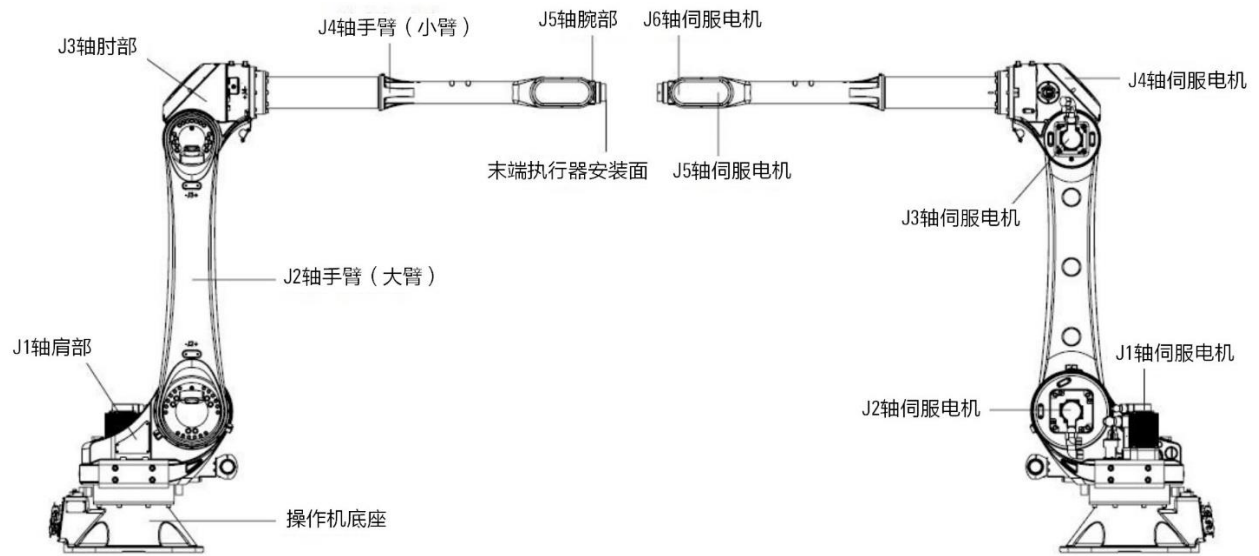
图 1-6 AIR20-3100 机器人本体及其各个部分
