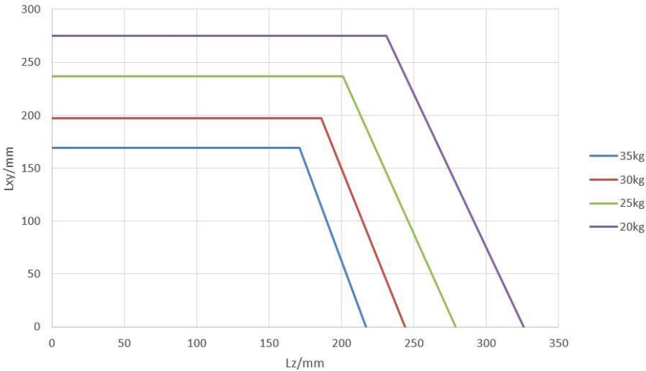
图 7-17 AIR35-2700 腕部负载质心位置示意图
