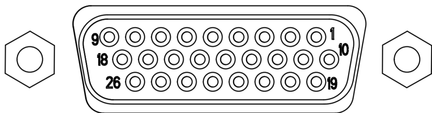
图 4-8 AIR6SC-500A 型操作机小臂 I/O 输出接口
