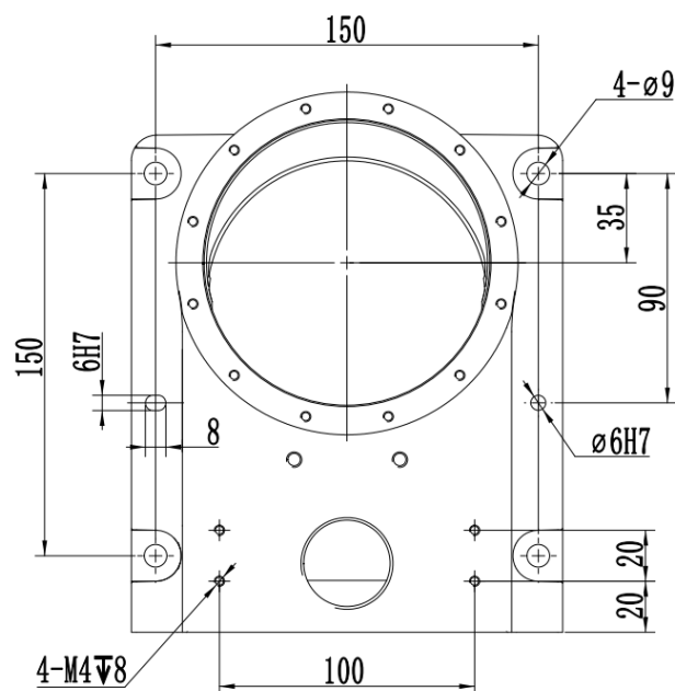
图 3-2 AIR6SC-500A 型操作机底座接口尺寸
