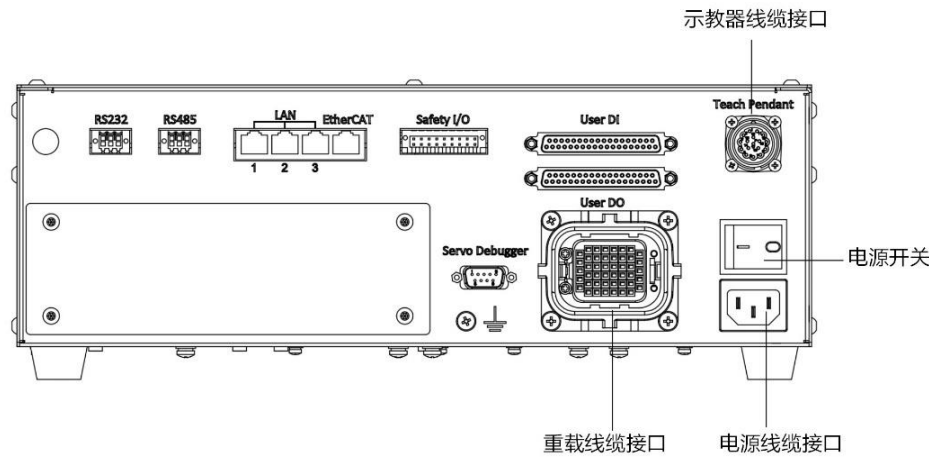
图 4-4 AIR6SC-500A 控制柜示意图
