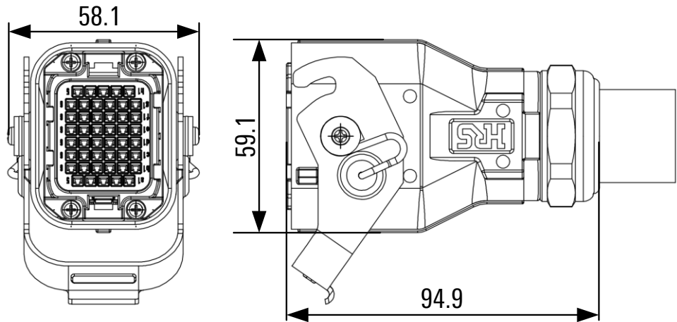
图 4-6 柜体侧重载插头尺寸
