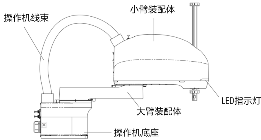
图 2-2 AIR6SC-500A 型机器人本体及其各个部分
