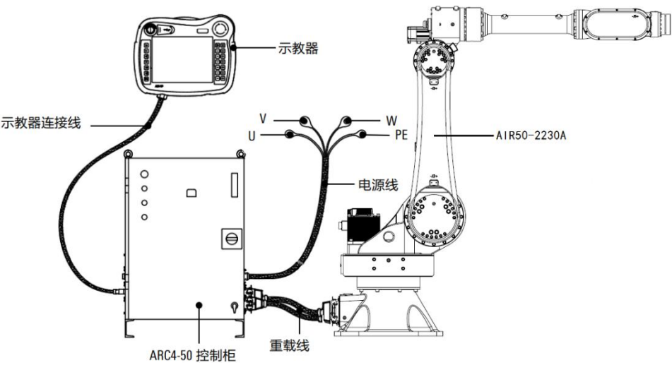
图 5-5 工业机器人系统接线概览
