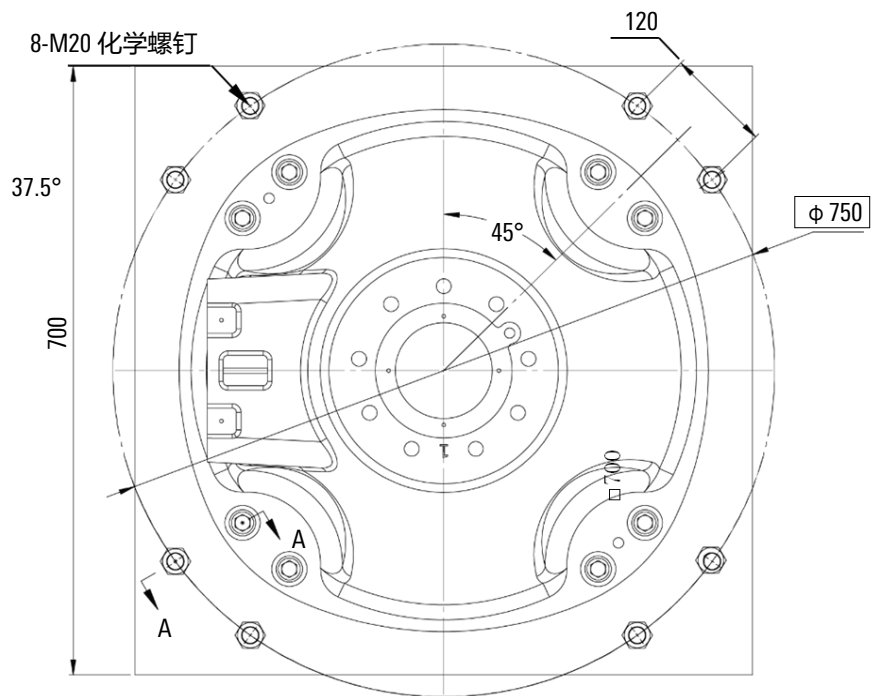
(a) 平面布置尺寸
