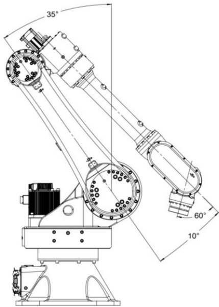
图 7-2 AIR50-2230A 操作机搬运位姿图
