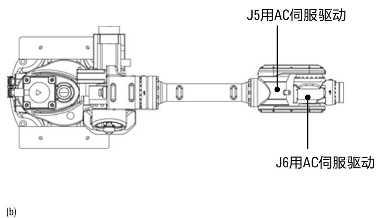
图 2-2 AIR50-2230A 机器人本体及其各个部分示意图
