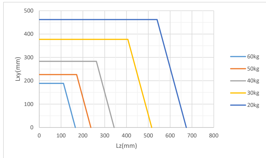
图 6-9 AIR50-2230A 腕部负载质心位置示意图
