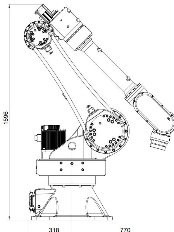
图 7-3 AIR50-2230A 搬运时操作机尺寸
