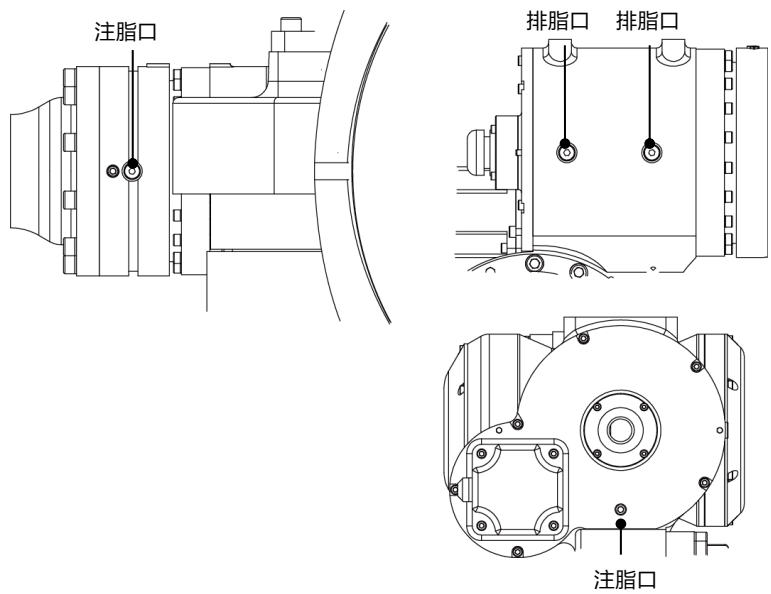
图 10-9 更换 J4 轴齿轮箱及减速器润滑脂
