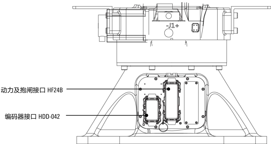
图 4-1 AIR50-2230A 操作机本体上重载连接器
