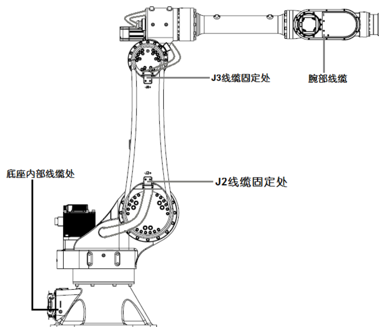
图 10-1 操作机线缆布局图
