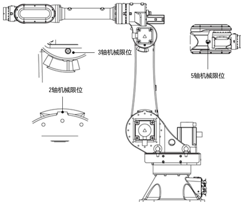
图 6-2 AIR50-2230A 操作机上机械式制动器
