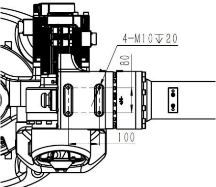
图 6-11 AIR50-2230A 肘部负载接口尺寸示意图
