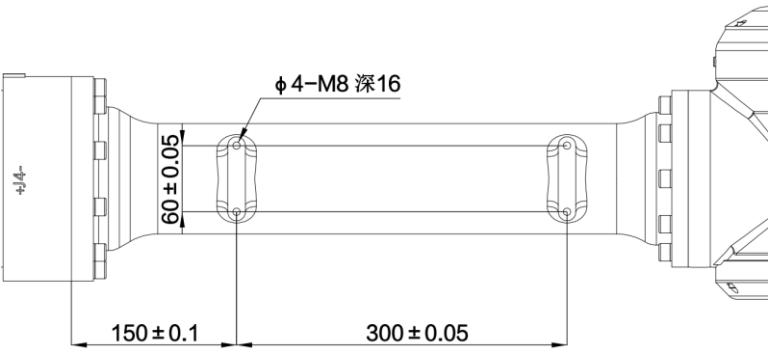
图 6-12 AIR50-2230A 小臂接口尺寸图
