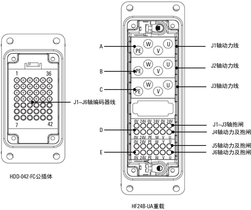
图 4-2 AIR50-2230A 操作机重载接口定义
