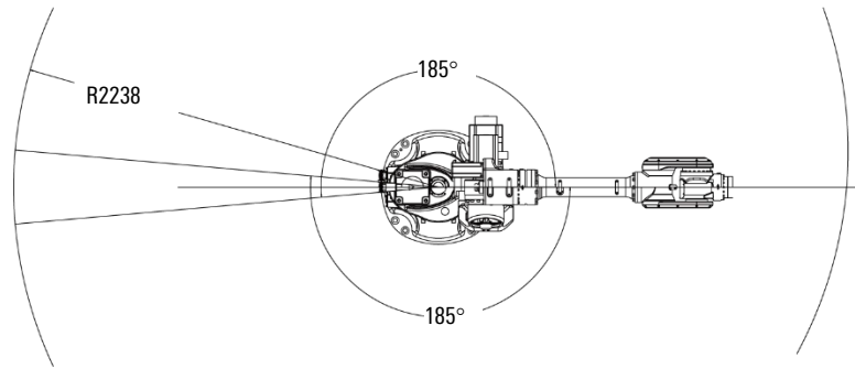
图 6-1 AIR50-2230A 操作机工作范围
