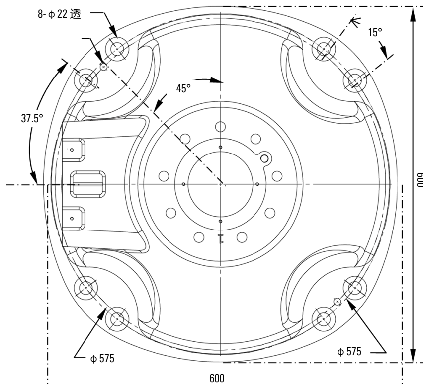
图 3-3 AIR50-2230A 操作机底座接口尺寸
