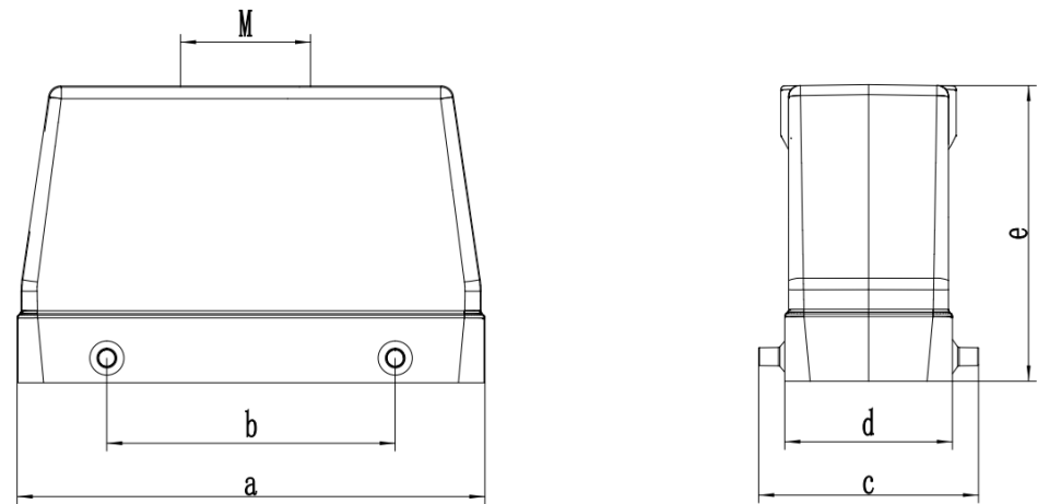
图 4-6 动力线重载接头尺寸
