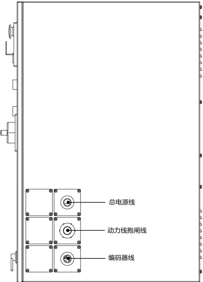
图 5-1 AIR50-2230A 控制柜线缆连接器定义
