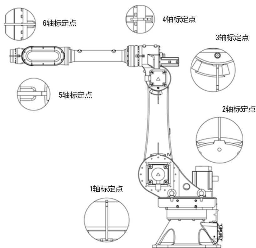
图 6-3 AIR50-2230A 各轴零点示意图
