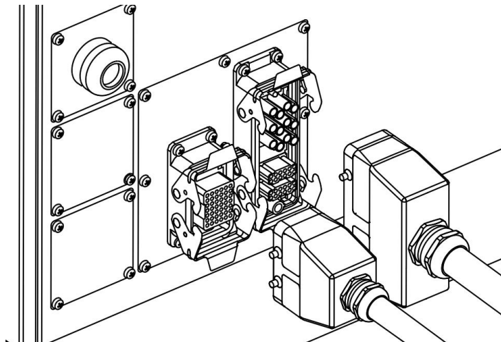
图 5-4 控制柜重载连接器接口
