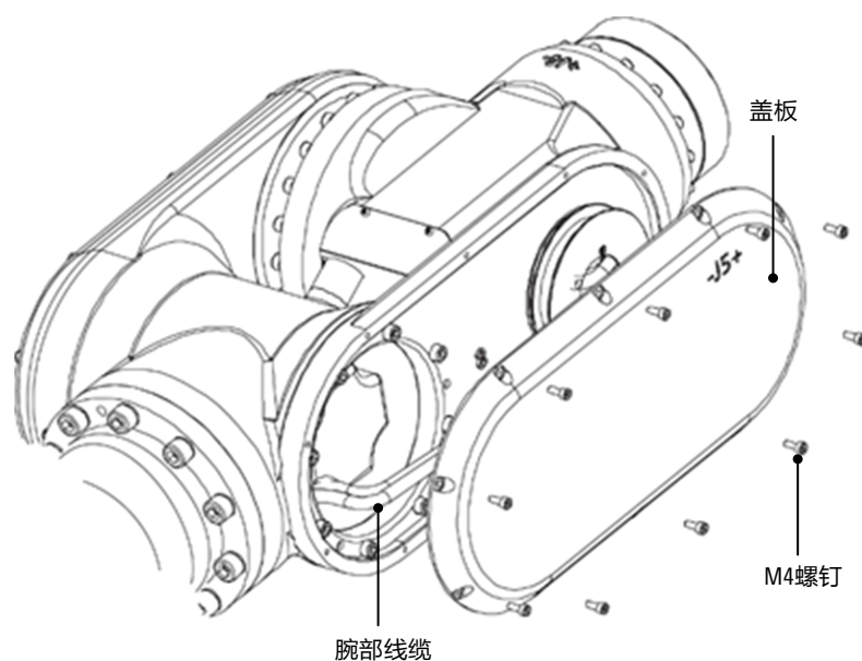
图 10-4 腕部内部线缆
