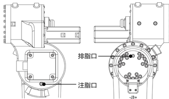
图 10-8 更换 J3 轴减速器润滑脂
