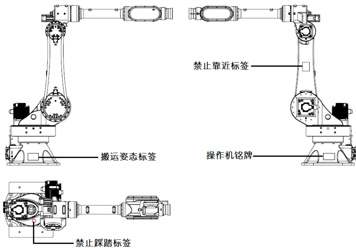
图 2-7 标签位置说明图
