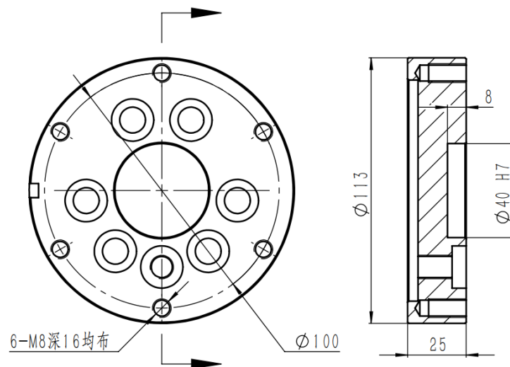
图 6-7 AIR50-2230A 腕部法兰尺寸示意图
