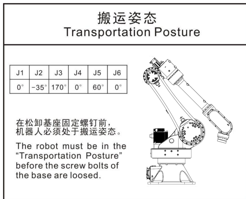
图 2-5 AIR50-2230A 本体各轴搬运姿态标签
