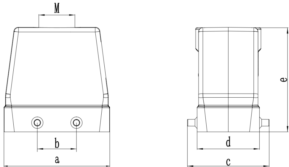
图 4-4 编码器线重载接头尺寸
