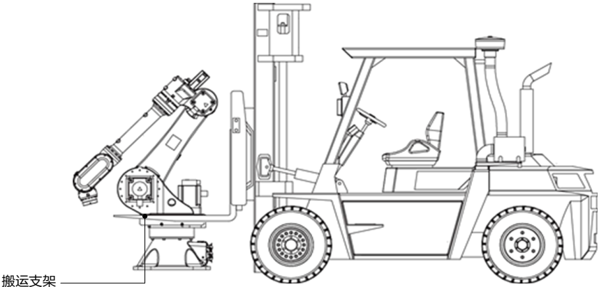
图 7-4 AIR50-2230A 叉车搬运示意图
