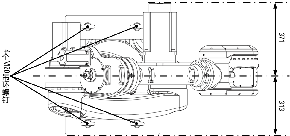
图 7-5 AIR50-2230A 吊环搬运示意图
