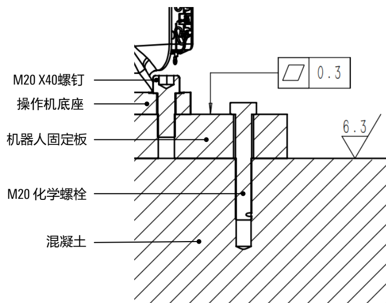
(b) 剖面图
