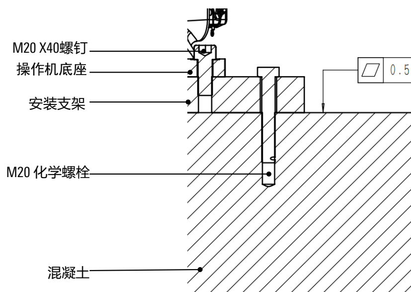
(b) 剖面图
