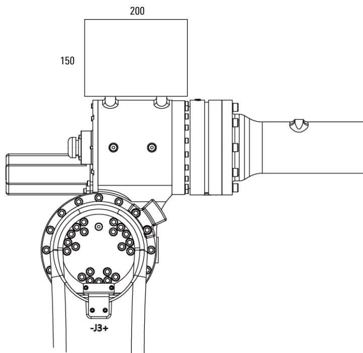
图 6-10 AIR50-2230A 肘部负载接口尺寸示意图
