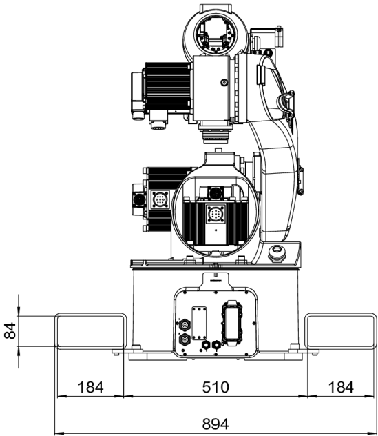
图 9-2 AIR20-2000C&AIR12-2000C-HI 系列搬运时操作机尺寸
