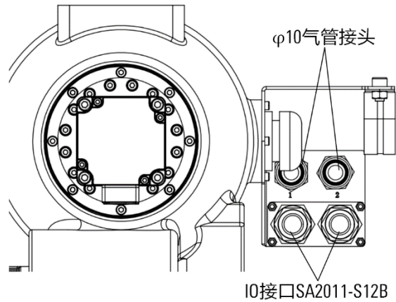
图 5-1 操作机小臂接口示意图
