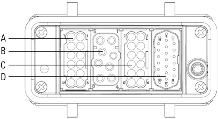
图 5-3 AIR20-2000C&AIR12-2000C-HI 操作机本体上适配 inCube22 重载连接器
