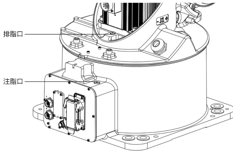
图 12-6 更换 J1 轴减速器润滑脂
