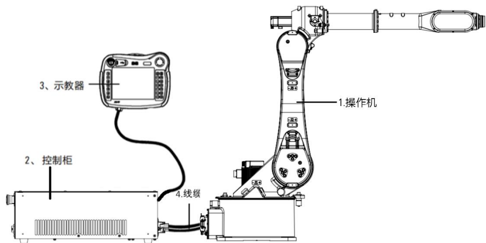
图 1-1 机器人系统构成-inCube22
