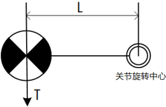
图 7-4 负载离心率示意图
