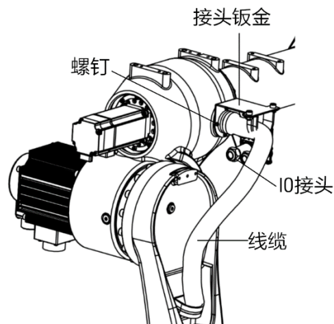
图 12-3 肘部内部线缆
