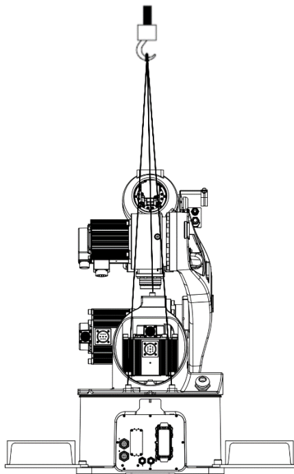
图 9-7 AIR20-2000C&AIR12-2000C-HI 系列吊环搬运示意图
