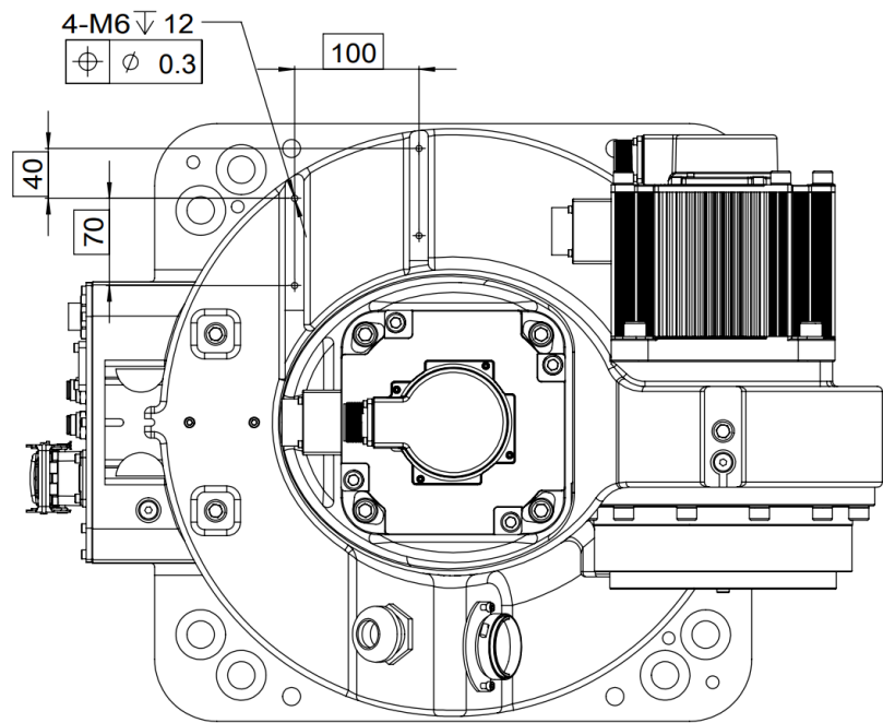
图 7-8 AIR20-2000C&AIR12-2000C-HI 系列肩部接口尺寸图
