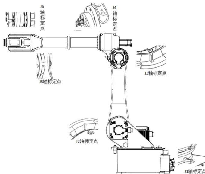
图 8-1 AIR20-2000C&AIR12-2000C-HI 系列各轴零点示意图
