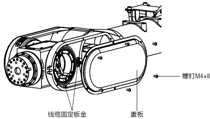
图 12-4 腕部内部线缆
