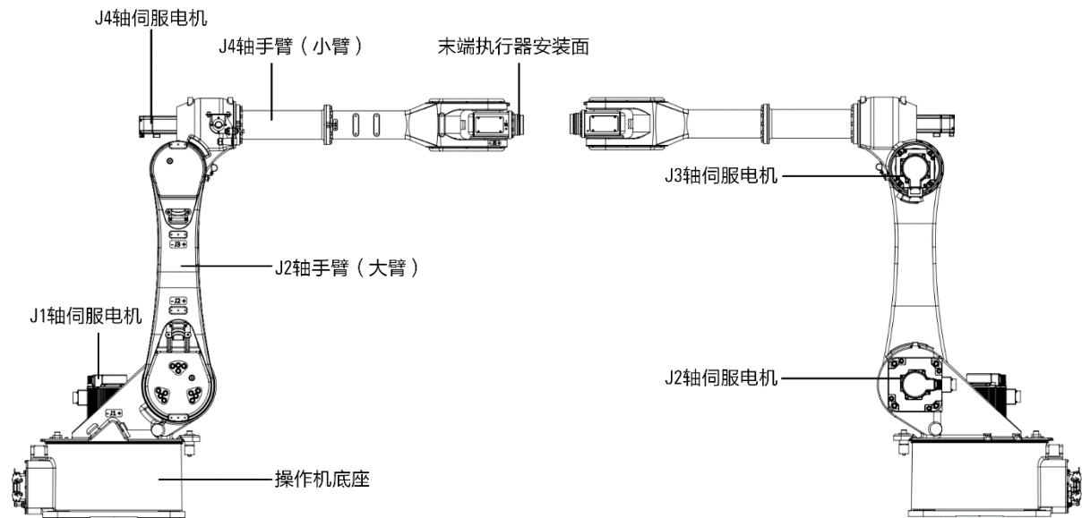
图 1-2 AIR20-2000C&AIR12-2000C-HI 系列机器人本体及其各个部分
