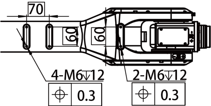
图 7-7 AIR20-2000C&AIR12-2000C-HI 系列小臂接口尺寸图
