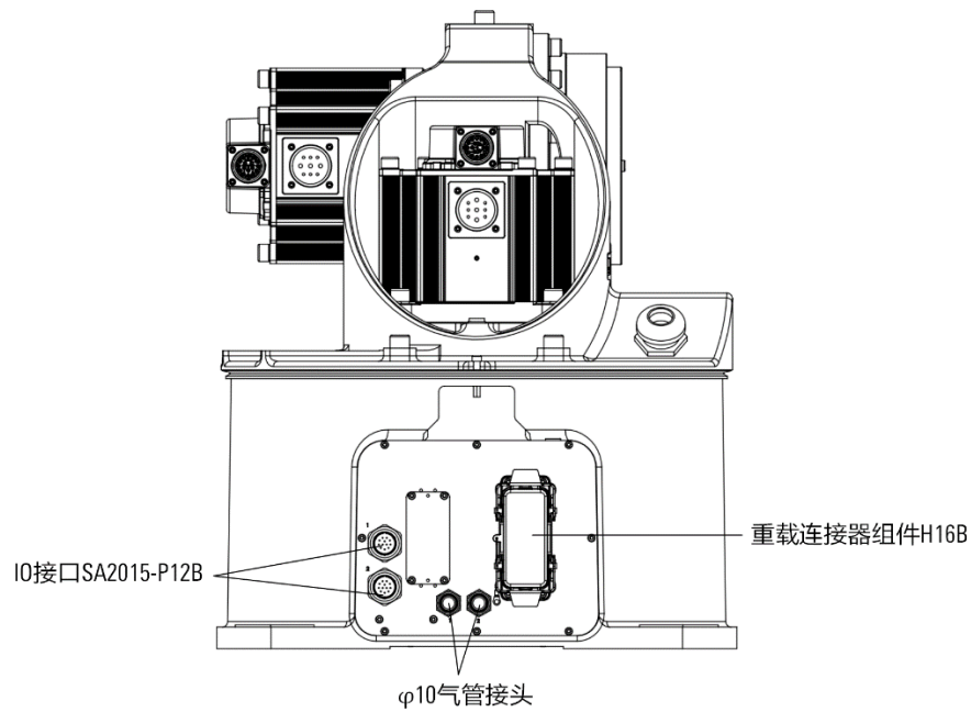
图 5-2 操作机底座接口示意图
