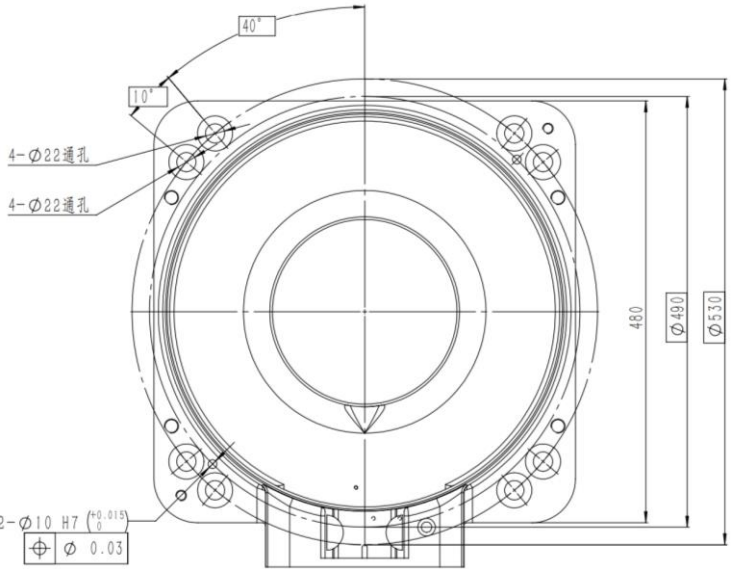
图 4-1 AIR20-2000C&AIR12-2000C-HI 系列操作机底座接口尺寸
