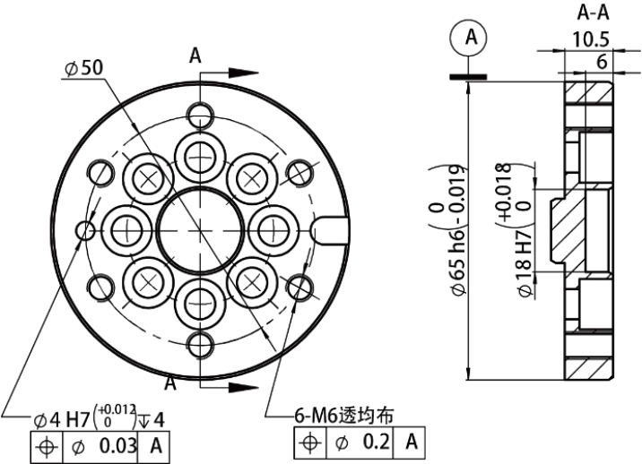
图 7-3 AIR20-2000C&AIR12-2000C-HI 系列腕部法兰尺寸示意图
