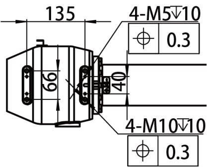
图 7-6 AIR20-2000C&AIR12-2000C-HI 系列肘部负载接口尺寸示意图
