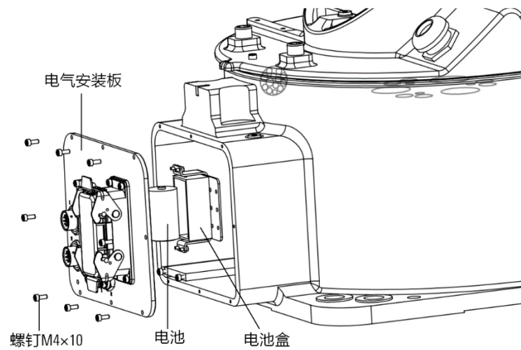
图 12-5 拆卸操作机电器安装面板
