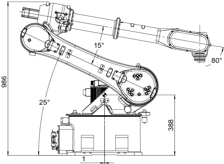
图 9-3 AIR20-2000C&AIR12-2000C-HI 系列搬运时操作机尺寸
