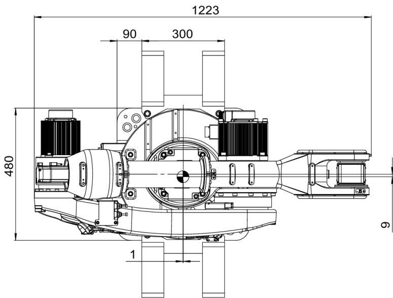
图 9-4 AIR20-2000C&AIR12-2000C-HI 系列搬运时操作机尺寸
