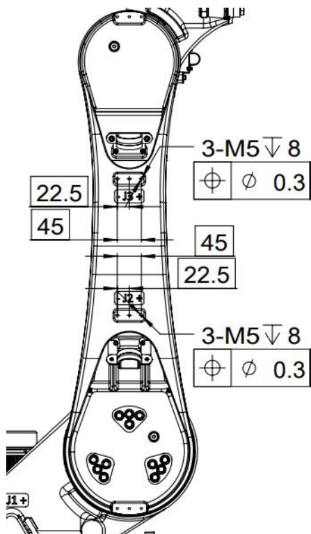
图 7-9 AIR20-2000C&AIR12-2000C-HI 系列大臂接口尺寸图
