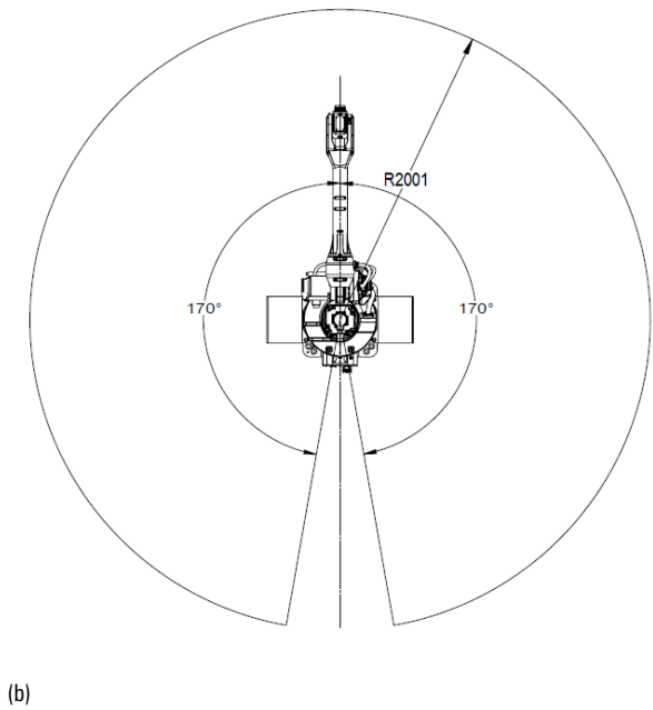
图 7-1 AIR20-2000C&AIR12-2000C-HI 系列操作机工作范围
