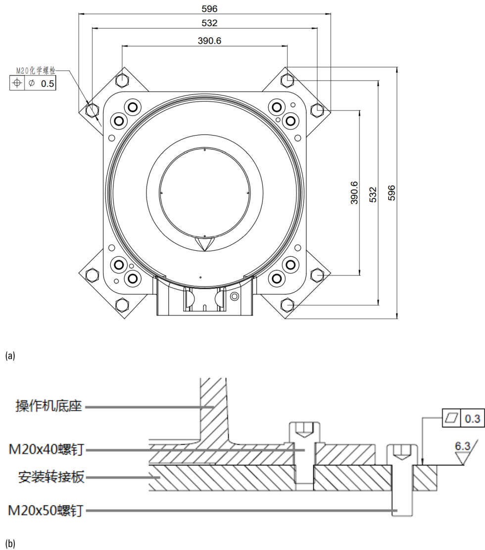
图 4-3 操作机支架固定示意图
