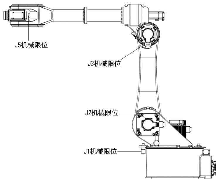
图 7-2 AIR20-2000C&AIR12-2000C-HI 系列操作机上机械式制动器
