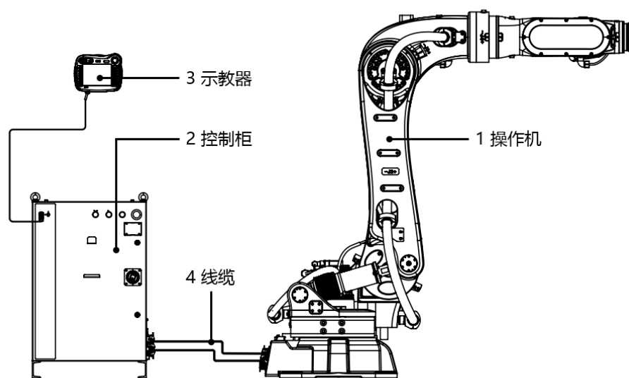
图 1-1 大负载机器人系统的构成
