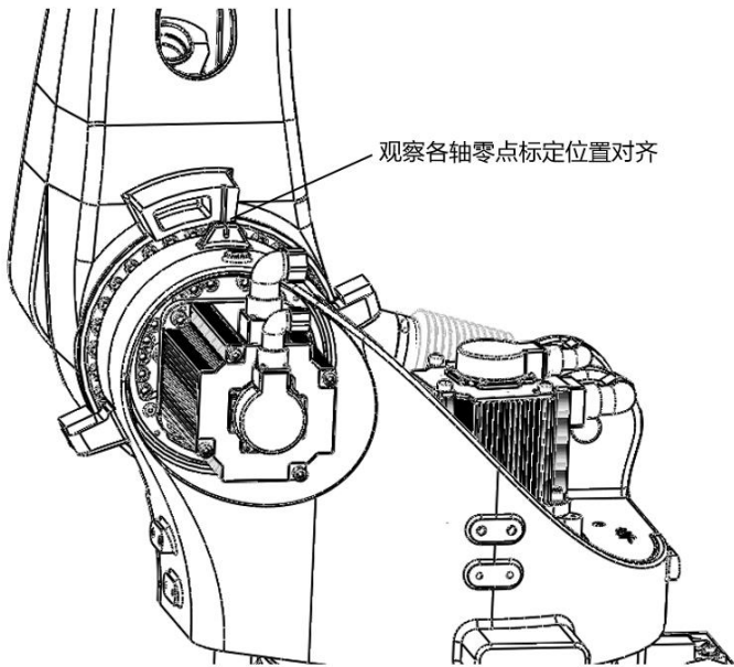
图 8-3 大负载肉眼观察零点标定方式
