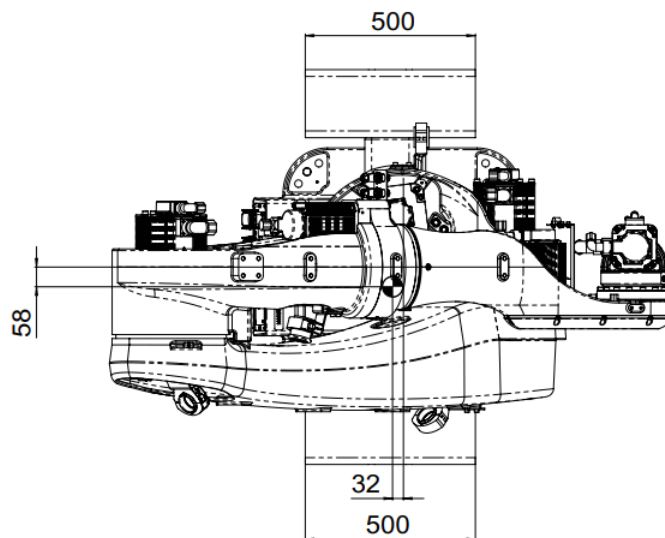
图 9-5 AIR220-3100/AIR130-3100/AIR170-3100 搬运时操作机尺寸
