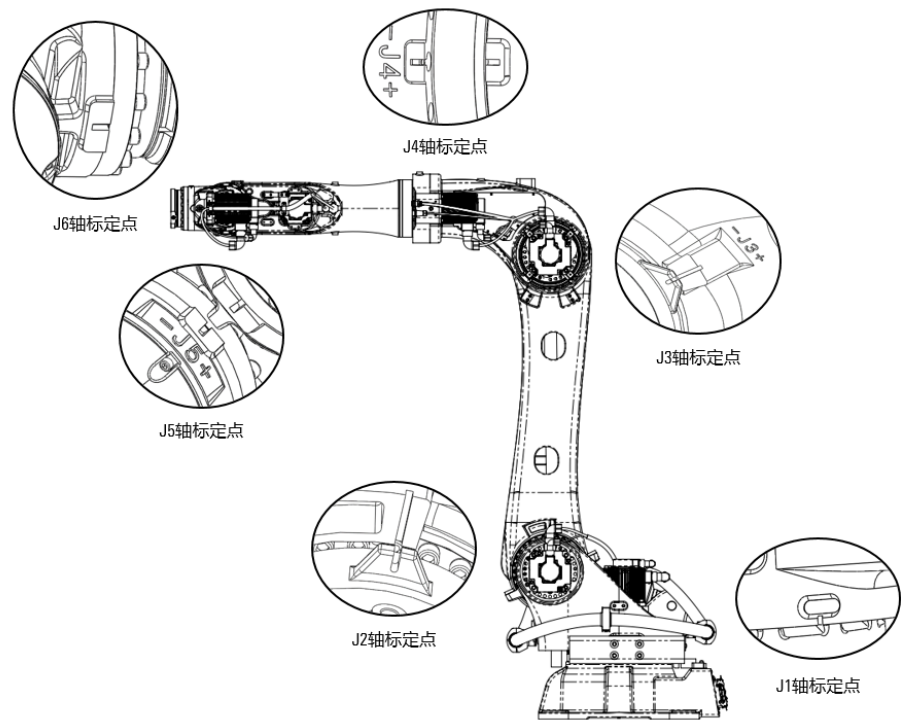
图 8-2 AIR220-3100/AIR130-3100/AIR170-3100 各轴零点示意图
