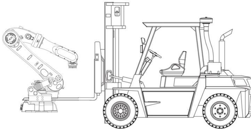
图 9-7 AIR220-3100/AIR130-3100/AIR170-3100 叉车搬运示意图
