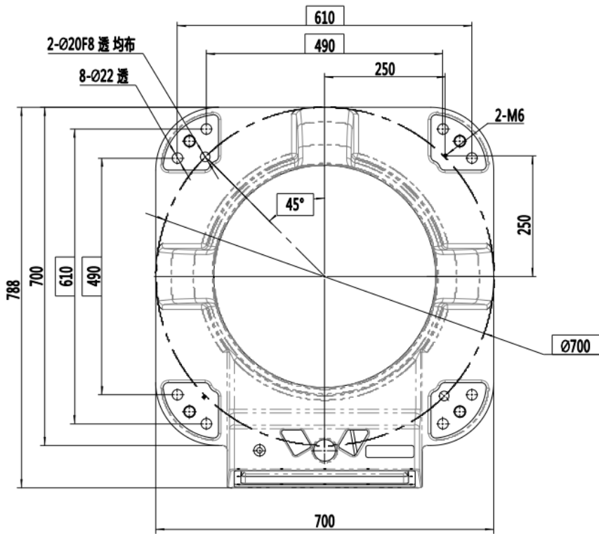
图 4-1 操作机基座接口尺寸
