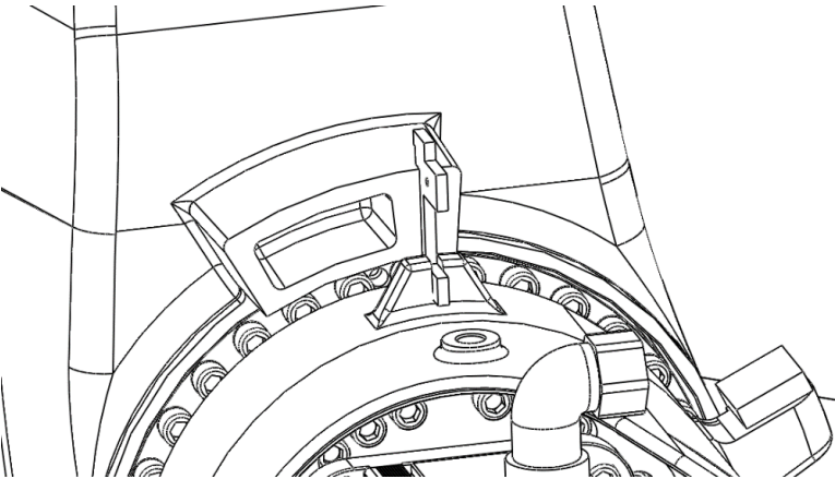
图 8-4 大负载零点标定块标定方式
