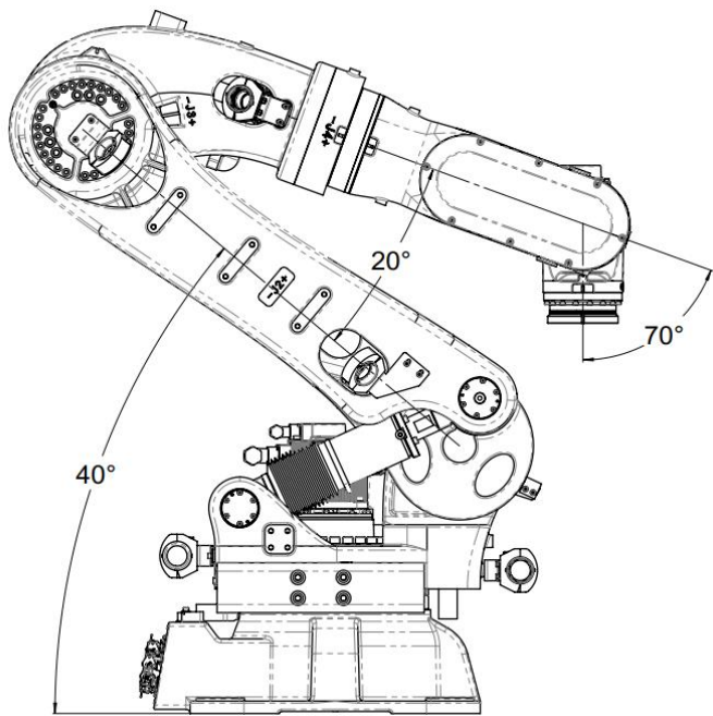
图 9-2 AIR280-2700/AIR130-2700/AIR170-2700/AIR220-2700 操作机搬运位姿图
