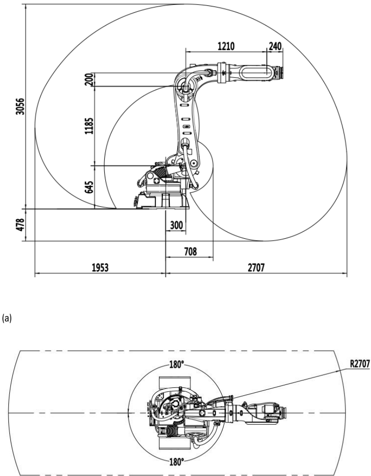
(b) 图 7-3 AIR280-2700/AIR130-2700/AIR170-2700/AIR220-2700 操作机工作范围
