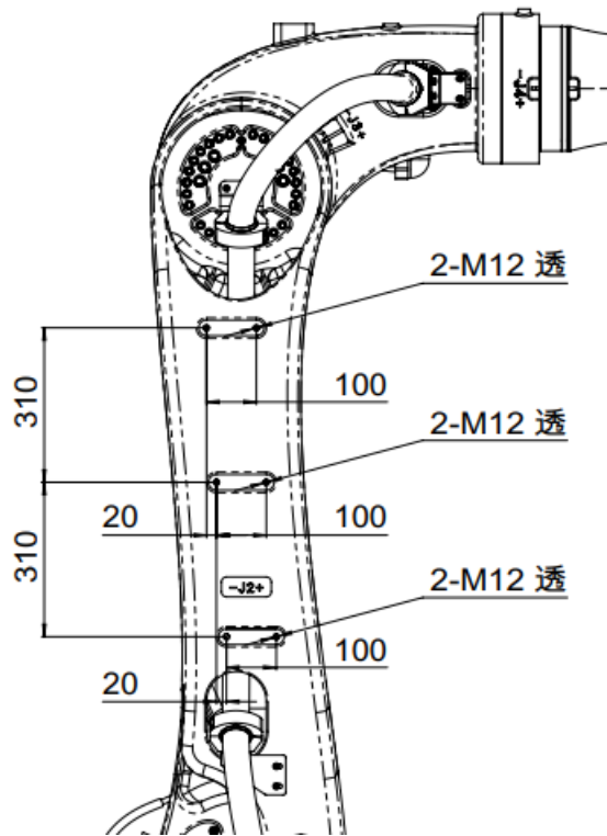
图 7-17 AIR220-3100/AIR130-3100/AIR170-3100 大臂接口尺寸图
