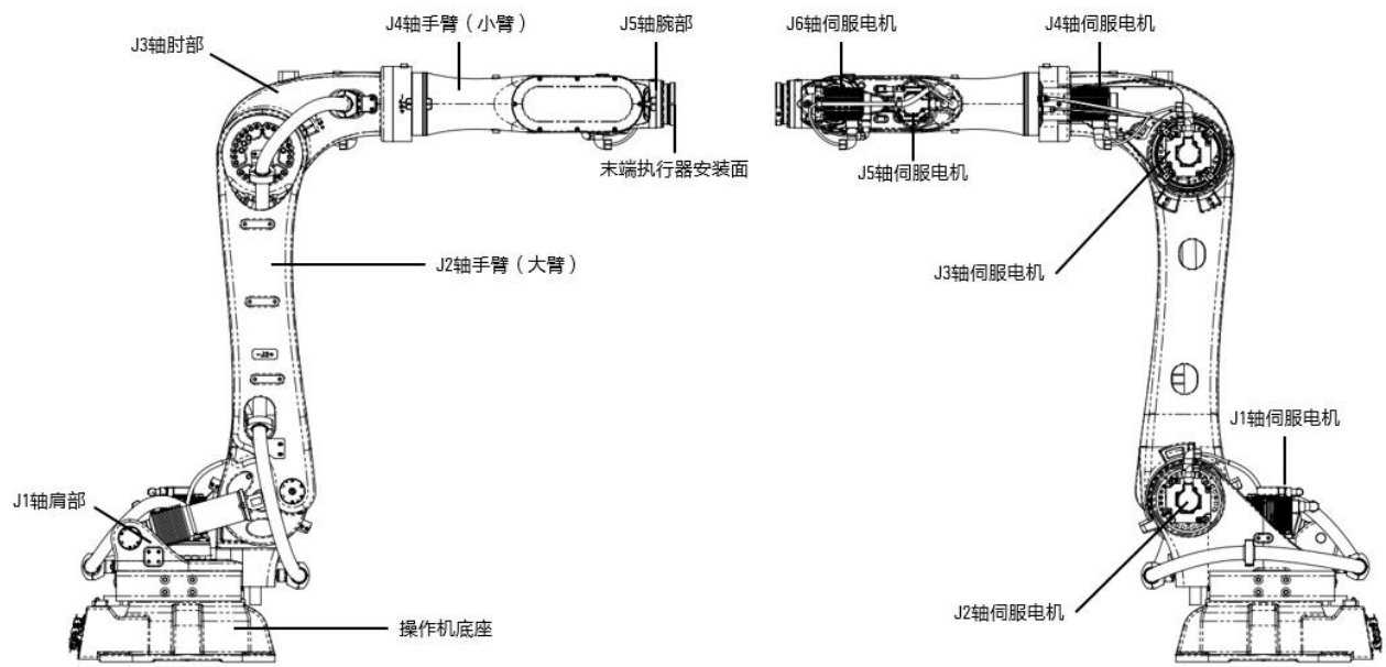
图 1-3 AIR220-3100/AIR130-3100/AIR170-3100 机器人本体及其各个部分
