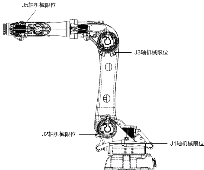
图 7-6 AIR220-3100/AIR130-3100/AIR170-3100 操作机机械式制动
