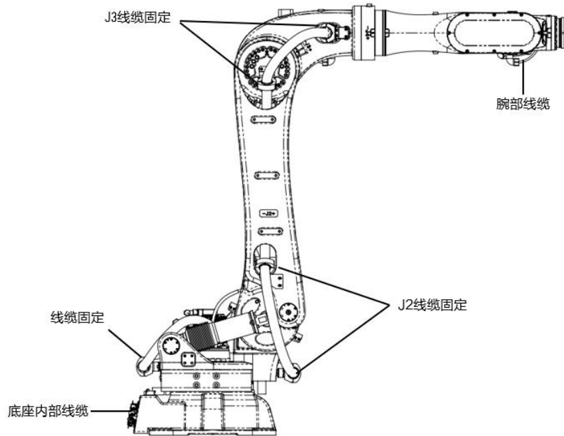
图 12-2 AIR220-3100/AIR130-3100/AIR170-3100 操作机线缆布局图
