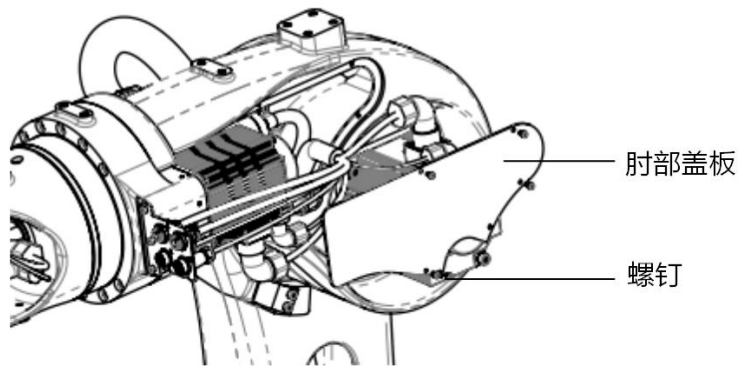
图 12-4 肘部内部线缆
