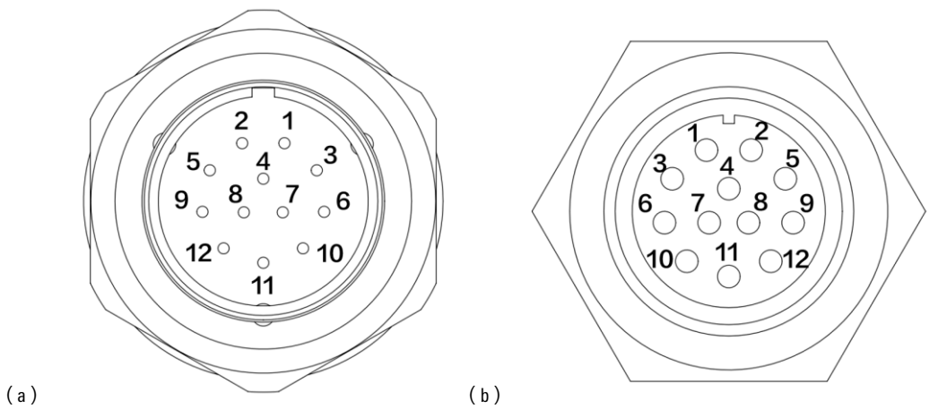
图 5-5 大负载操作机底座 IO 航插接口（左）及小臂 IO 航插接口（右）
