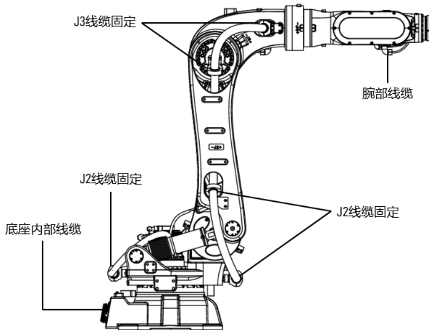
图 12-1 AIR280-2700/AIR130-2700/AIR170-2700/AIR220-2700 操作机线缆布局图
