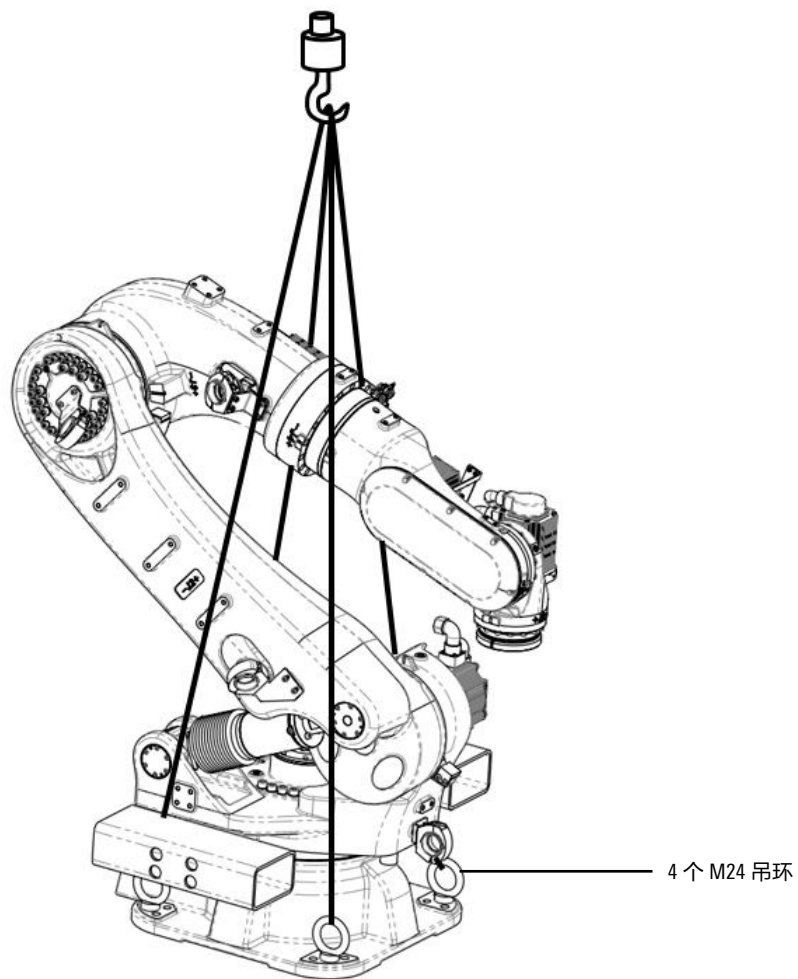
图 9-8 AIR280-2700/AIR130-2700/AIR170-2700/AIR220-2700 吊环搬运示意图
