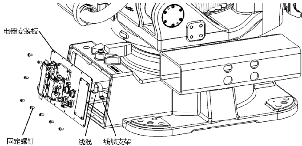
图 12-3 底座内部线缆
