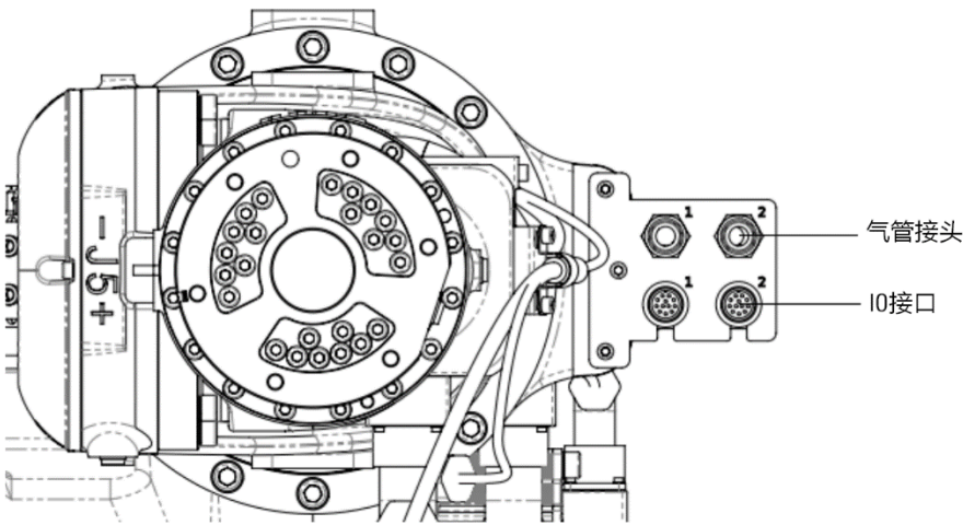
图 5-2 大负载操作机小臂上的电气接口
