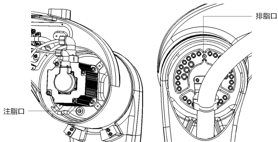
图 12-10 更换 J3 轴减速器润滑脂
