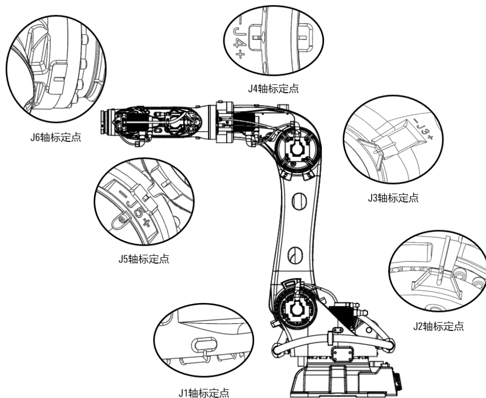
图 8-1 AIR280-2700/AIR130-2700/AIR170-2700/AIR220-2700 各轴零点示意图
