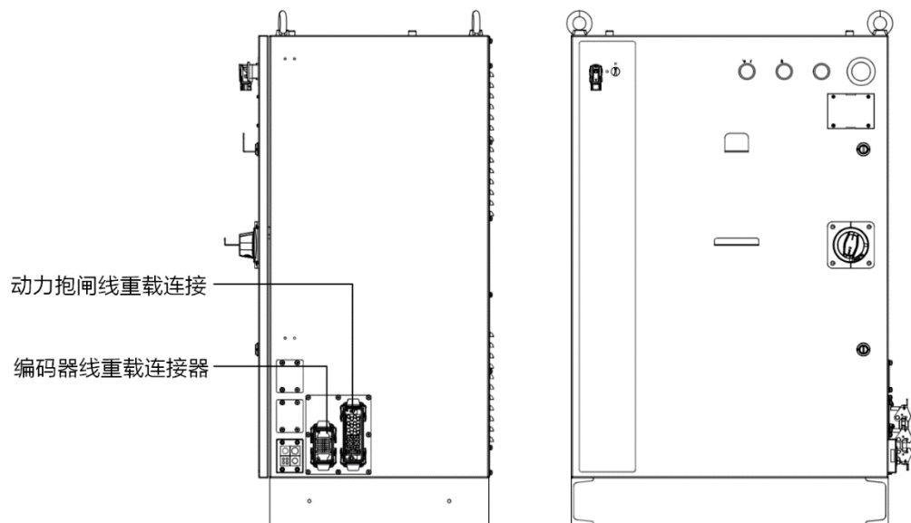
图 6-4 控制柜线缆连接器定义
