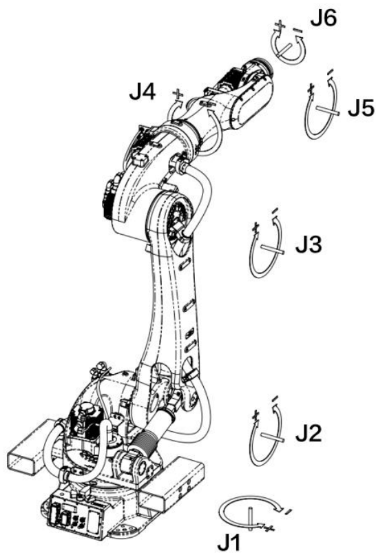
图 7-2 AIR220-3100/AIR130-3100/AIR170-3100 操作机各轴运动方向
