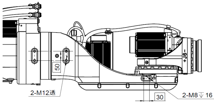
图 7-14 AIR280-2700/AIR130-2700/AIR170-2700/AIR220-2700 操作机小臂接口尺寸图
