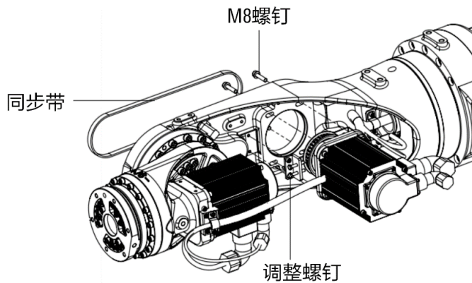
图 12-14 拆卸盖板
