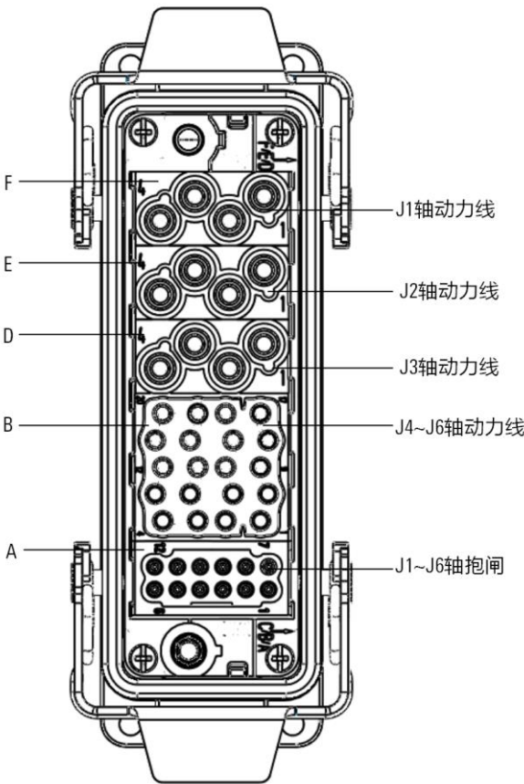
图 5-3 大负载操作机动力线重载连接器
