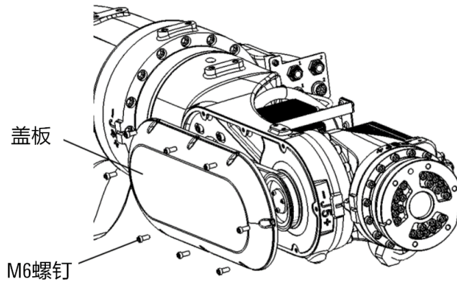
图 12-14 拆卸盖板
