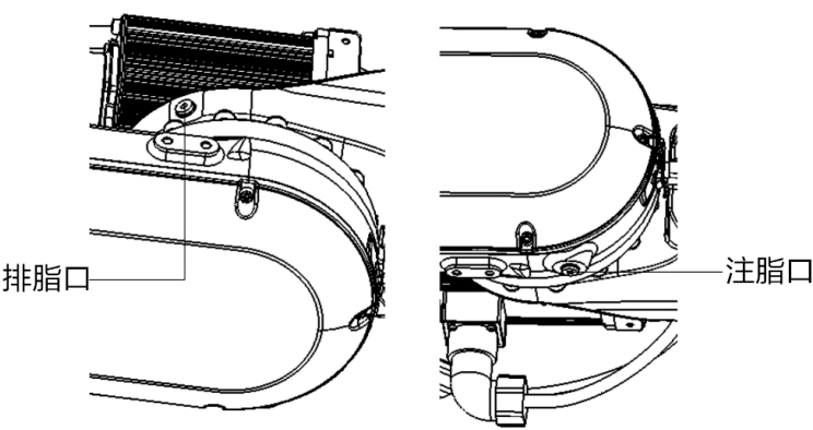
图 12-12 更换 J5 轴减速器润滑脂
