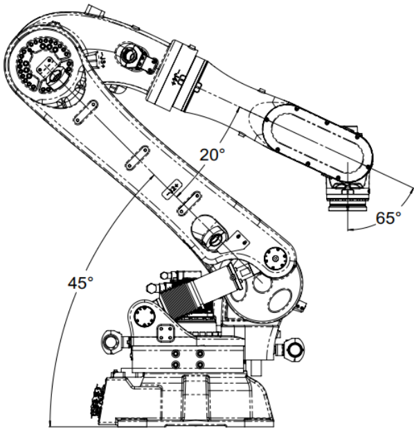
图 9-3 AIR220-3100/AIR130-3100/AIR170-3100 操作机搬运位姿图
