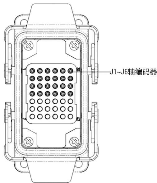
图 5-4 大负载操作机编码器线重载连接器
