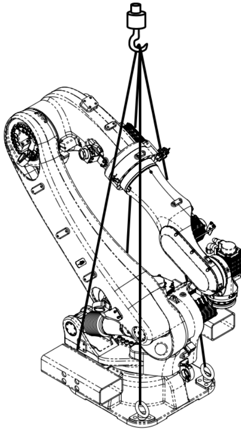
图 9-9 AIR220-3100/AIR130-3100/AIR170-3100 吊环搬运示意图
