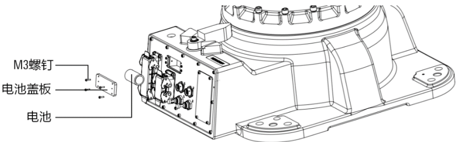
图 12-7 更换电池
