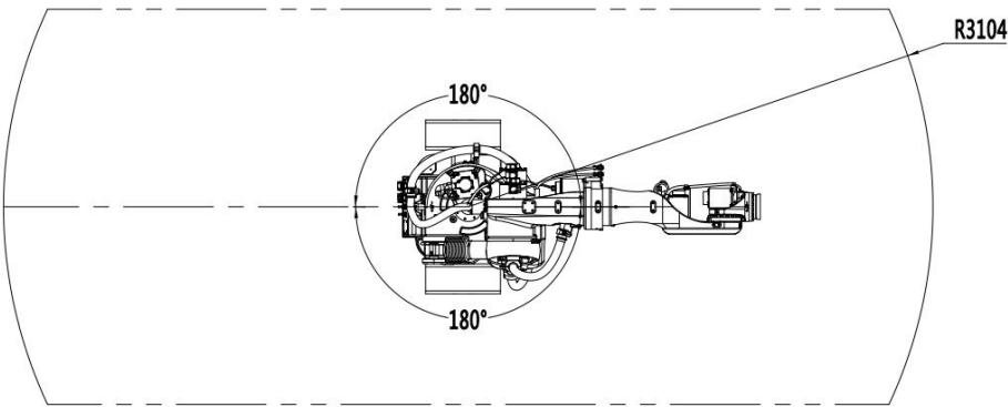
(b) 图 7-4 AIR220-3100/AIR130-3100/AIR170-3100 操作机工作范围
