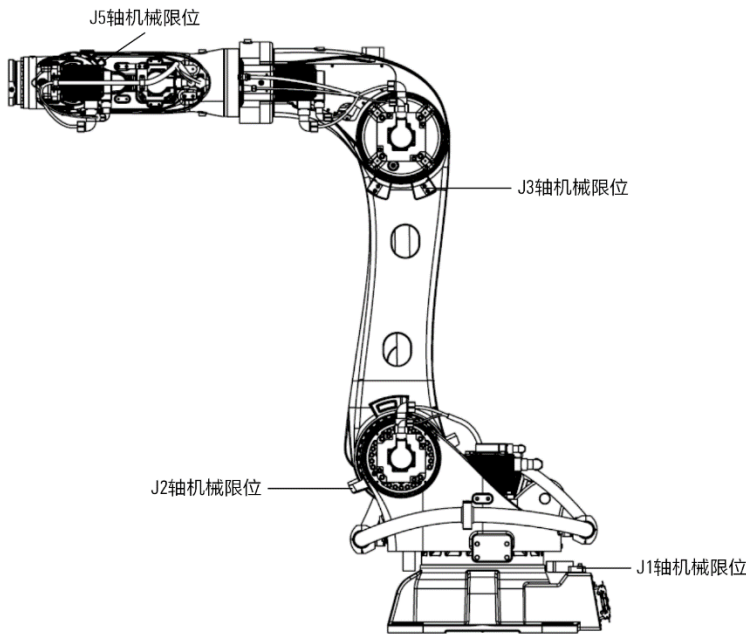
图 7-5 AIR280-2700/AIR130-2700/AIR170-2700/AIR220-2700 操作机机械式制动器
