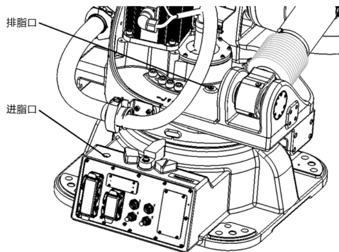
图 12-8 更换 J1 轴减速器润滑脂
