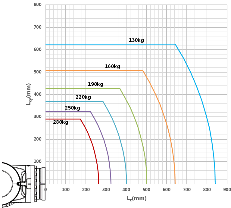
(b) 图 7-9 操作机腕部负载质心位置示意图
