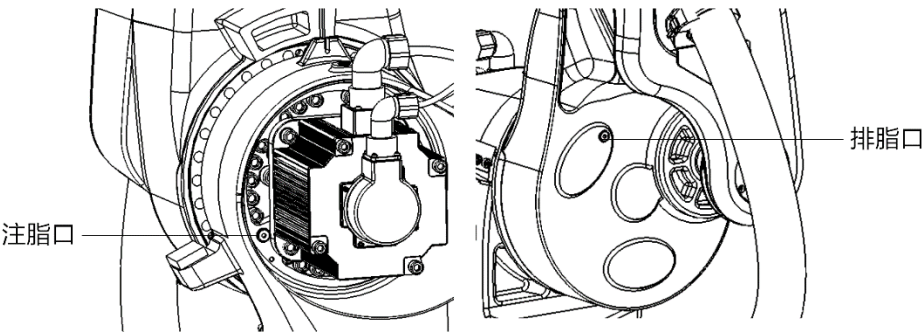
图 12-9 更换 J2 轴减速器润滑脂
