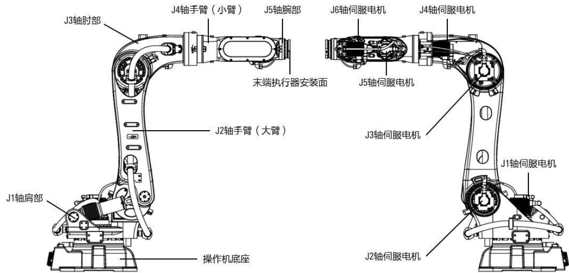
图 1-2 AIR280-2700/AIR130-2700/AIR170-2700/AIR220-2700 机器人本体及其各个部分
