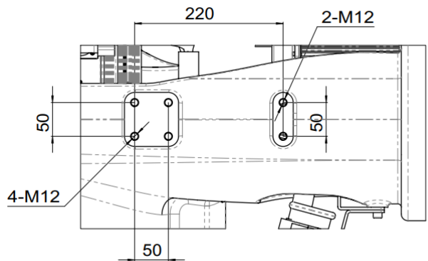
图 7-13 操作机肘部负载接口尺寸示意图
