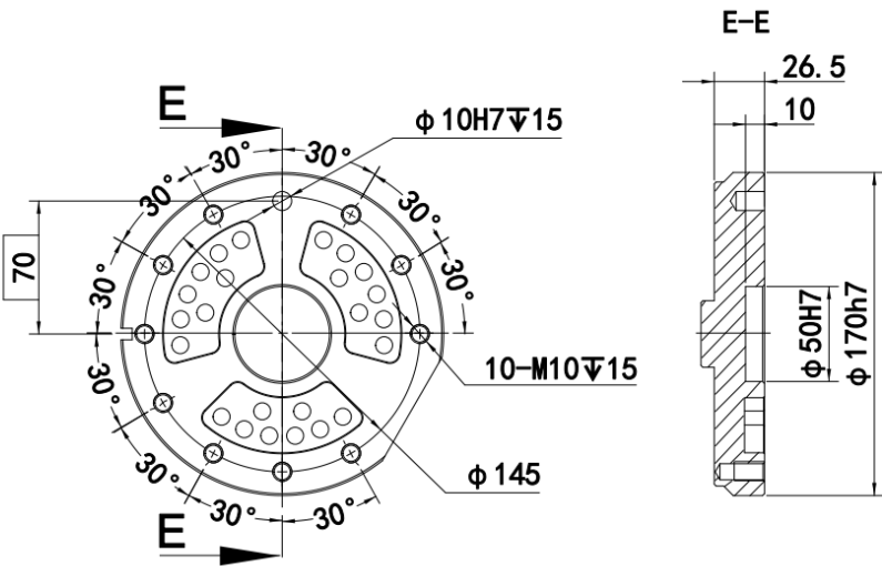
图 7-7 大负载操作机腕部法兰尺寸示意图
