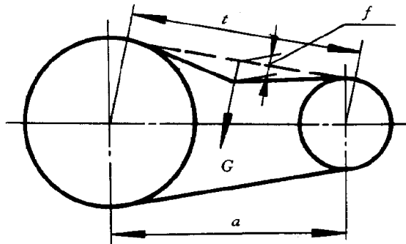
图 12-16 同步带安装挠度
