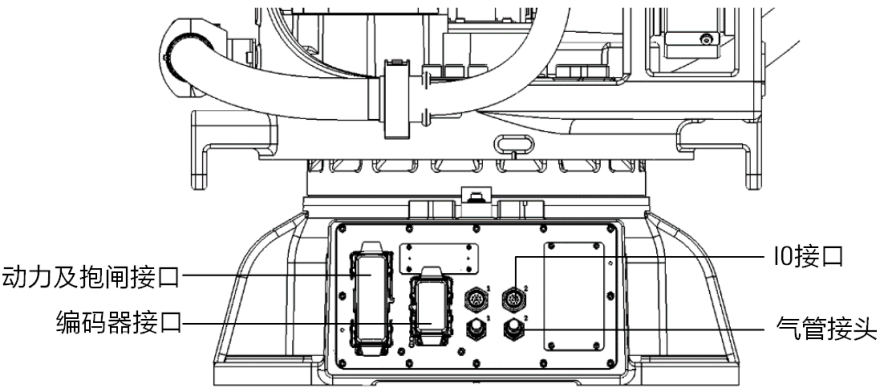
图 5-1 大负载操作机底座上电气接口
