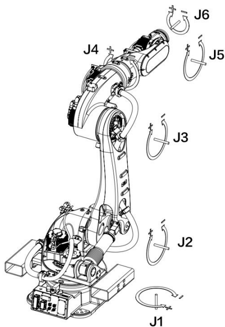
图 7-1 AIR280-2700/AIR130-2700/AIR170-2700/AIR220-2700 操作机各轴运动方向
