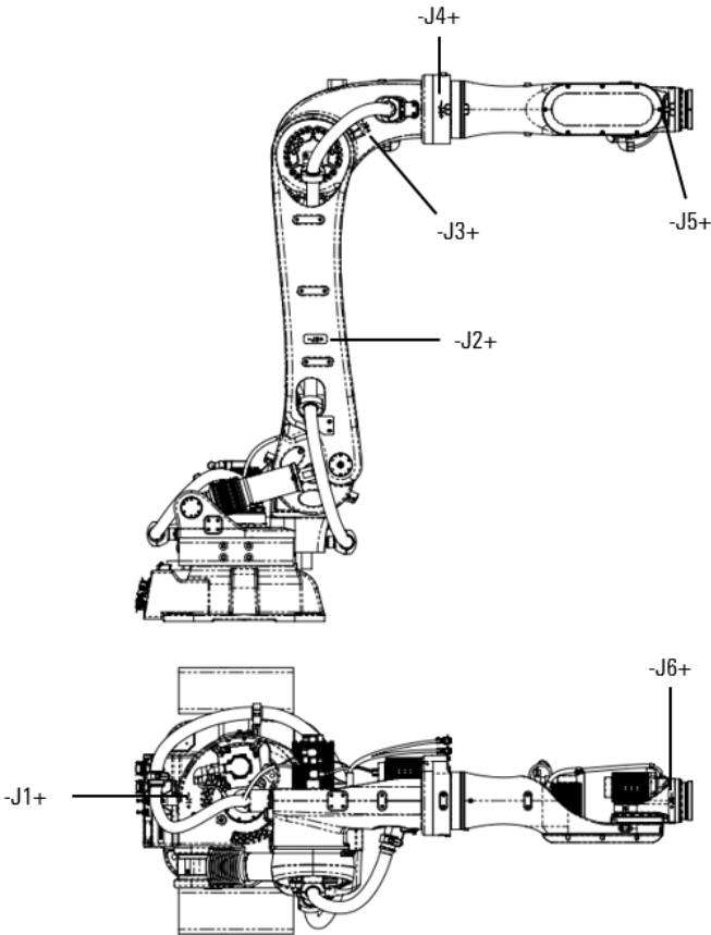
图 2-5 AIR220-3100/AIR130-3100/AIR170-3100 操作机上各轴方向标识
