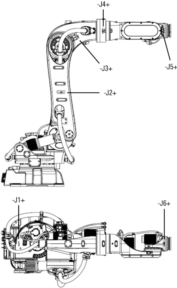
图 2-4 AIR280-2700/AIR130-2700/AIR170-2700/AIR220-2700 操作机上各轴方向标识
