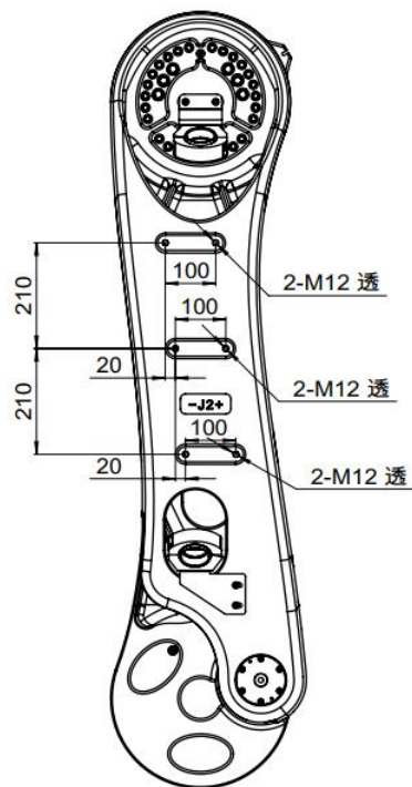
图 7-16 AIR280-2700/AIR130-2700/AIR170-2700/AIR220-2700 大臂接口尺寸图
