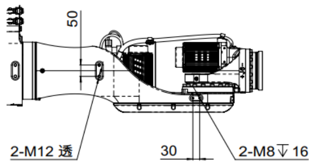
图 7-15 AIR220-3100/AIR130-3100/AIR170-3100 操作机小臂接口尺寸图
